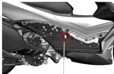
Cubierta secundaria al vaso de expansión
