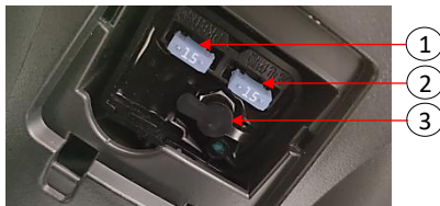
Accesorios del soporte del puerto de carga
