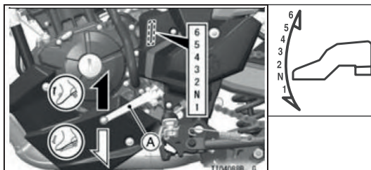
A: Pedal de cambios
