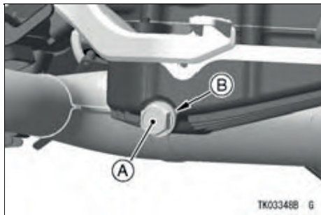
A. Perno de drenaje de aceite del motor B. Junta
