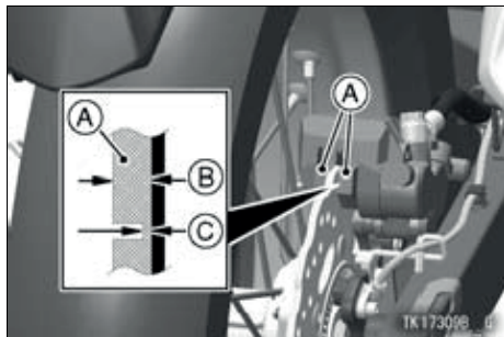
A: Pastillas del freno trasero B: Espesor del forro C: 1,5 mm
