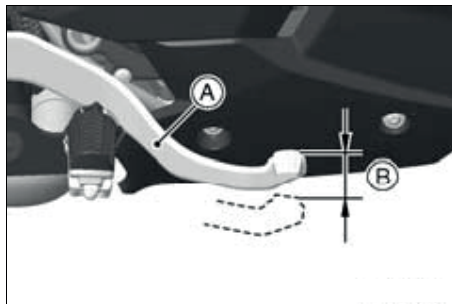
A: Pedal de freno B: 10 mm
