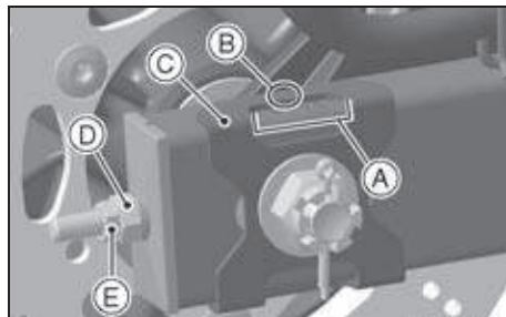
A. Marcas B. Muescas C. Indicador D. Tuerca de ajuste E. Contratuerca
