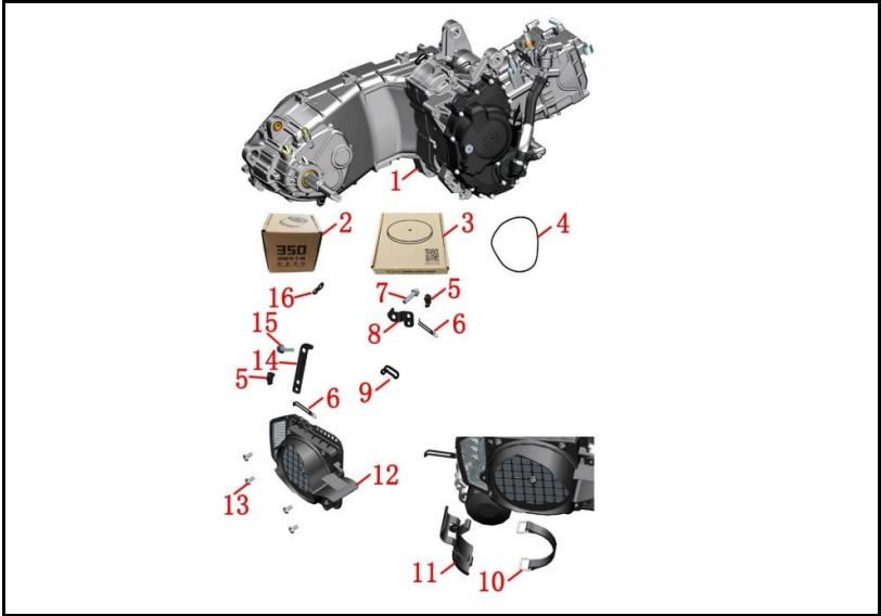
FIGURA N° 82: FILTRO MOTOR
