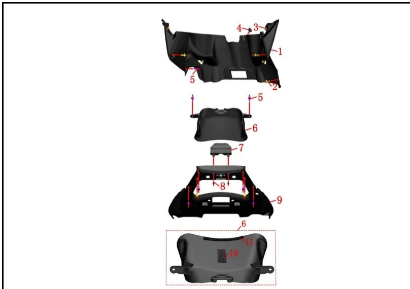
FIGURA N° 45: CUBIERTA
