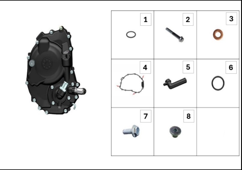
FIGURA N° 29: COMPONENTES TAPA CARCASA DERECHA
