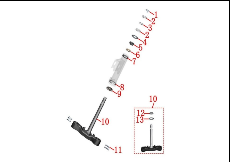
FIGURA N° 64: ESPIGA CENTRAL
