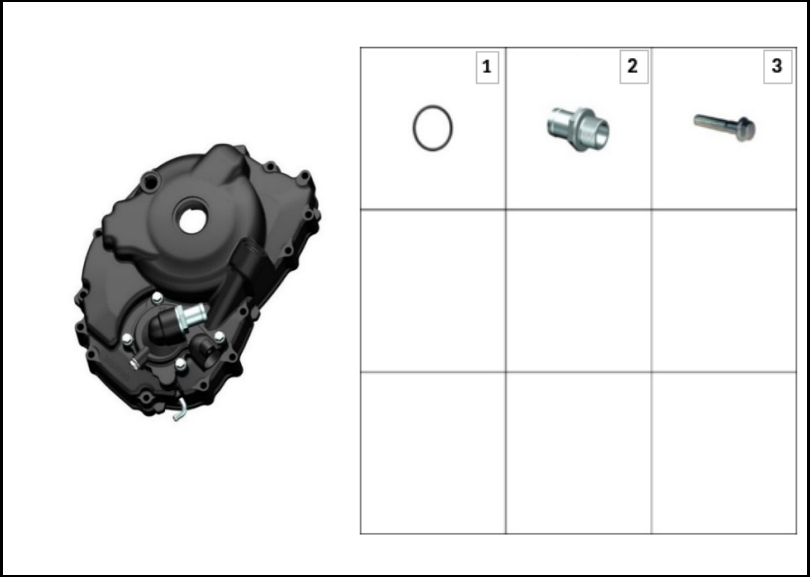
FIGURA N° 33: COMPONENTES TAPA CARCASA DERECHA
