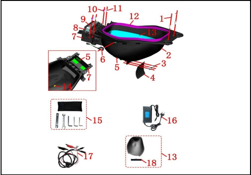
FIGURA N° 57: CAJA GUANTERA
