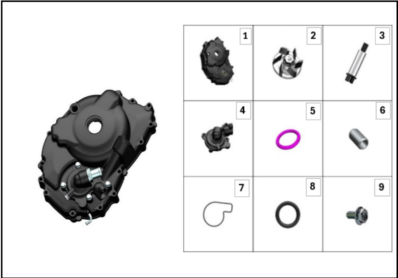
FIGURA N° 32: BOMBA AGUA
