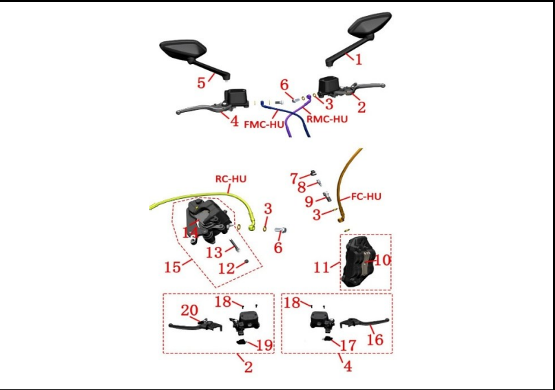
FIGURA N° 63: BOMBA FRENO TRASERA / DELANTERA
