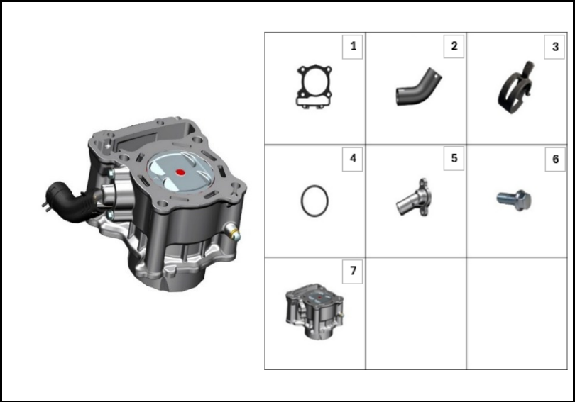
FIGURA N°8: CILINDRO
