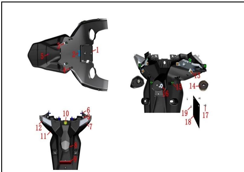
FIGURA N° 58: GUARDABARRO TRASERO
