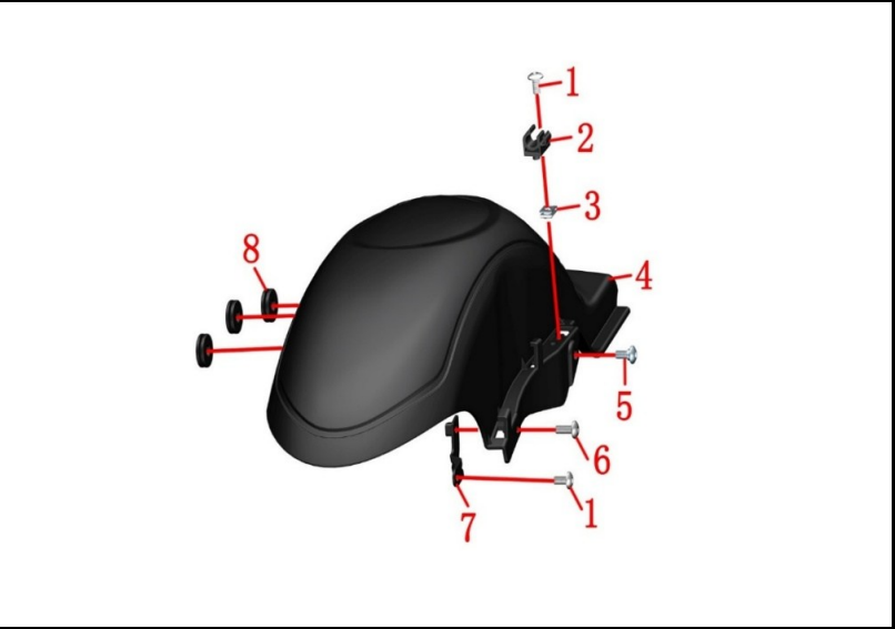
FIGURA N° 67: GUARDABARRO INTERNO
