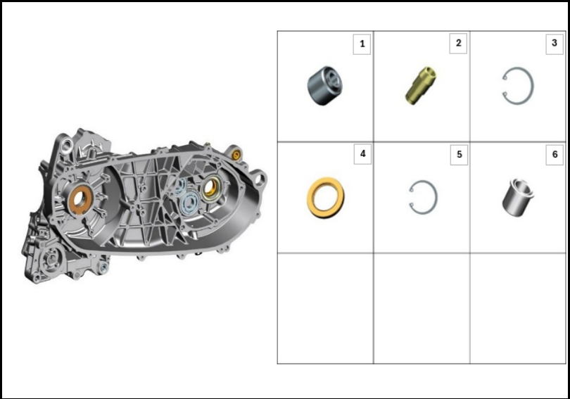
FIGURA N° 18: COMPONENTES CARCASA MOTOR IZQUIERDA
