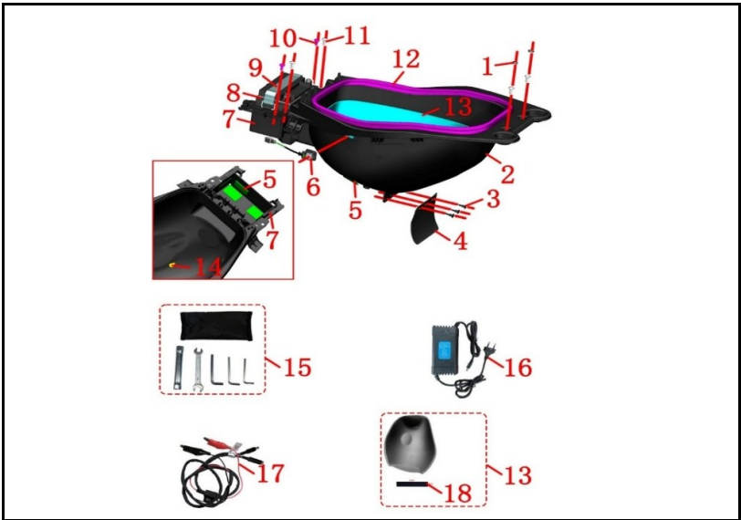
FIGURA N° 57: CAJA GUANTERA
