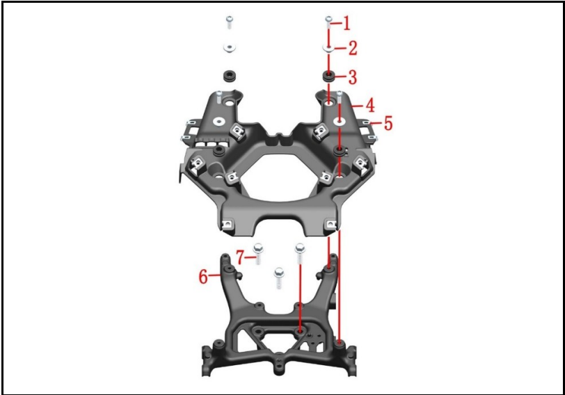
FIGURA N° 41: SOPORTE FAROLA
