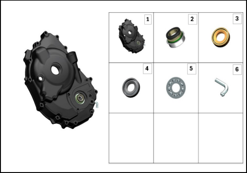
FIGURA N° 34: TAPA CARCASA DERECHA
