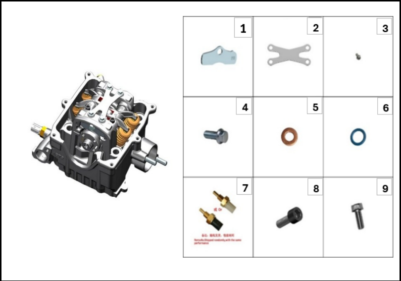
FIGURA N°4: SENSOR TEMPERATURA
