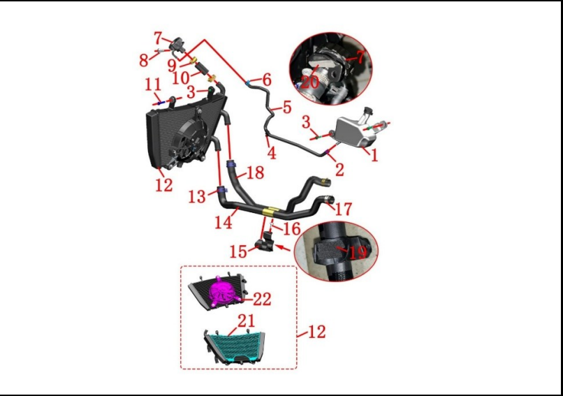
FIGURA N° 88: RADIADOR
