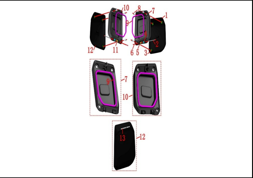
FIGURA N° 50: TAPA CAJA GUANTERA FRONTAL
