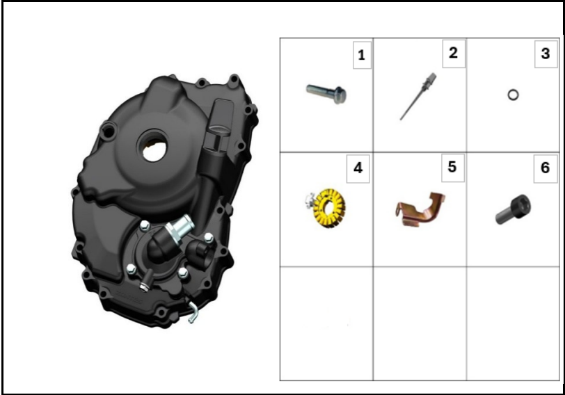
FIGURA N° 31: PLATO BOBINAS
