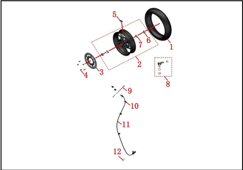
FIGURA N° 66: LLANTA DELANTERA
