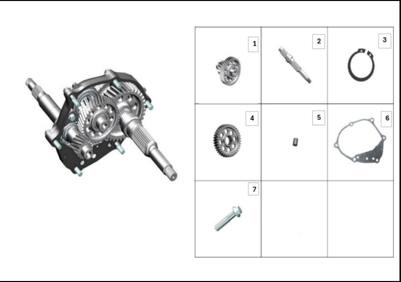
FIGURA N° 23: COMPONENTES CAUBIERTA TRANSMISION
