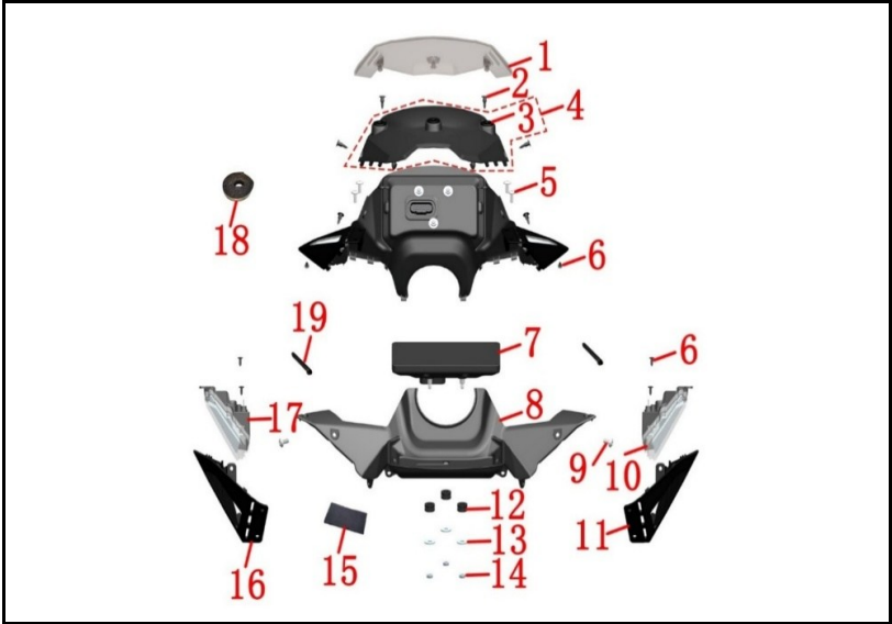
FIGURA N° 40: VELOCIMETRO
