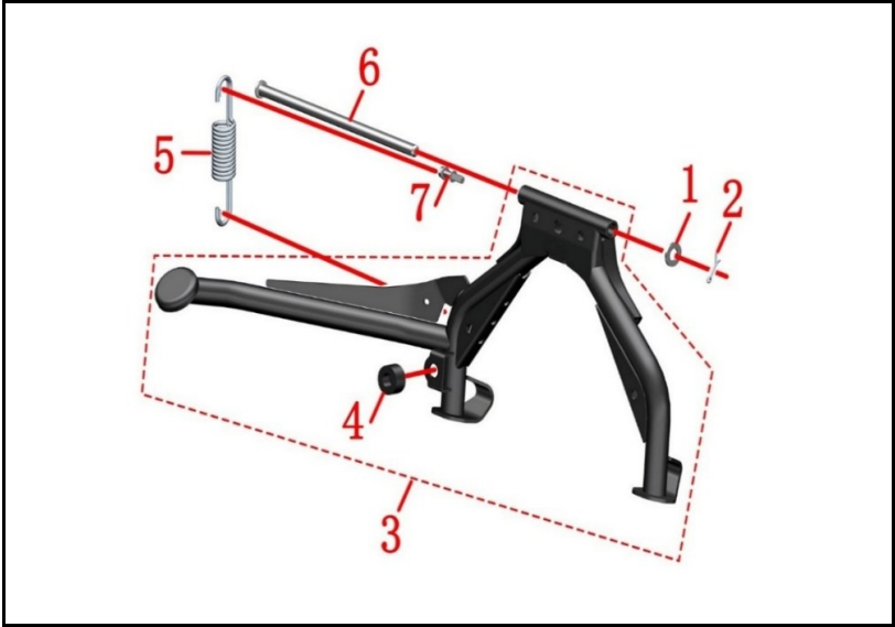
FIGURA N° 83: GATO CENTRAL
