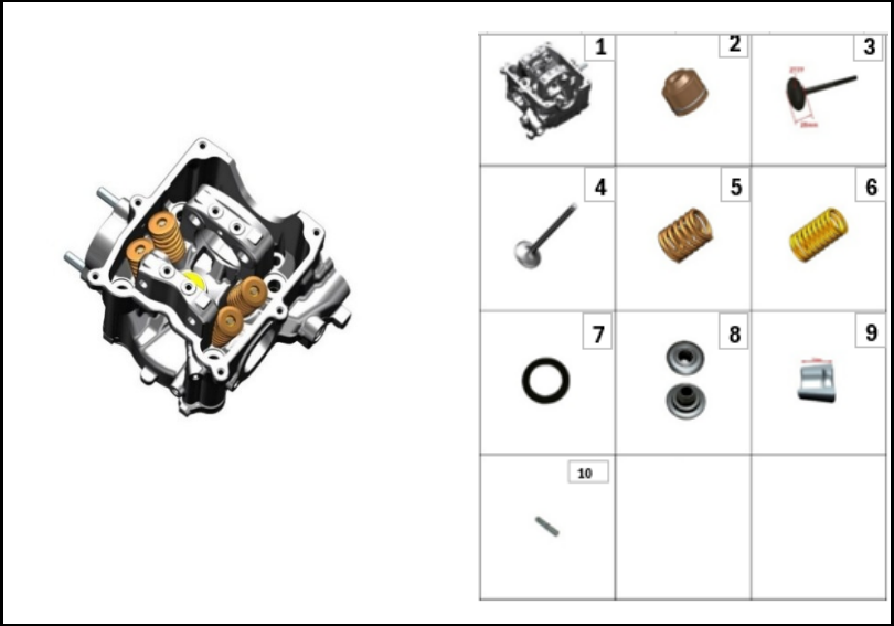
FIGURA N° 5: VALVULA
