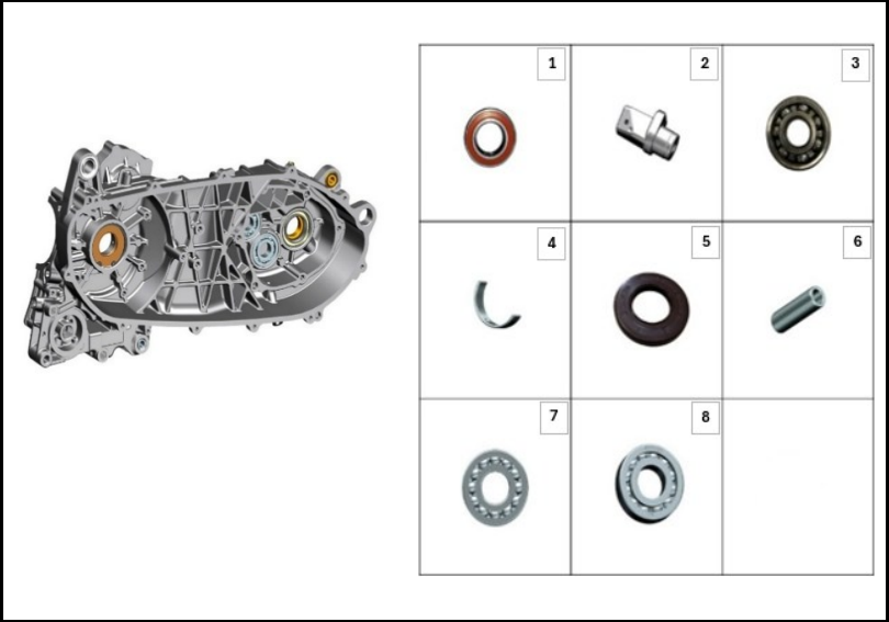
FIGURA N° 17: RODAMIENTO CARCASA MOTOR IZQUIERDA
