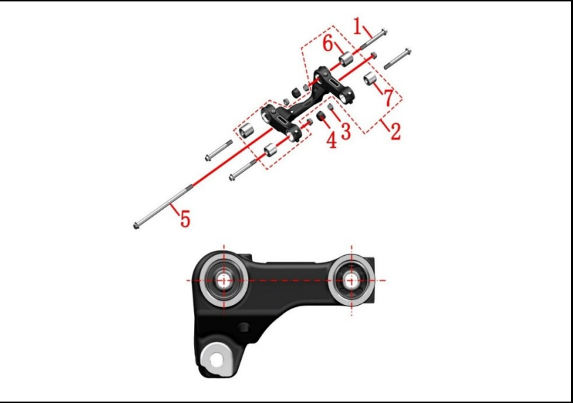
FIGURA N° 77: SOPORTE AMORTIGUADOR
