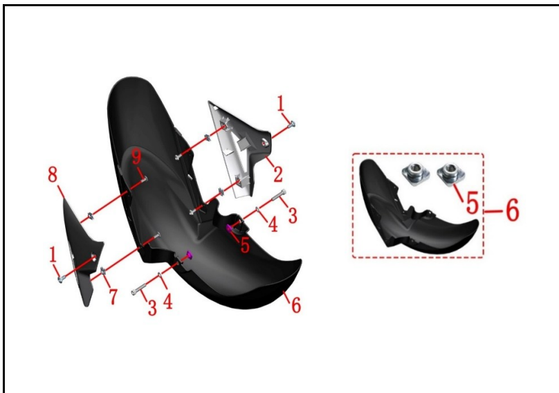
FIGURA N° 44: GUARDABARRO DELANTERO
