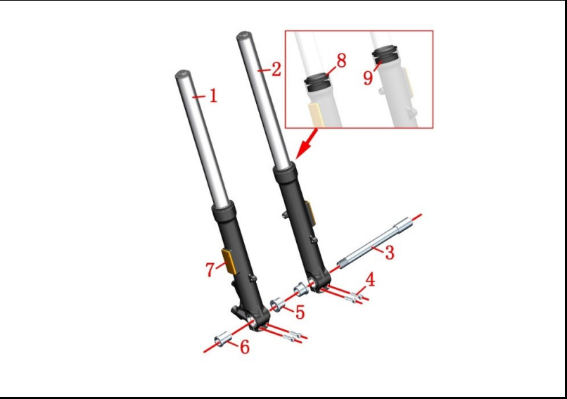
FIGURA N° 65: SUSPENSION DELANTERA
