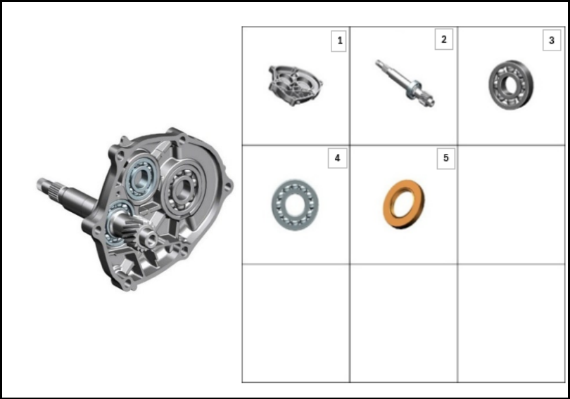
FIGURA N° 25: CUBIERTA TRANSMISION
