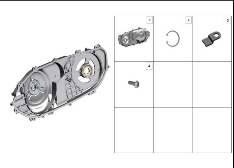
FIGURA N° 27: CUBIERTA IZQUIERDA MOTOR
