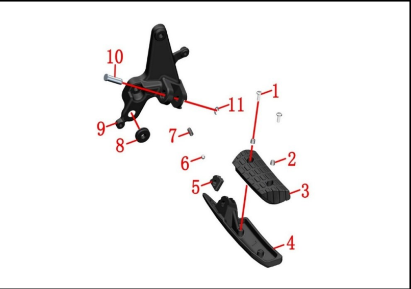
FIGURA N° 86: SOPORTE REPOSAPIE TRASERO IZQUIERDO
