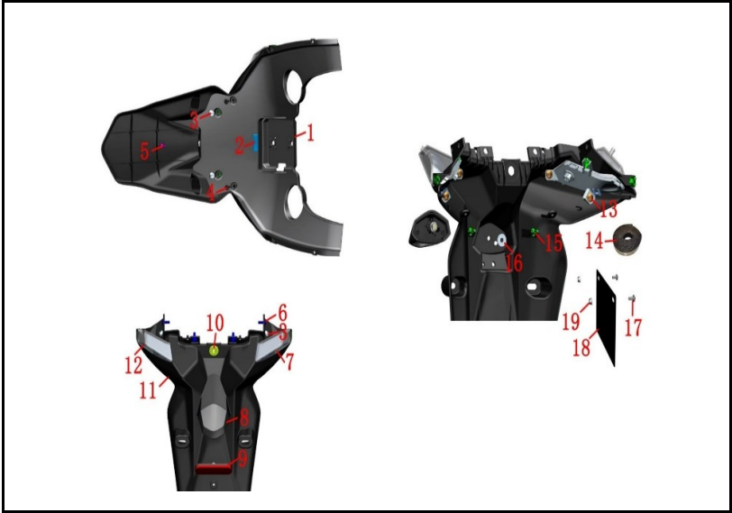
FIGURA N° 58: GUARDABARRO TRASERO
