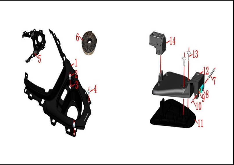
FIGURA N° 51: CUBIERTA COMBUSTIBLE
