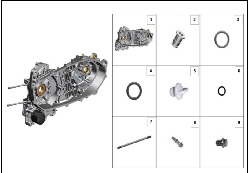
FIGURA N°14: COMPONENTES CARCASA MOTOR IZQUIERDA
