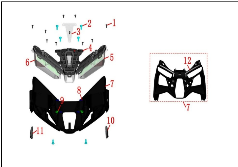
FIGURA N° 43: FAROLA
