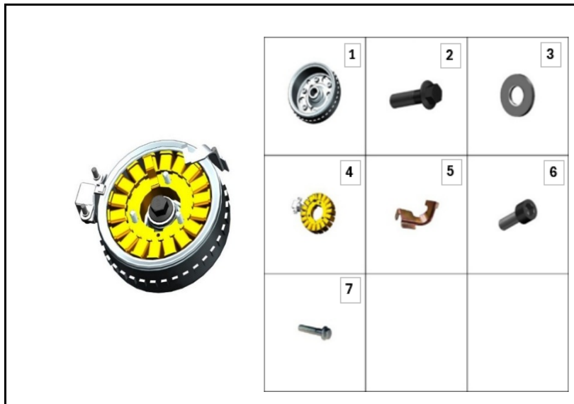
FIGURA N° 37: VOLANTE
