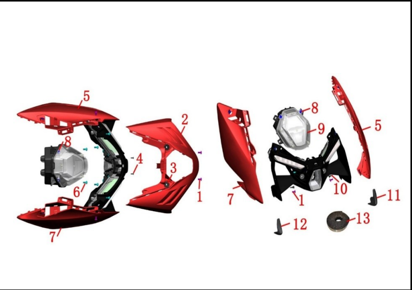
FIGURA N° 42: CARENAJE FAROLA
