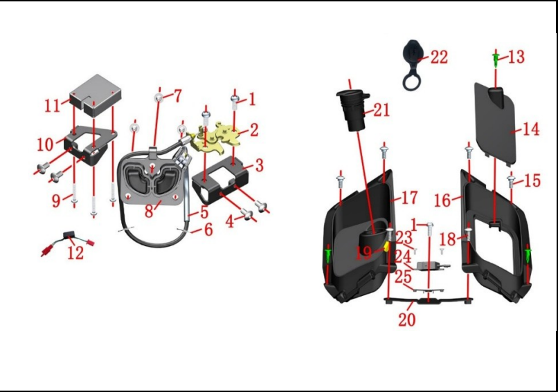
FIGURA N° 49: CUBIERTA GABINETE
