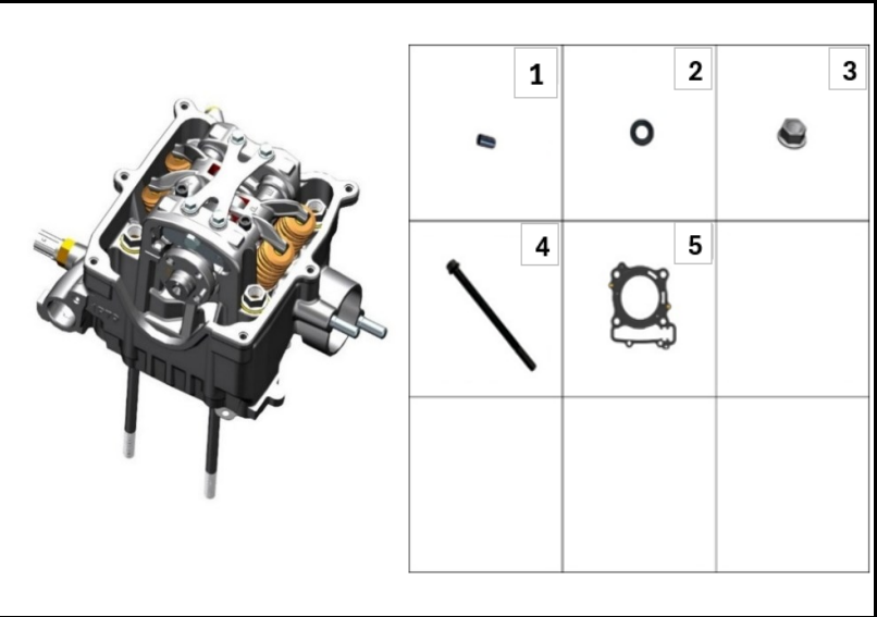
FIGURA N° 2: CULATA
