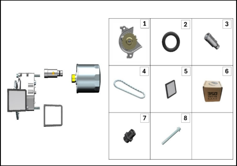
FIGURA N° 39: BOMBA ACEITE
