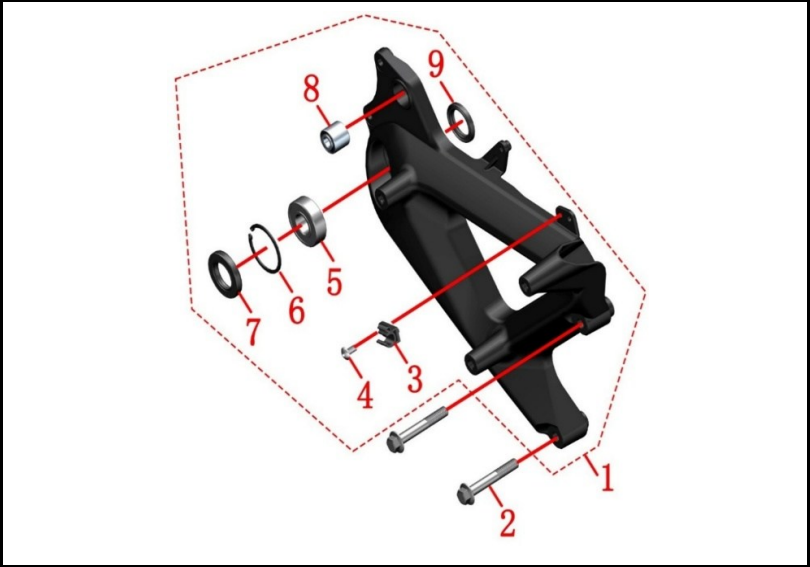
FIGURA N° 70: SOPORTE LATERAL
