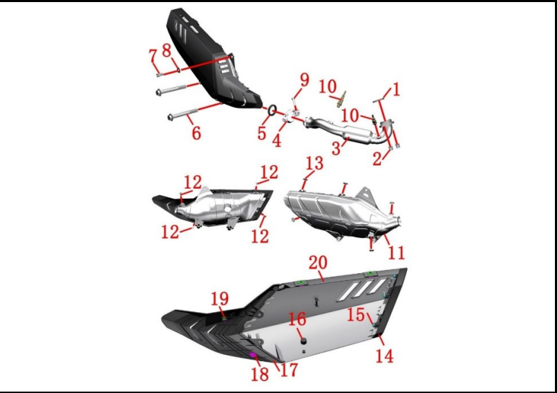
FIGURA N° 84: SILENCIADOR
