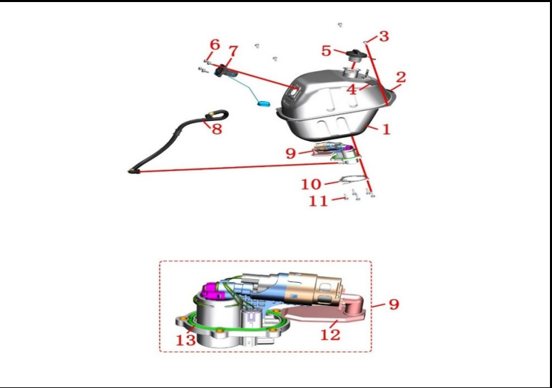
FIGURA N° 72: TANQUE COMBUSTIBLE
