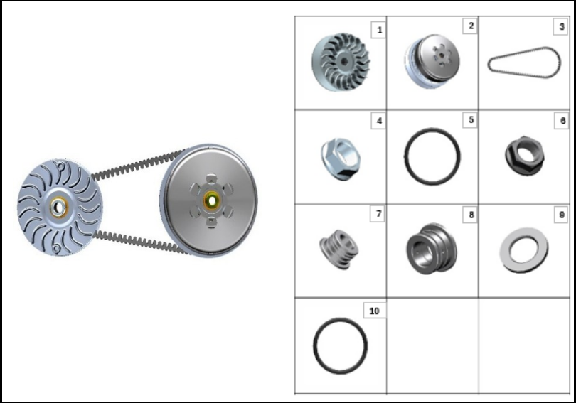
FIGURA N°9: CLUTCH
