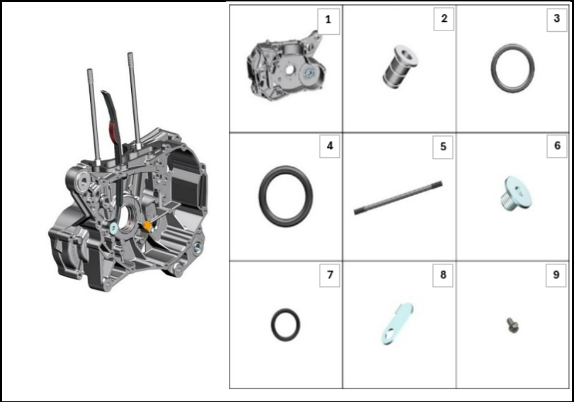
FIGURA N° 20: CARCASA MOTOR DERECHA
