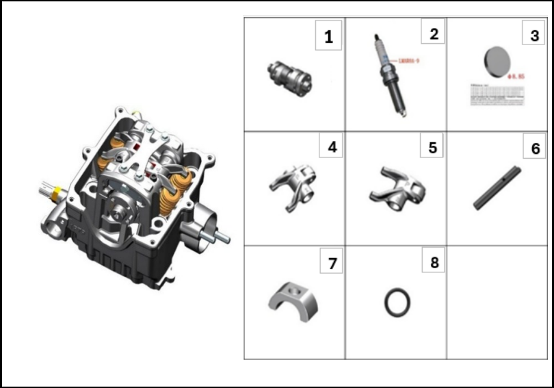
FIGURA N° 3: EJE LEVAS
