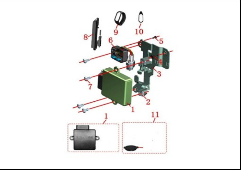
FIGURA N° 76: SISTEMA KEYLESS
