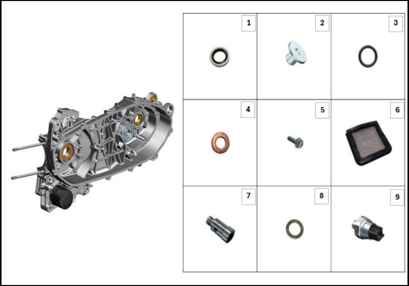
FIGURA N°15: COMPONENTES CARCASA MOTOR IZQUIERDA
