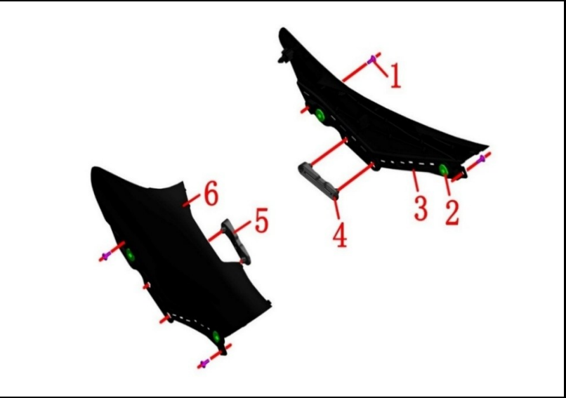
FIGURA N° 52: CUBIERTA LATERAL TANQUE COMBUSTIBLE
