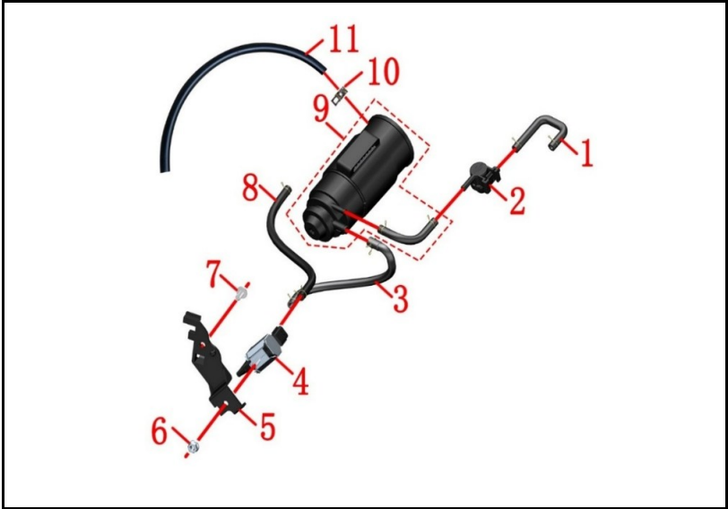
FIGURA N° 80: CANISTER
