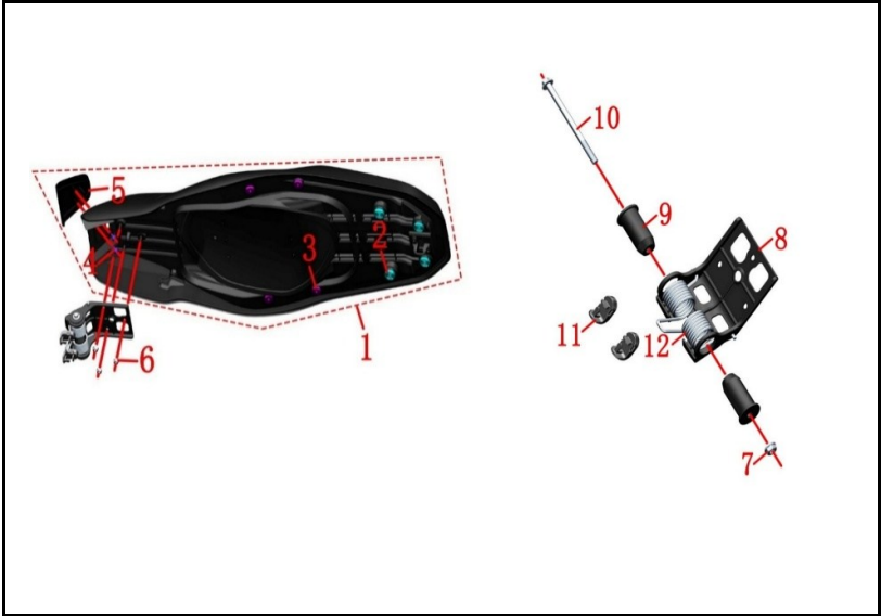
FIGURA N° 56: SILLIN
