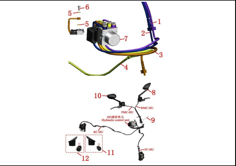
FIGURA N° 62: MODULO ABS
