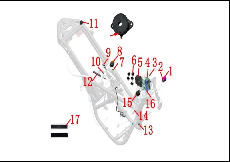
FIGURA N° 73: SISTEMA ELECTRICO
