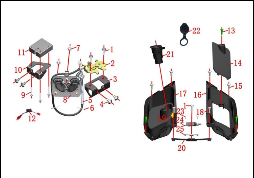
FIGURA N° 49: CUBIERTA GABINETE
