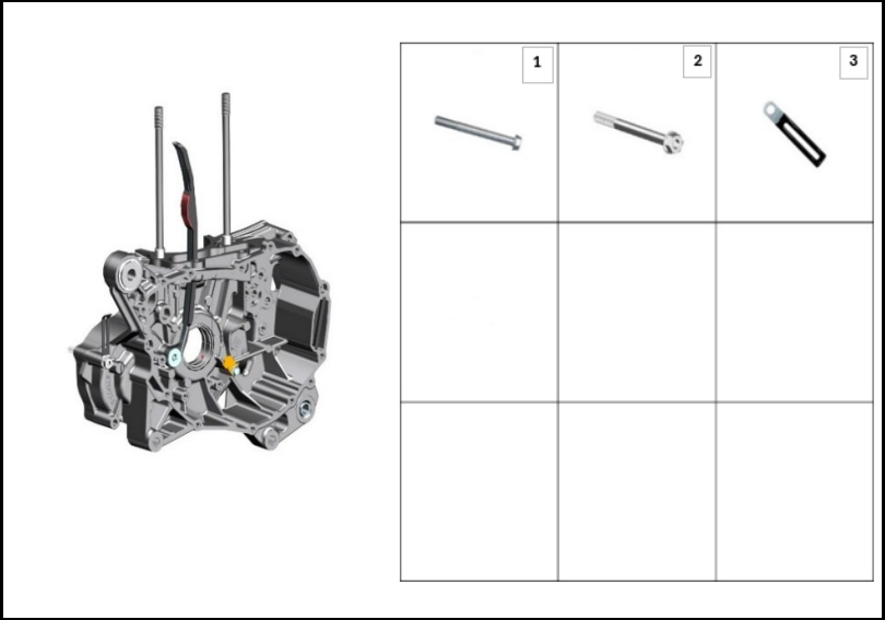
FIGURA N° 19: COMPONENTES CARCASA MOTOR DERECHA
