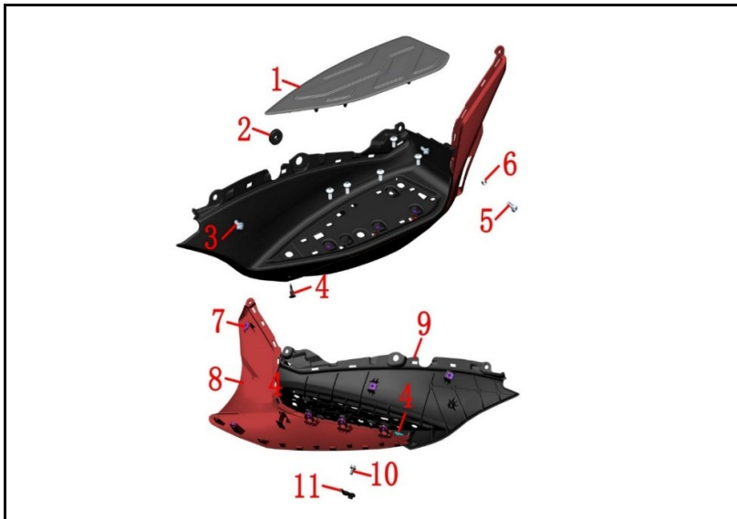
FIGURA N° 47: CUBIERTA PISO DERECHA
