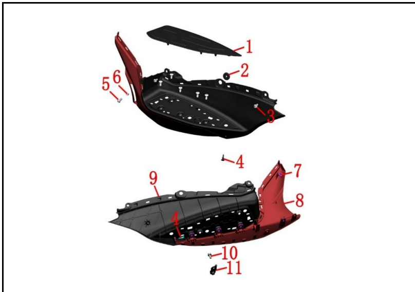
FIGURA N° 46: CUBIERTA PISO IZQUIERDA
