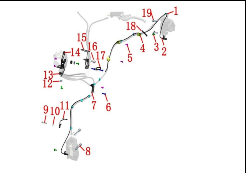
FIGURA N° 61: COMPLEMENTO MODULO ABS
