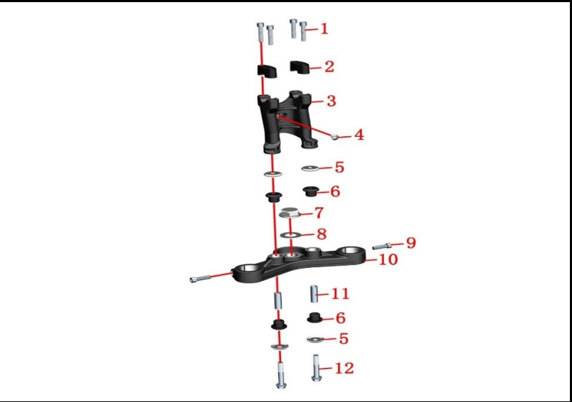
FIGURA N° 60: SOPORTE MANUBRIO
