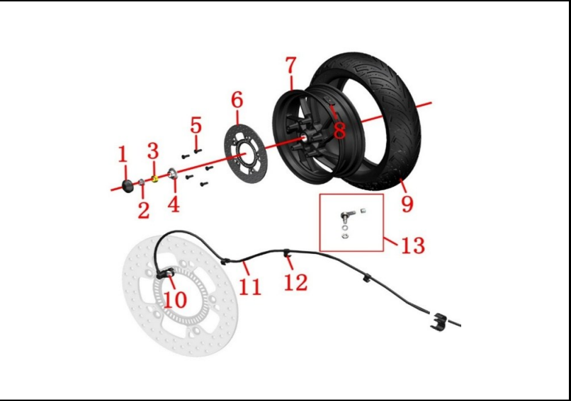
FIGURA N° 69: LLANTA TRASERA
