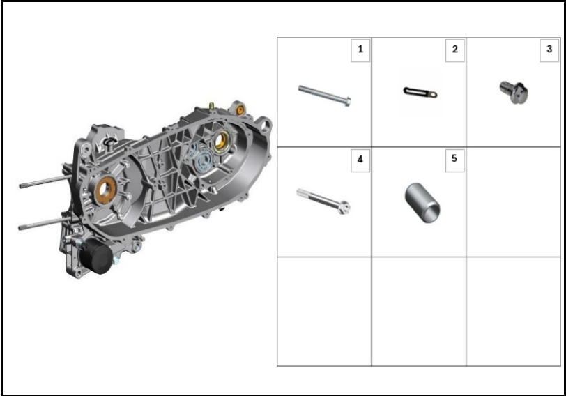
FIGURA N°13: GUIAS CARCASA MOTOR IZQUIERDA
