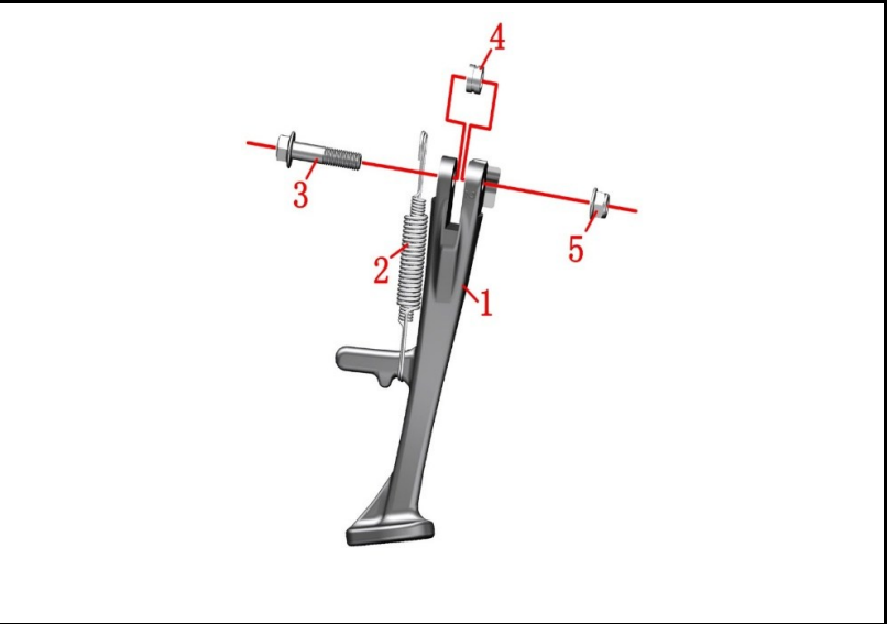
FIGURA N° 78: GATO LATERAL
