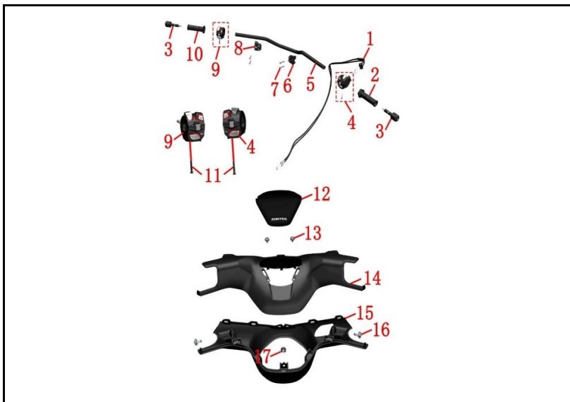
FIGURA N° 59: MANUBRIO
