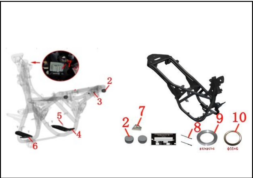
FIGURA N° 71: CHASIS
