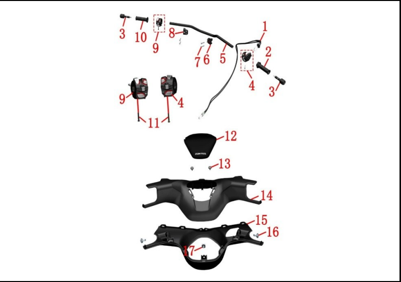
FIGURA N° 59: MANUBRIO
