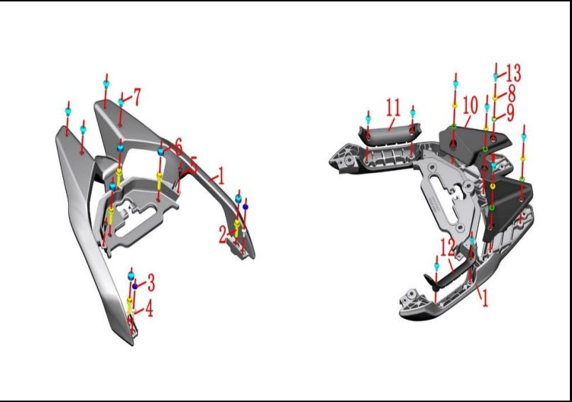
FIGURA N° 54: AGARRADERA TRASERA
