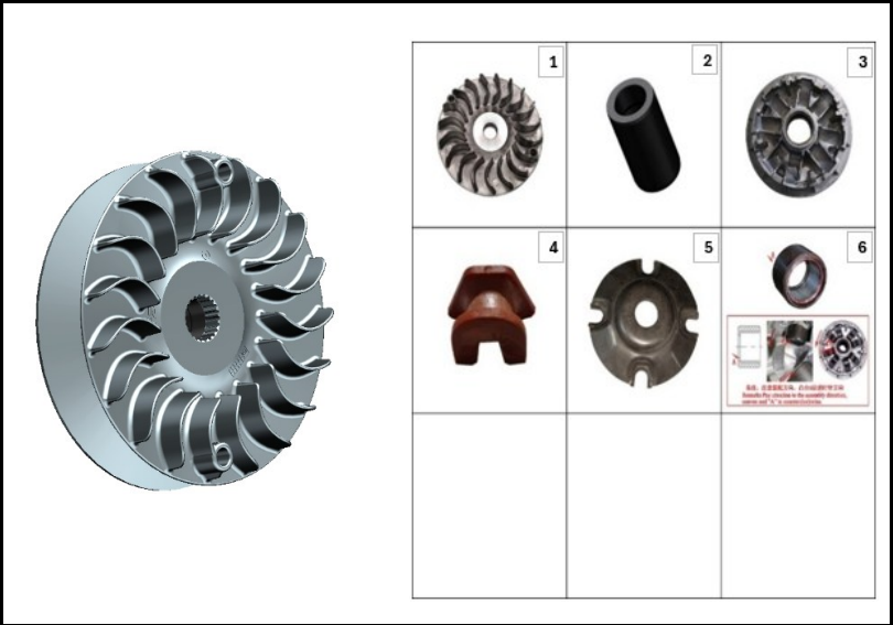
FIGURA N°10: VENTILADOR CVT
