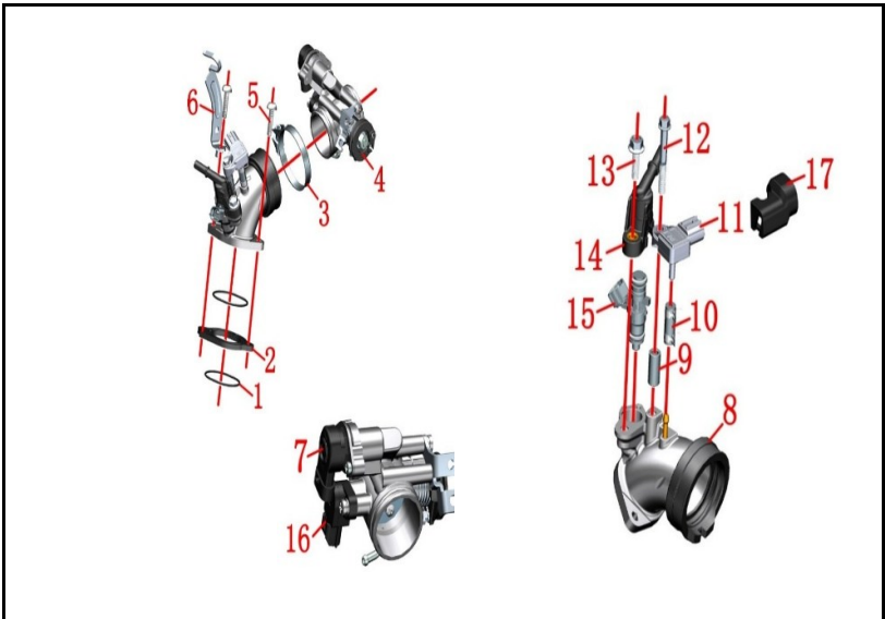
FIGURA N° 81: CUERPO ACELERACION
