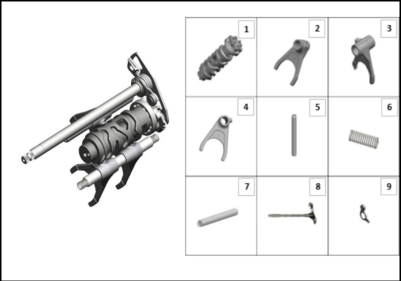
FIGURA N° 8: EJE CAMBIOS
