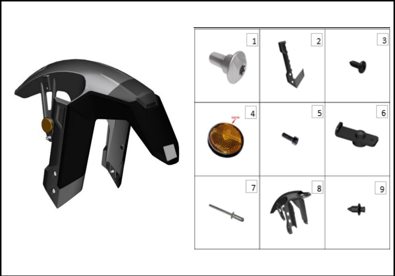
FIGURA N° 60: GUARDABARRO DELANTERO INTERNO
