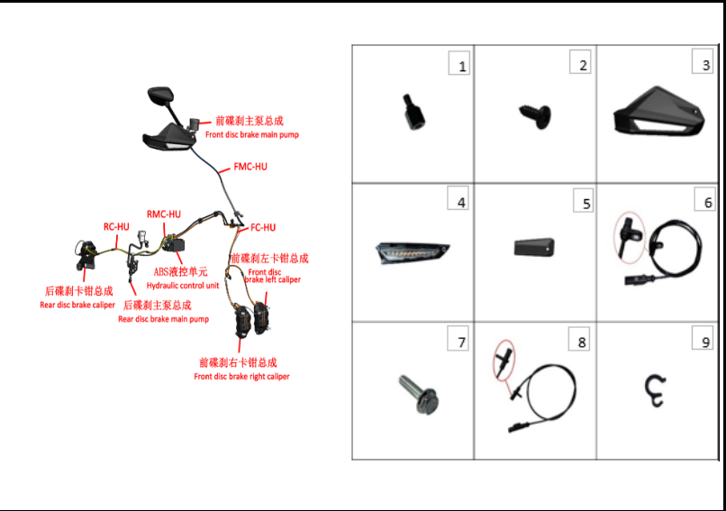
FIGURA N° 67: SISTEMA FRENOS
