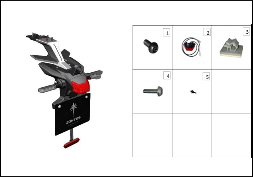
FIGURA N° 55: LUZ PLACA
