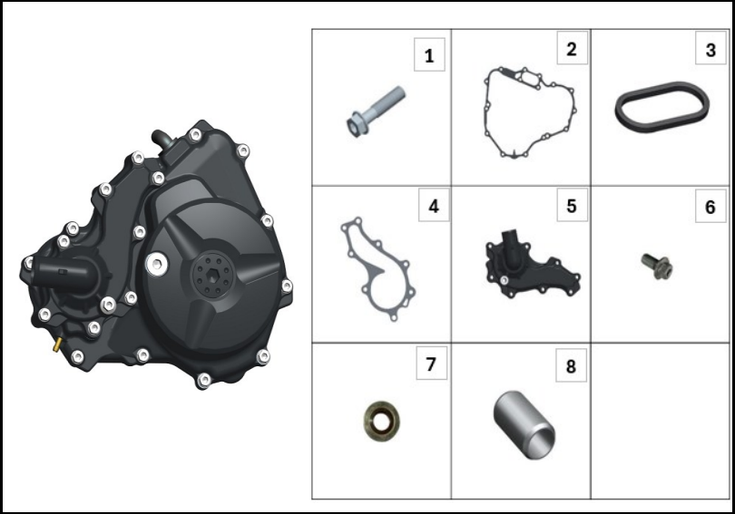
FIGURA N° 15: CUBIERTA VOLANTE
