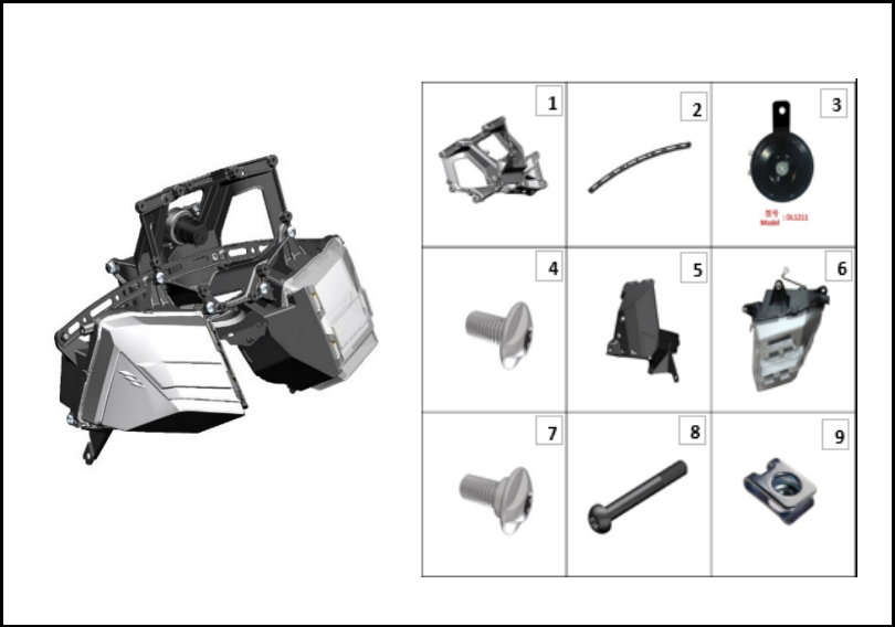
FIGURA N° 35: FAROLA IZQUIERDA
