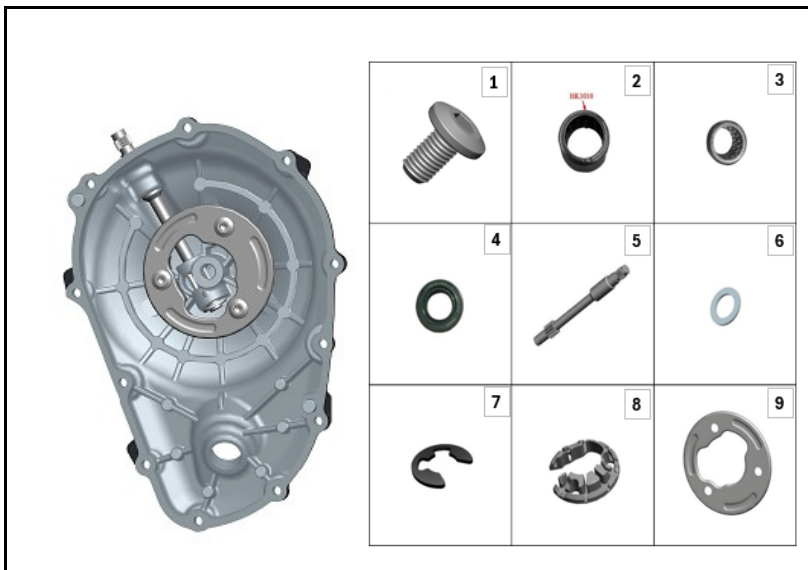
FIGURA N° 22: CUBIERTA CLUTCH
