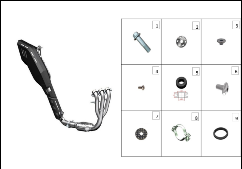
FIGURA N° 112: COMPONENTES SILENCIADOR
