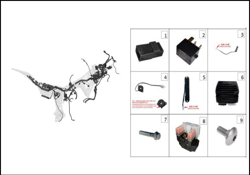
FIGURA N° 88: SISTEMA ELECTRICO
