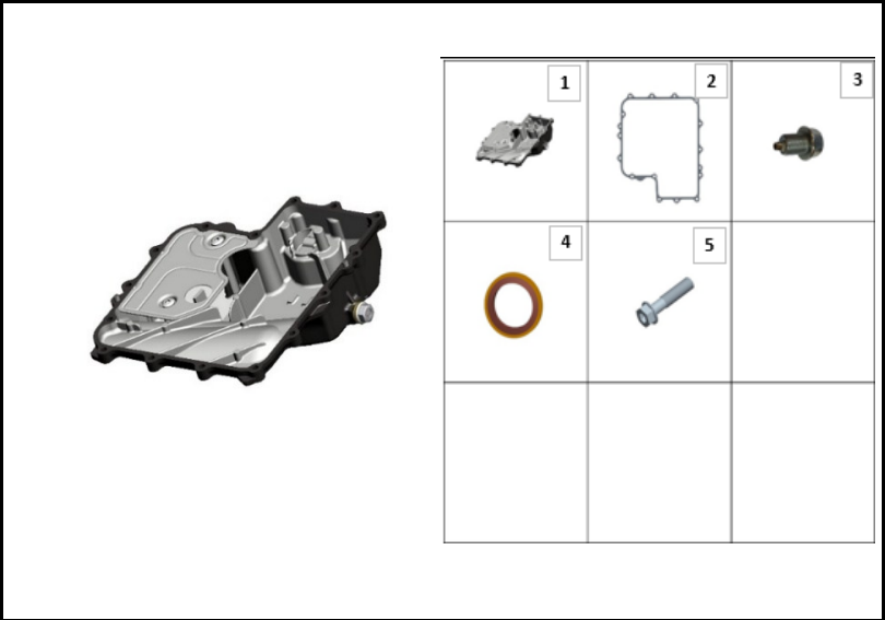
FIGURA N° 24: CUBIERTA PIÑON
