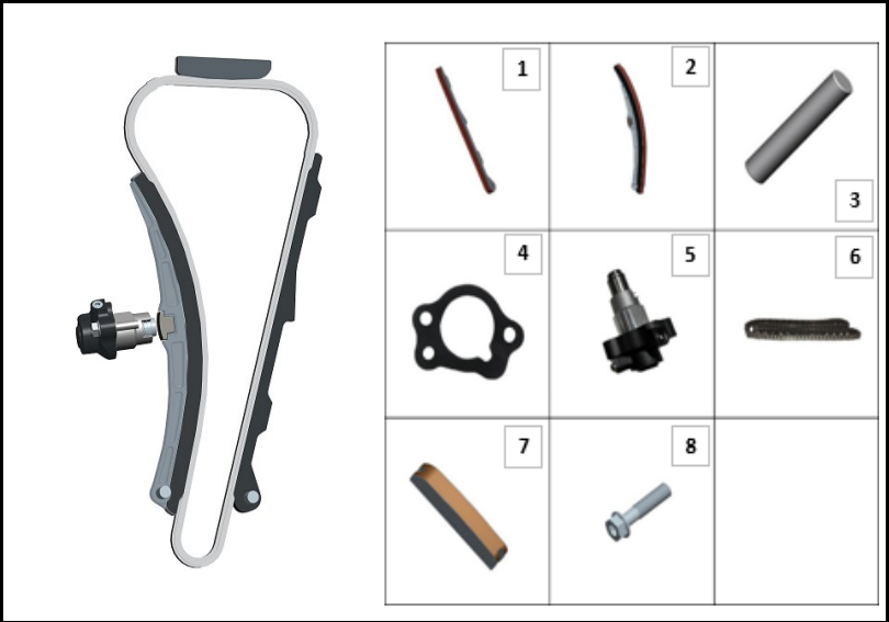
FIGURA N° 6: CADENILLA DISTRIBUCION
