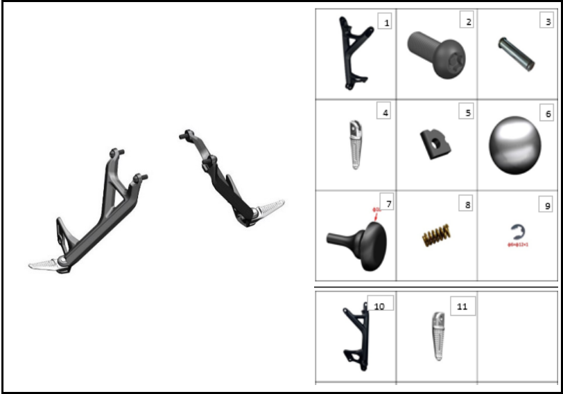
FIGURA N° 104: SOPORTE REPOSAPIE TRASERO
