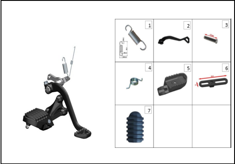
FIGURA N° 103: PEDAL FRENO
