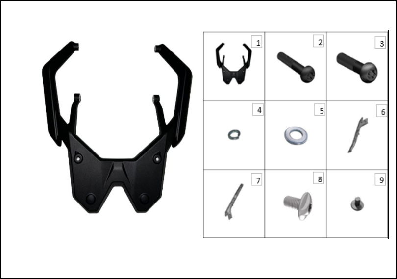
FIGURA N° 52: AGARRADERA TRASERA
