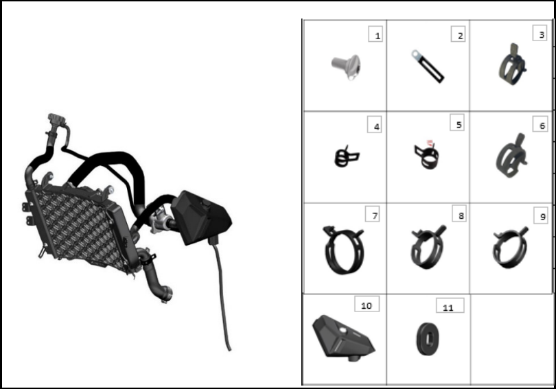
FIGURA N° 107: CUBIERTA TANQUE RESERVORIO
