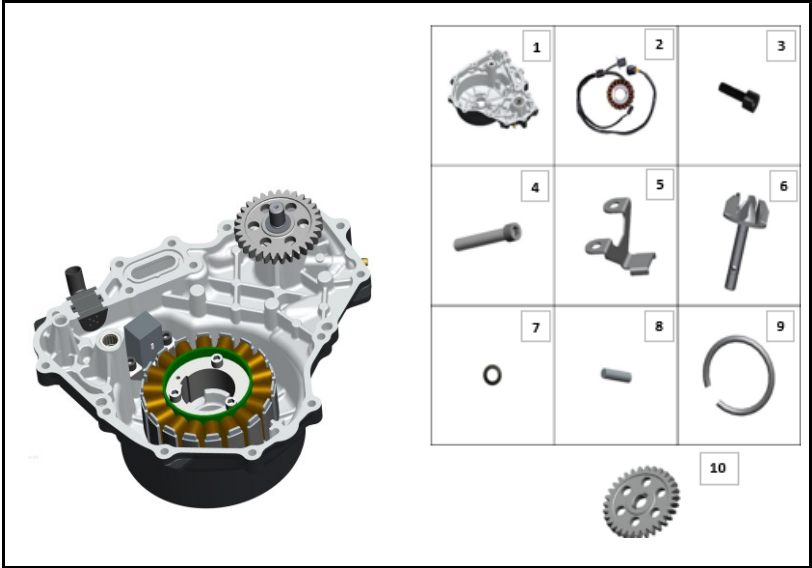
FIGURA N° 17: CUBIERTA VOLANTE
