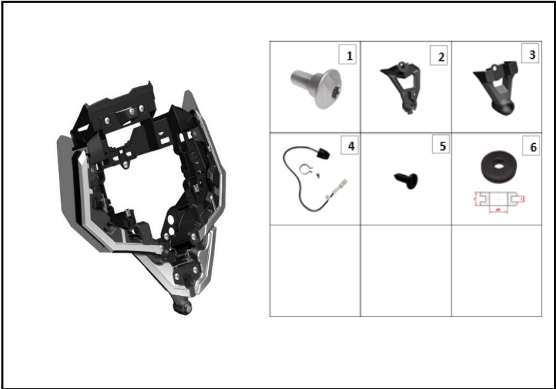
FIGURA N° 32: SOPORTE DIRECCIONAL
