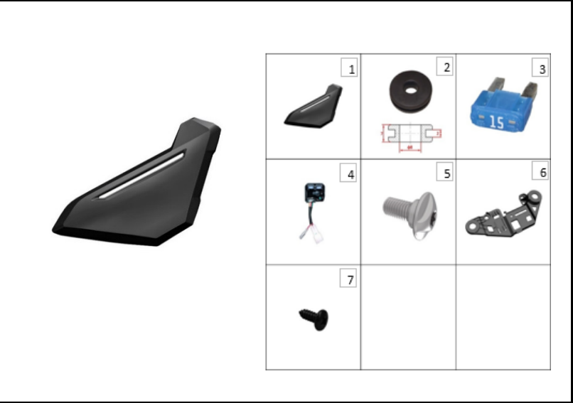
FIGURA N° 57: CUBIERTA LATERAL PUERTO CARGA
