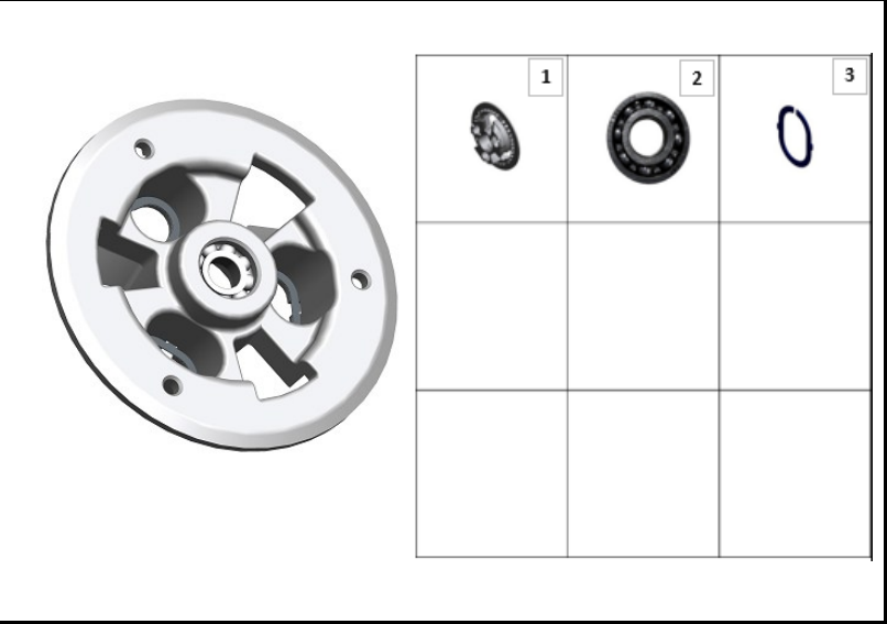
FIGURA N° 14: PRENSA CLUTCH
