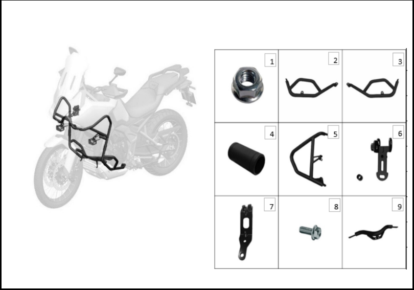
FIGURA N° 116: DEFENSA
