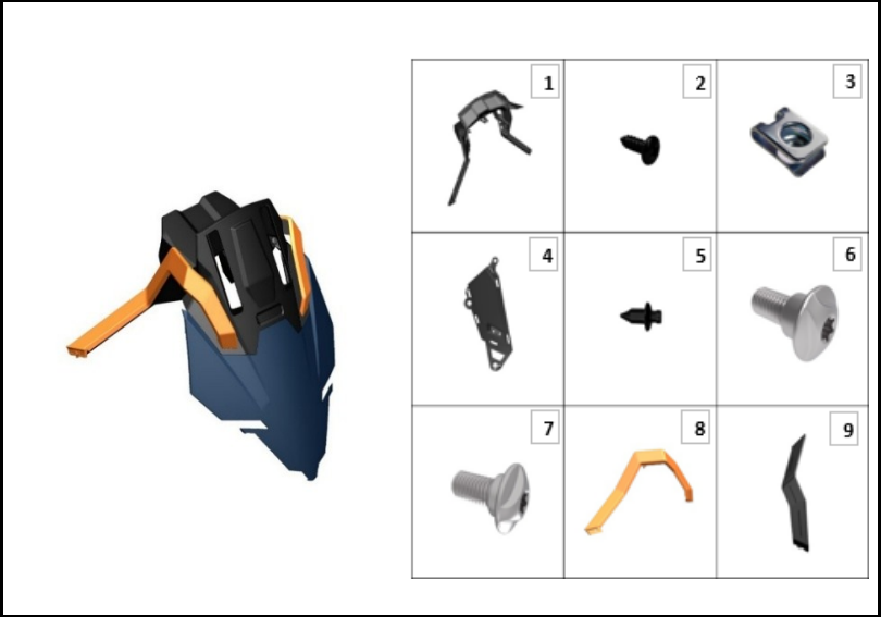
FIGURA N°29: SOPORTE VISOR
