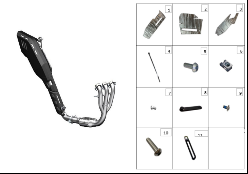
FIGURA N° 112: COMPONENTES SILENCIADOR
