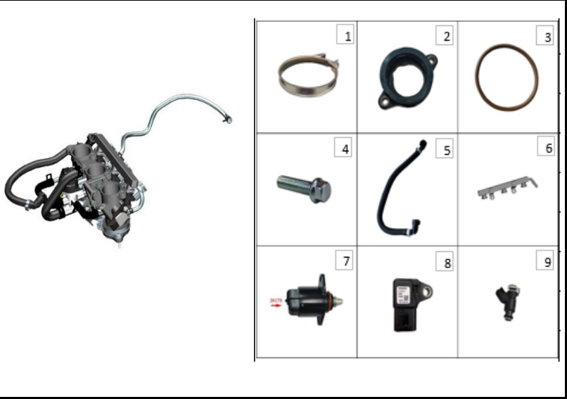
FIGURA N° 93: SENSORES CUERPO INYECCION
