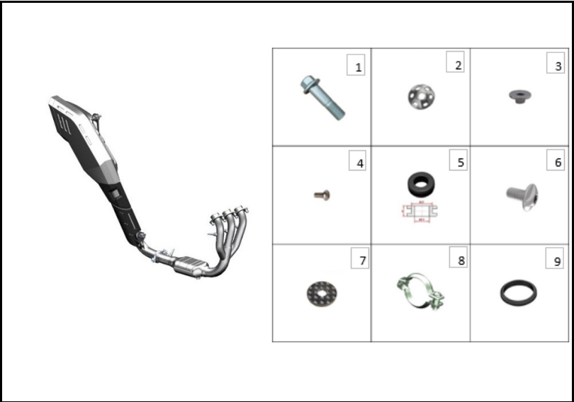
FIGURA N° 110: COMPONENTES SILENCIADOR
