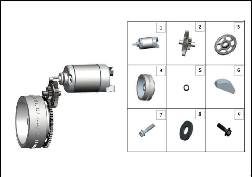
FIGURA N° 20: MOTOR ARRANQUE
