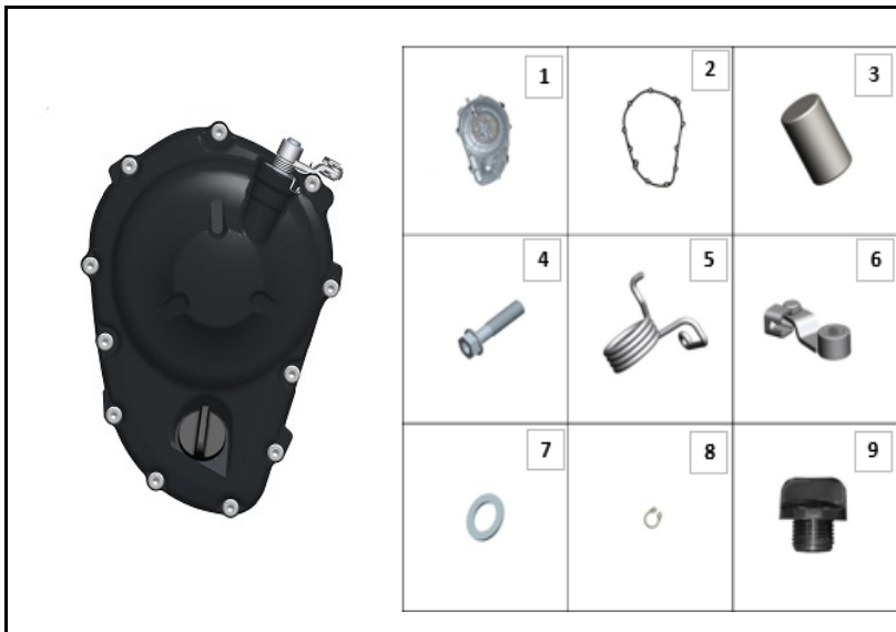
FIGURA N° 21: CUBIERTA CLUTCH
