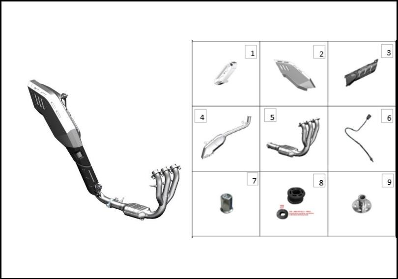
FIGURA N° 109: SILENCIADOR
