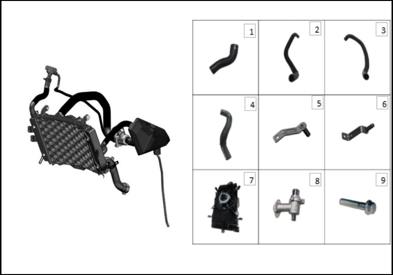
FIGURA N° 105: RADIADOR
