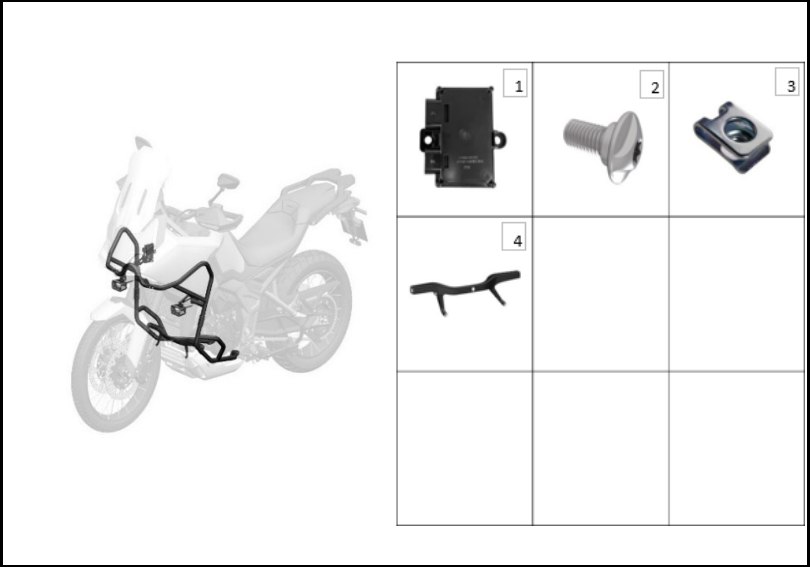
FIGURA N° 117: SOPORTE DEFENSA
