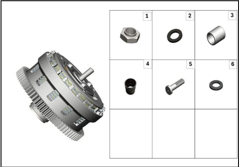
FIGURA N° 10: CLUTCH
