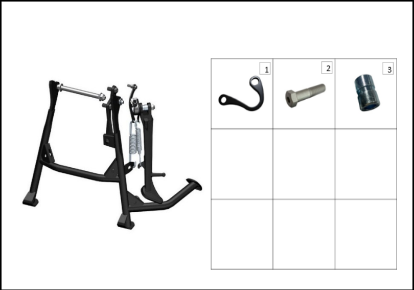
FIGURA N° 91: COMPONENTES GATO CENTRAL
