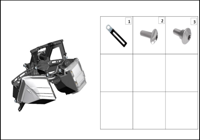
FIGURA N° 37: COMPLEMENTOS FAROLA
