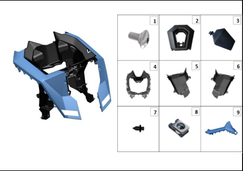
FIGURA N° 33: CUBIERTA FRONTAL DERECHA
