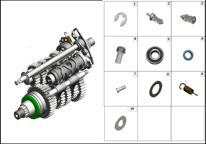
FIGURA N° 7:TRANSMISIÓN
