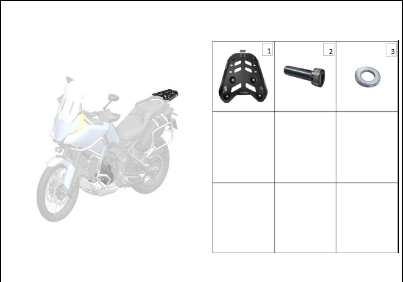
FIGURA N° 120: BASE MALETERO
