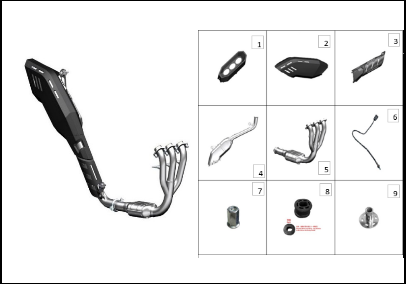
FIGURA N° 111: SILENCIADOR
