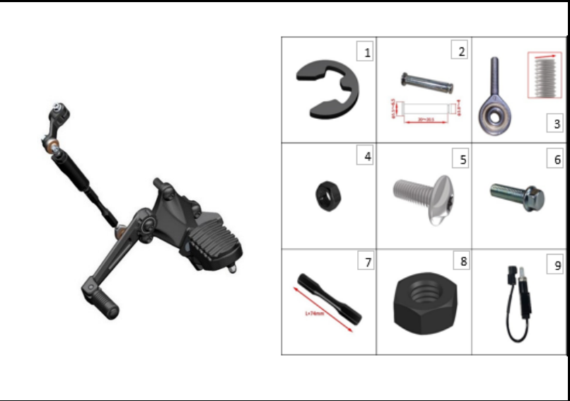
FIGURA N° 100: CONJUNTO PEDAL FRENO TRASERO
