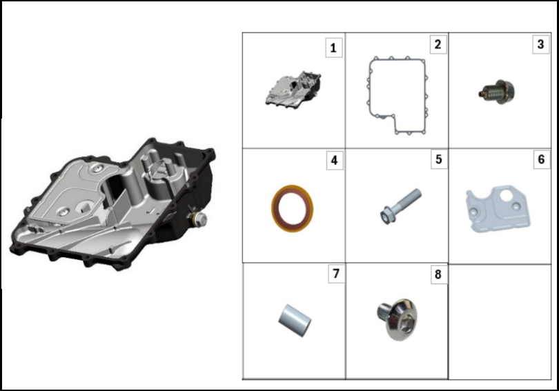
FIGURA N° 25: CARTER ACEITE
