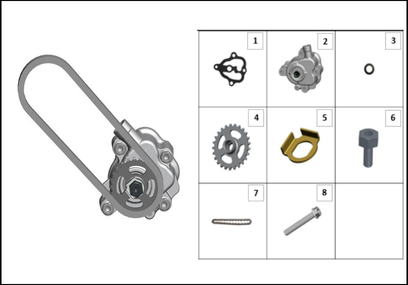
FIGURA N° 19: BOMBA AGUA
