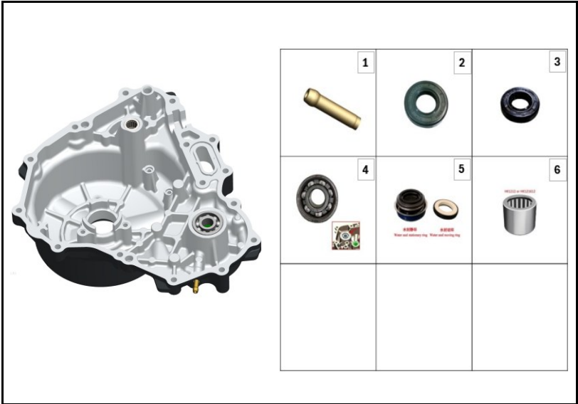
FIGURA N° 18: COMPONENTES CUBIERTA VOLANTE
