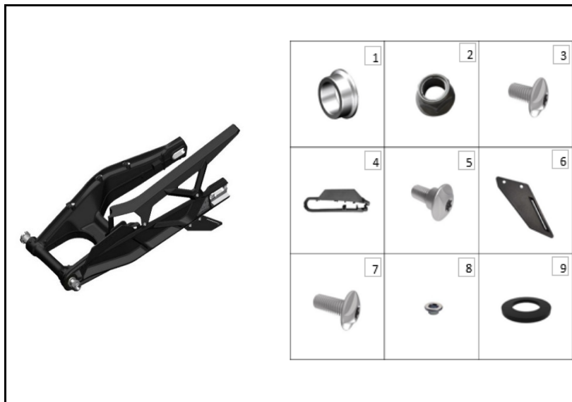
FIGURA N° 74: COMPLEMENTOS BRAZO OSCILANTE
