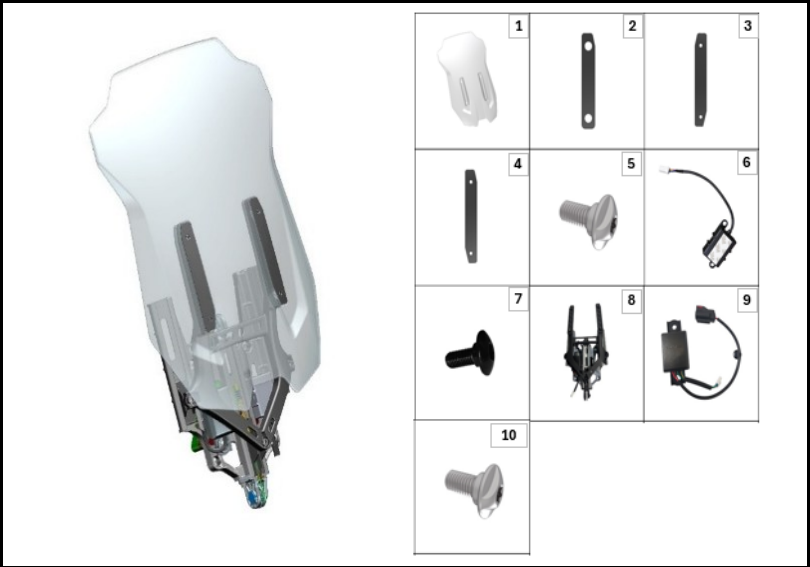
FIGURA N° 26: VISOR
