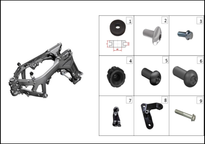
FIGURA N° 82: COMPONENTES CHASIS
