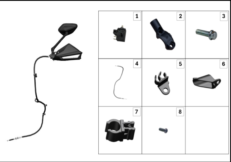
FIGURA N°64: CABLE CLUTCH
