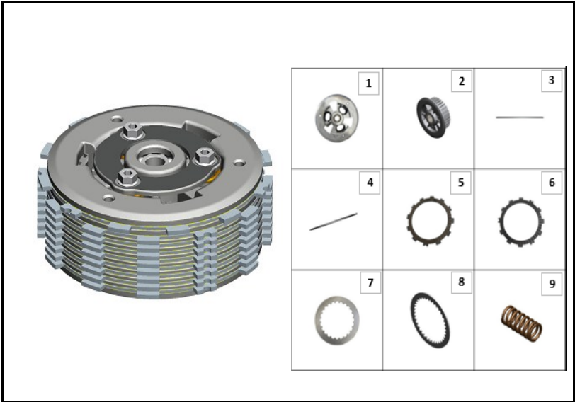
FIGURA N° 12: CLUTCH
