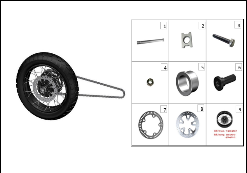
FIGURA N° 78: RIN TRASERO
