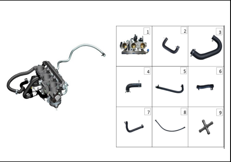
FIGURA N° 92: CUERPO INYECCION
