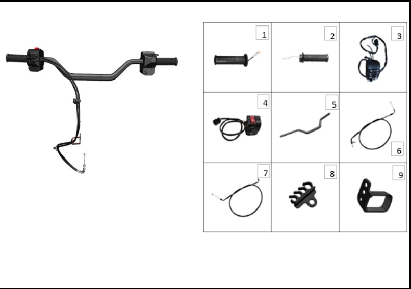
FIGURA N° 62: MANUBRIO
