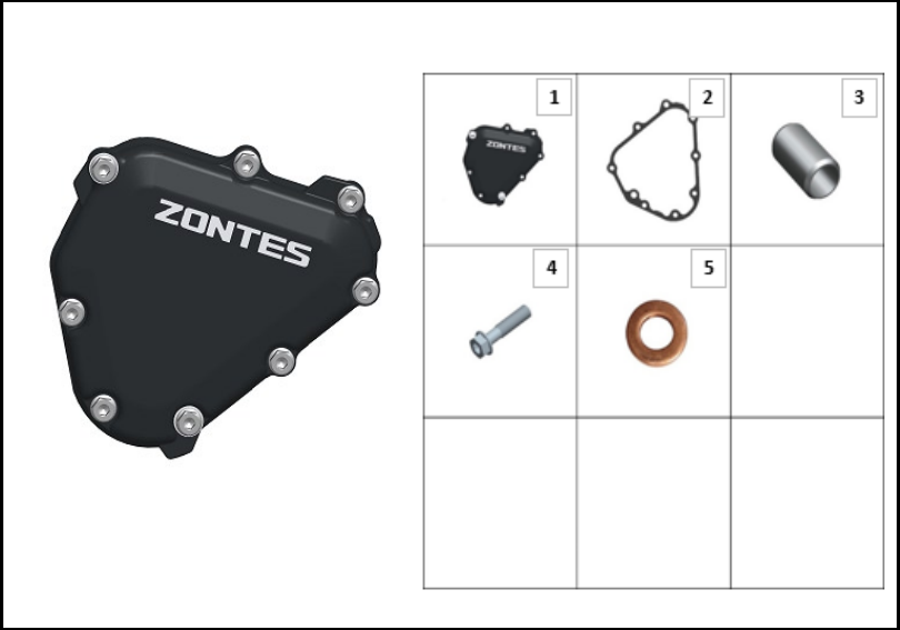
FIGURA N° 23: CUBIERTA PIÑON
