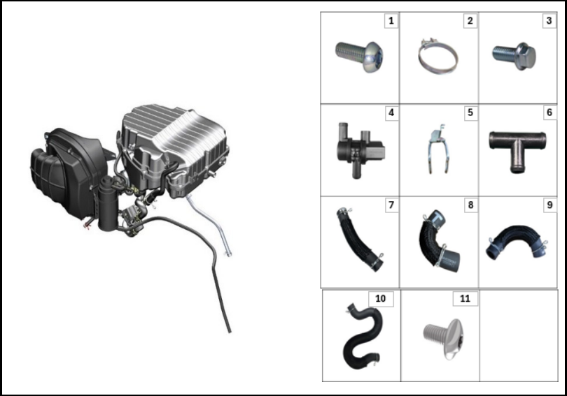
FIGURA N° 97: COMPONENTES CAJA FILTRO AIRE
