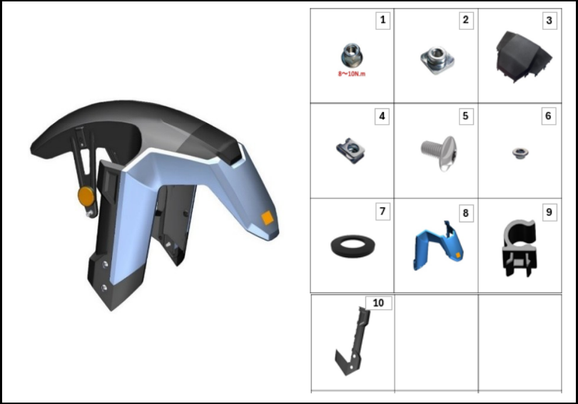
FIGURA N° 59: GUARDABARRO DELANTERO IZQUIERDO
