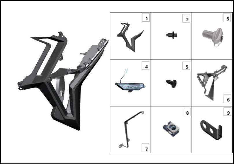
FIGURA N° 45: DIRECCIONAL LATERAL DERECHA
