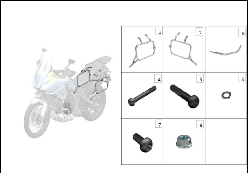
FIGURA N° 118: SOPORTE ALFORJAS
