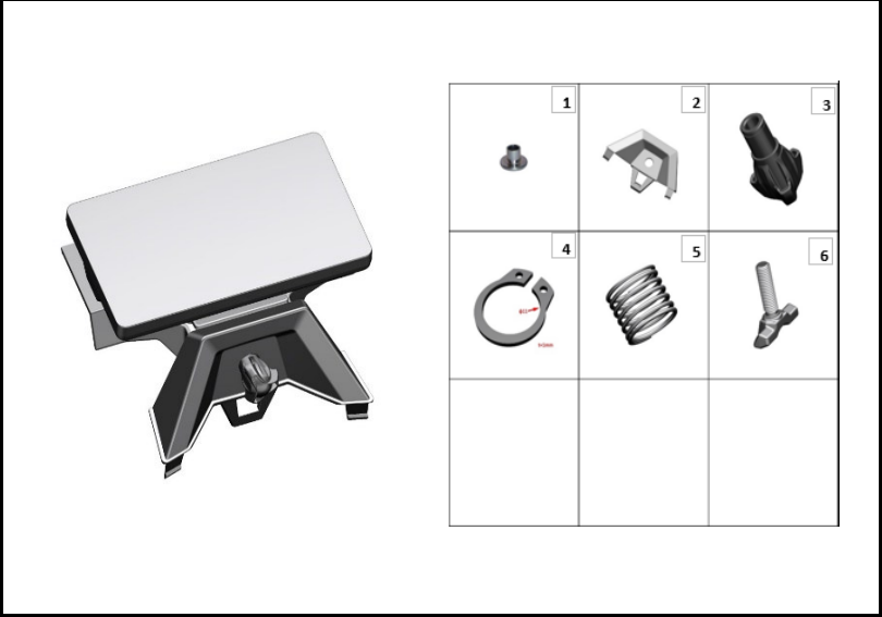
FIGURA N°28: VELOCIMETRO
