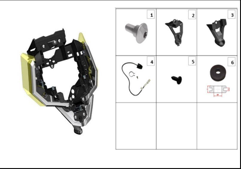
FIGURA N° 31: SOPORTE DIRECCIONAL
