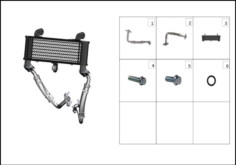
FIGURA N° 108: TUBOS RADIADOR
