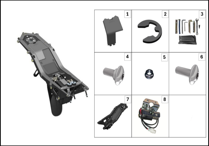
FIGURA N° 83: CERRADURA ELECTRONICA SILLIN
