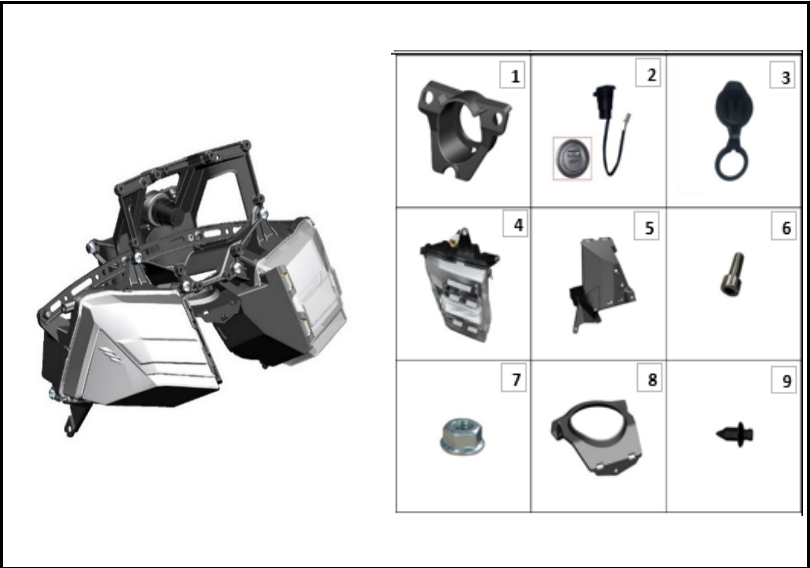
FIGURA N° 36: FAROLA DERECHA
