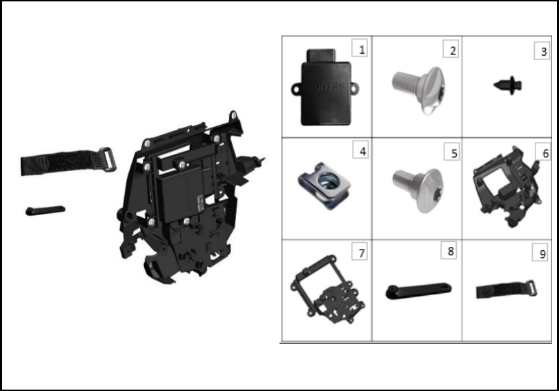
FIGURA N° 89: CONTROLADOR LUCES
