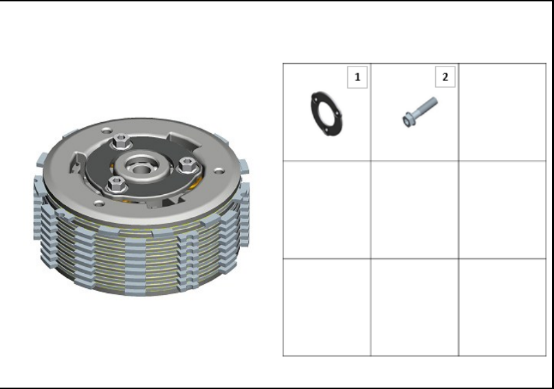
FIGURA N° 13: CLUTCH
