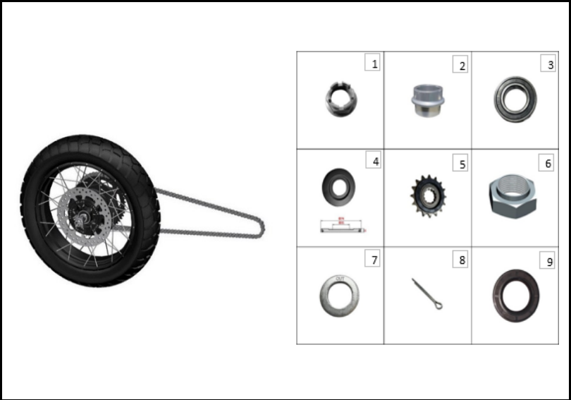
FIGURA N° 80: PIÑON SALIDA
