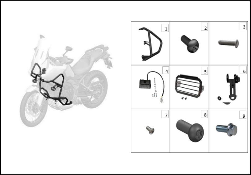
FIGURA N° 115: EXPLORADORAS
