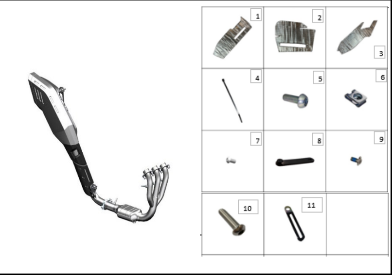
FIGURA N° 110: COMPONENTES SILENCIADOR
