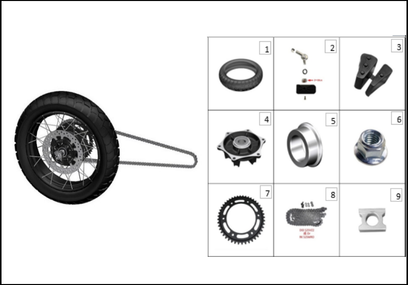
FIGURA N° 79: RUEDA TRASERA
