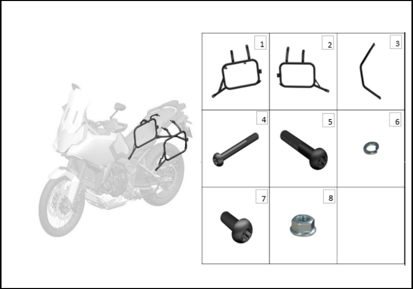
FIGURA N° 119: SOPORTE ALFORJAS
