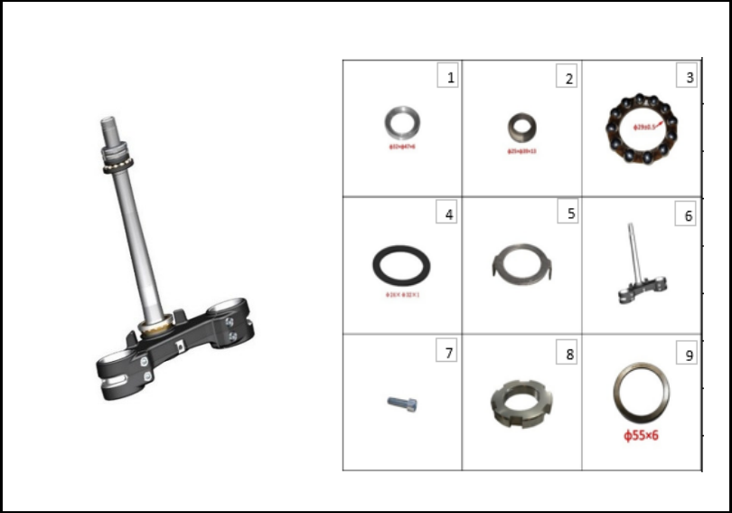
FIGURA N° 81: ESIPIGA CENTRAL
