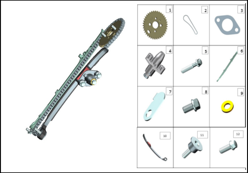
FIGURA N° 26: CADENILLA DISTRIBUCION
