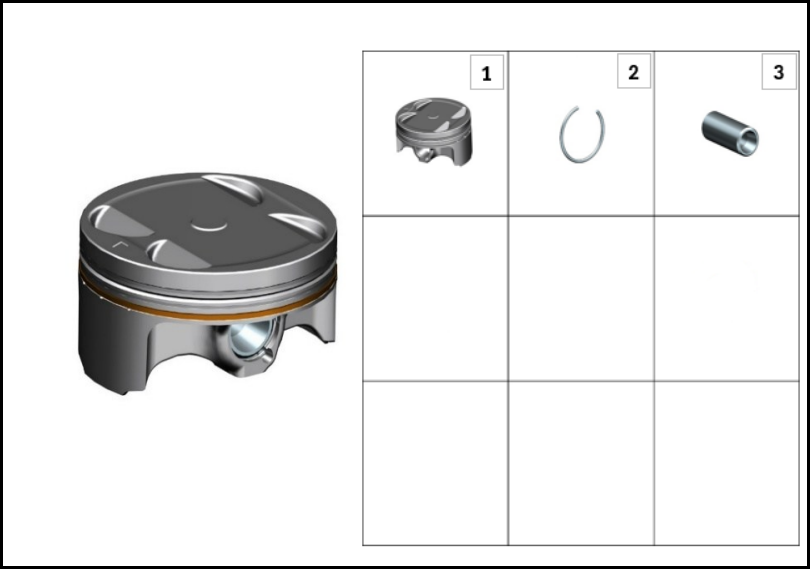
FIGURA N°5: PISTON
