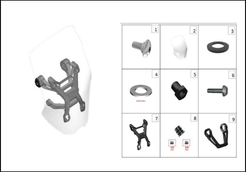
FIGURA N° 28: VISOR
