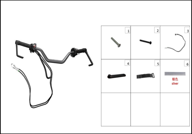
FIGURA N° 71:COMPLEMENTOS MANUBRIO
