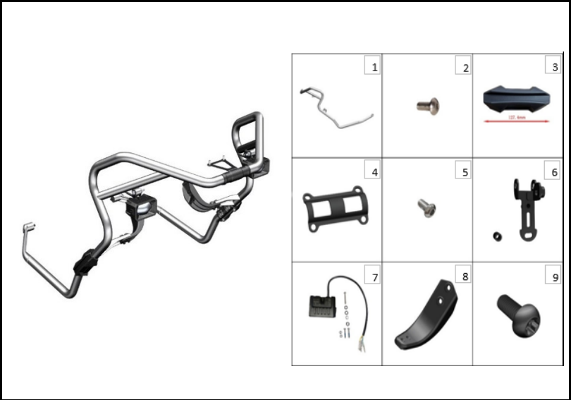
FIGURA N° 68: DEFENSA IZQUIERDA
