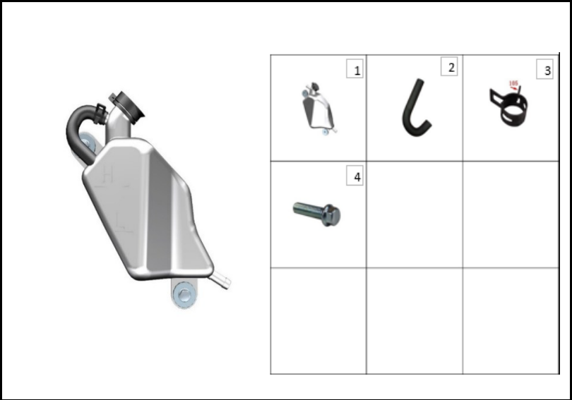
FIGURA N° 120: TANQUE RESERVORIO
