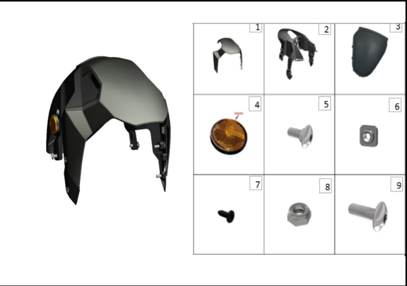
FIGURA N° 55: GUARDABARRO DELANTERO
