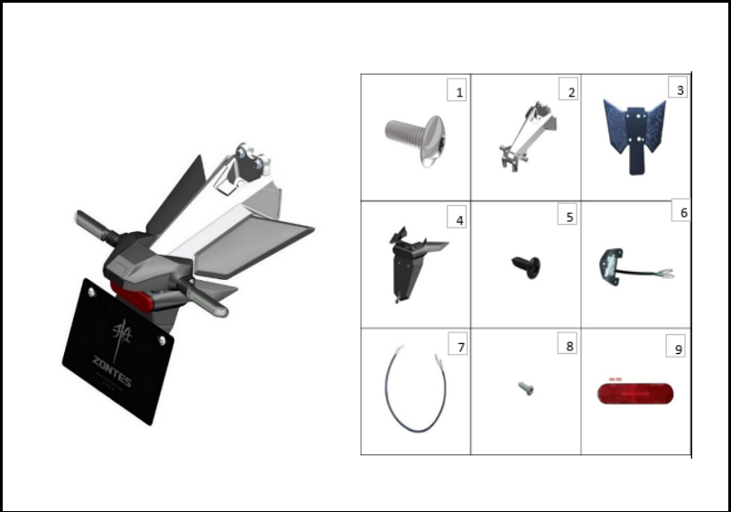
FIGURA N°60: GUARDABARRO TRASERO
