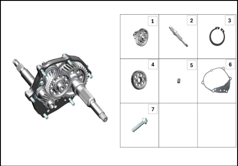
FIGURA N° 15: EJE SALIDA
