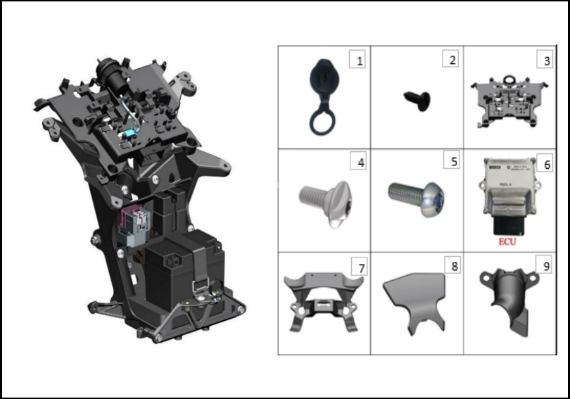
FIGURA N° 92: ECU
