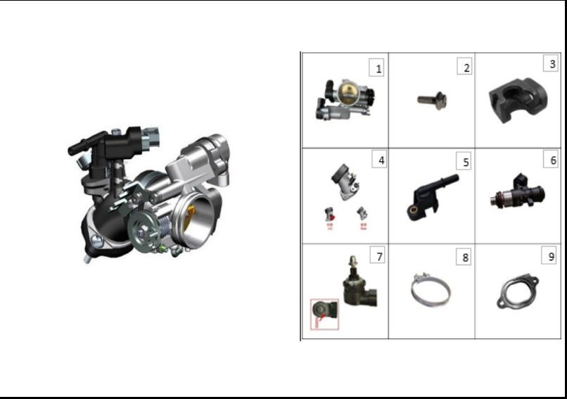
FIGURA N° 107: CUERPO ACELERACION
