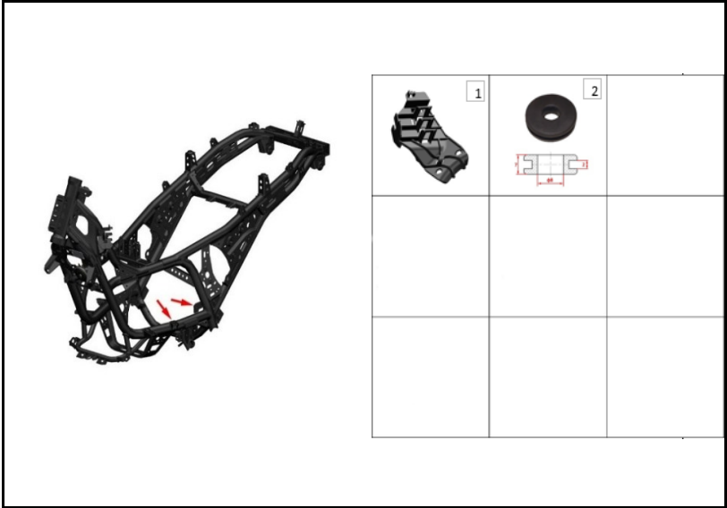
FIGURA N° 90:COMPLEMENTOS CHASIS
