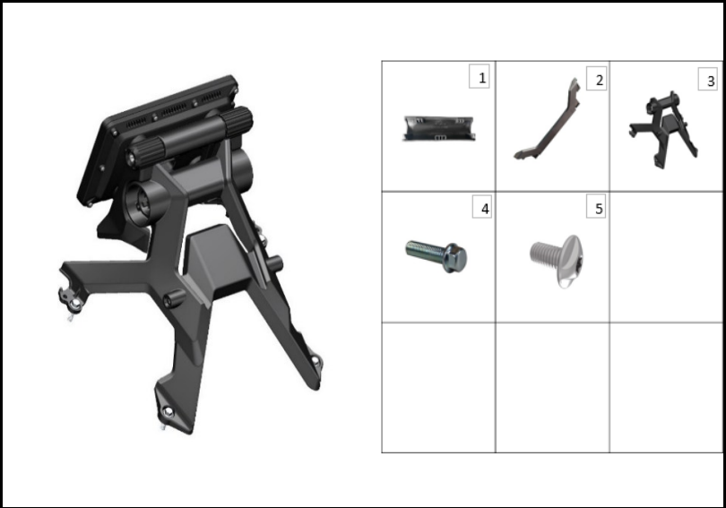
FIGURA N° 31: COMPONENTES VELOCIMETRO
