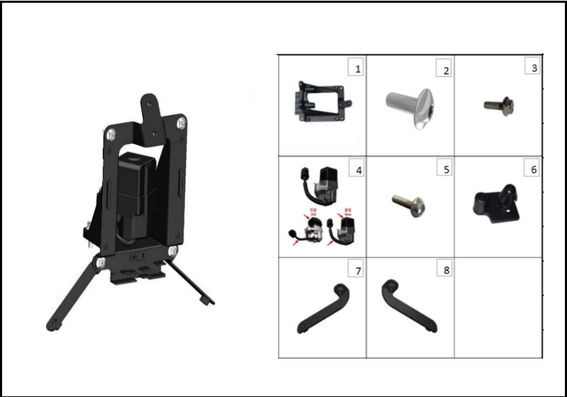
FIGURA N° 45: CERRADURA ELECTRONICA
