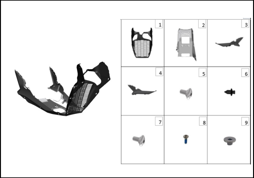
FIGURA N° 48: DEFLECTOR
