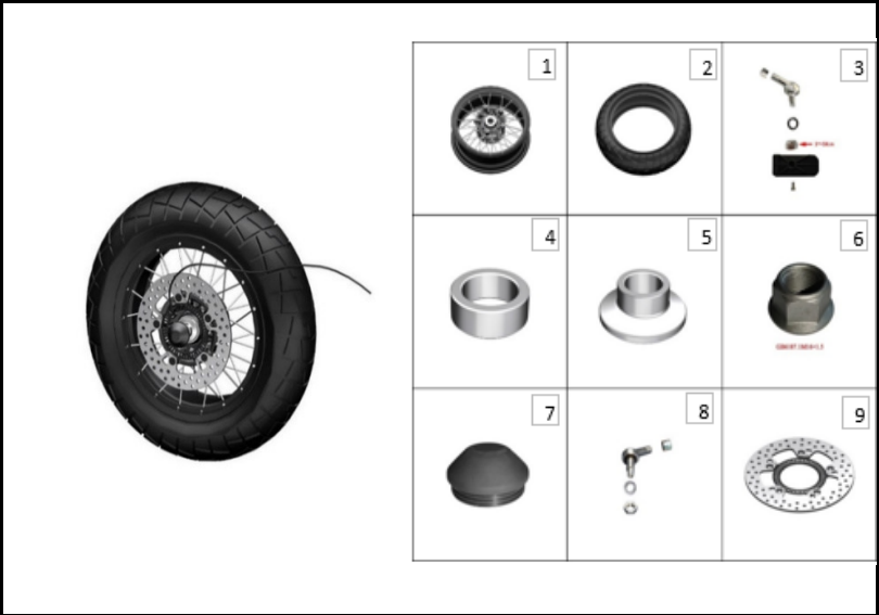
FIGURA N° 85: RUEDA TRASERA
