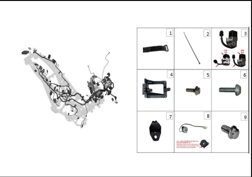
FIGURA N° 95: CERRADURA ELECTRONICA
