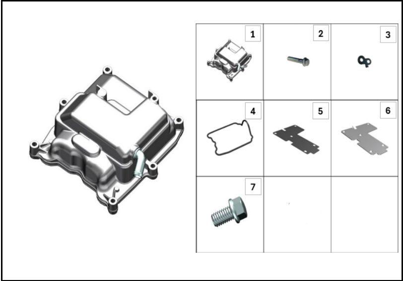
FIGURA N° 1: TAPA CULATA
