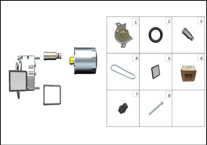
FIGURA N° 27: BOMBA ACEITE
