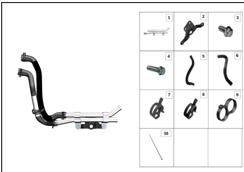
FIGURA N° 121: TUBO REFRIGERANTE
