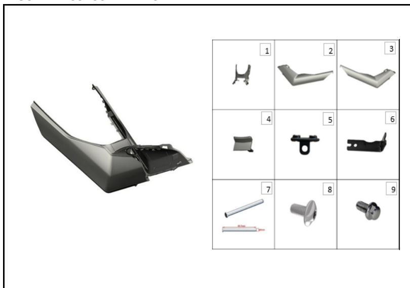
FIGURA N° 53: CUBIERTA CENTRAL
