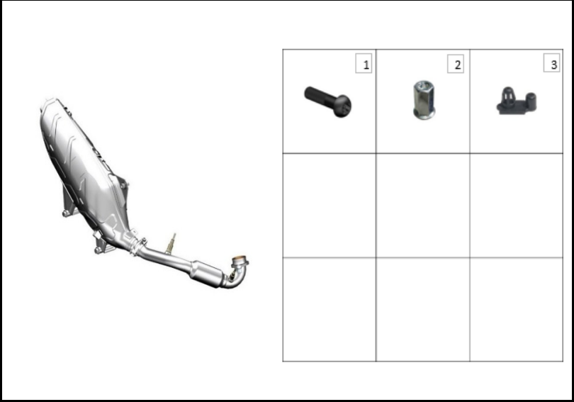
FIGURA N° 110: SILENCIADOR
