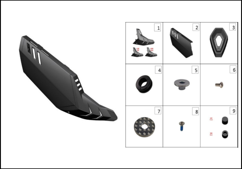
FIGURA N° 111: CUBIERTA SILENCIADOR
