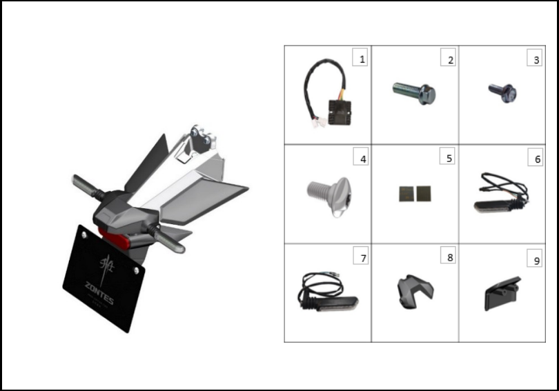
FIGURA N° 59: DIRECCIONAL TRASERA
