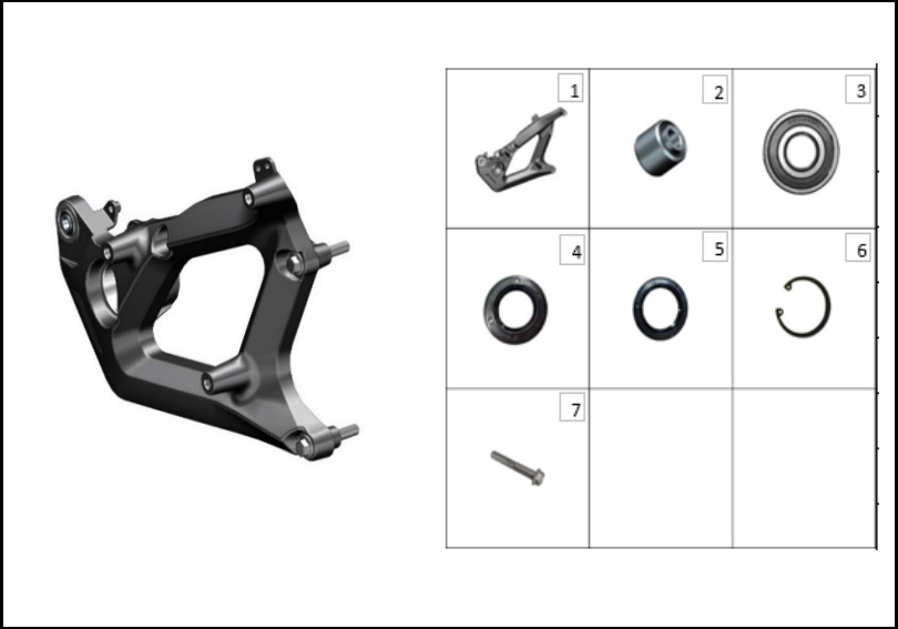
FIGURA N° 88: SOPORTE LATERAL
