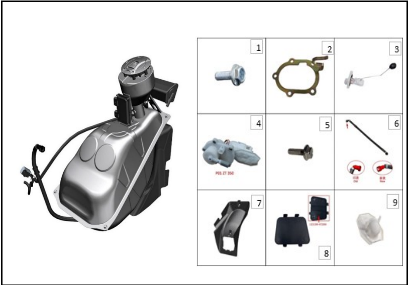
FIGURA N° 100: TANQUE COMBUSTIBLE
