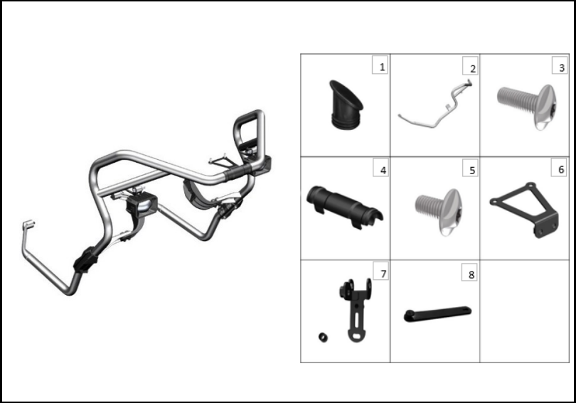
FIGURA N° 69: DEFENSA DERECHA
