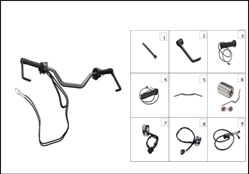
FIGURA N° 70: MANUBRIO
