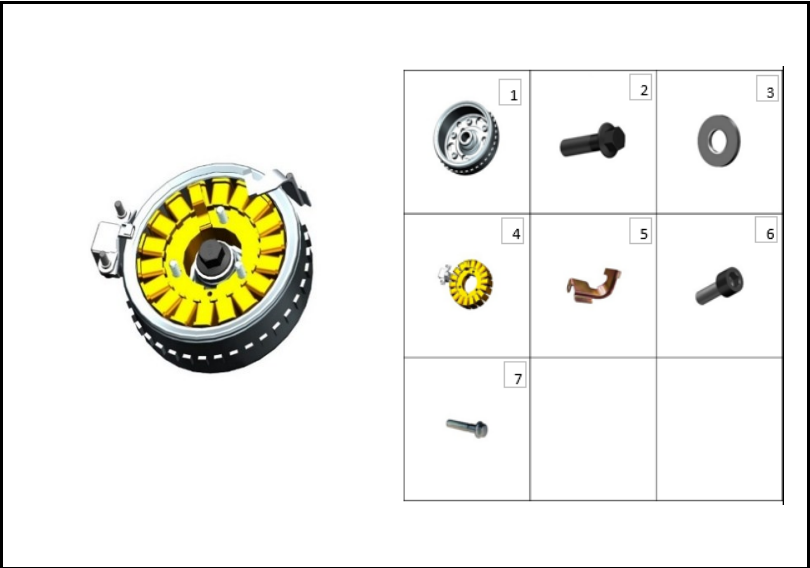
FIGURA N° 25: VOLANTE
