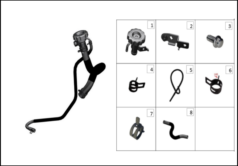
FIGURA N° 119: TAPA RADIADOR
