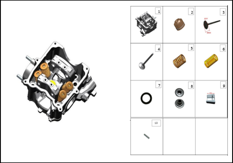
FIGURA N° 3: CULATA
