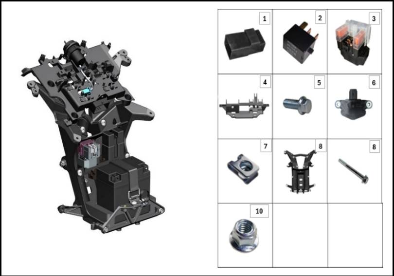
FIGURA N° 93: RELAY ARRANQUE
