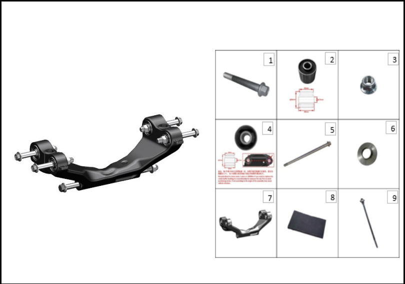
FIGURA N° 102: SOPORTE
