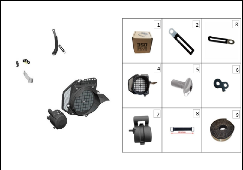
FIGURA N° 106: FILTRO MOTOR
