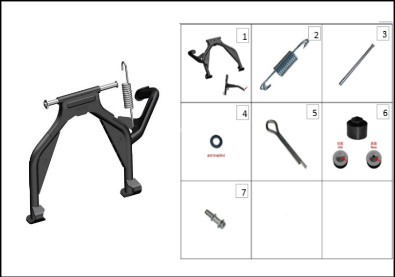
FIGURA N° 109: GATO CENTRAL
