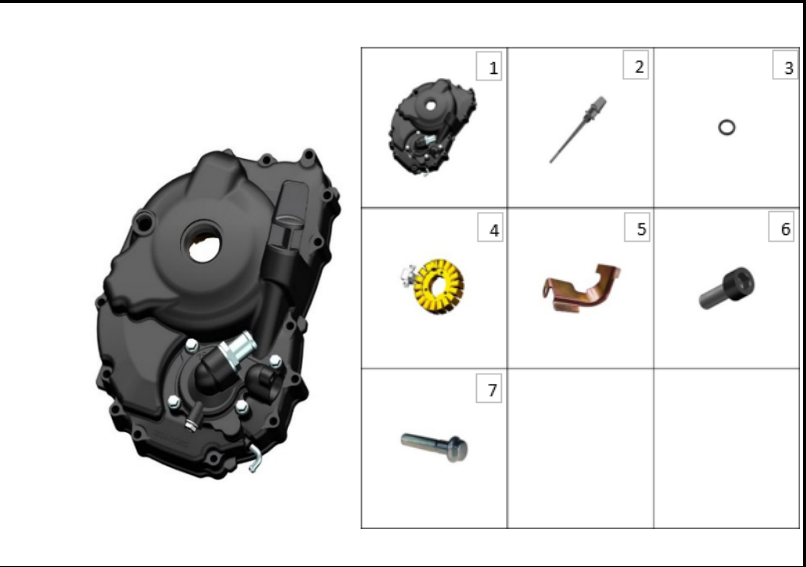
FIGURA N° 21: PLATO BOBINAS
