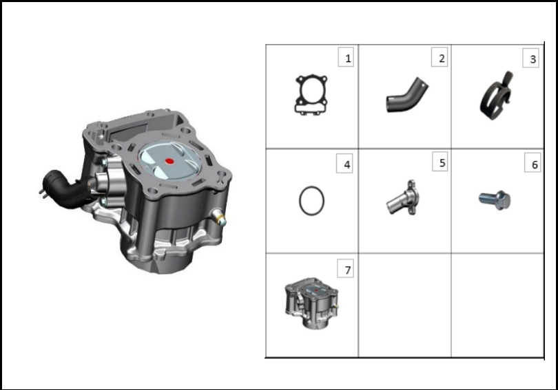
FIGURA N° 4: CILINDRO
