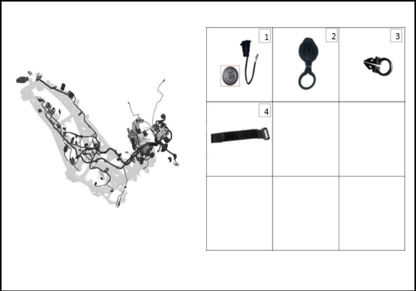
FIGURA N° 99: PUERTO USB
