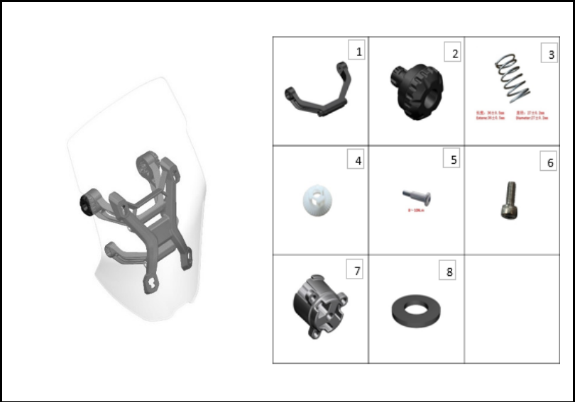
FIGURA N° 29: COMPONENTES VISOR
