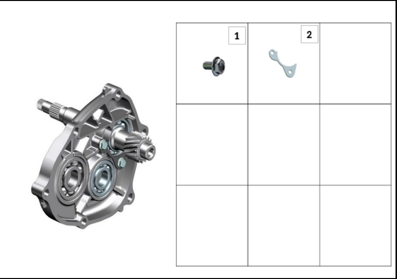
FIGURA N° 16: CUBIERTA TRANSMISION
