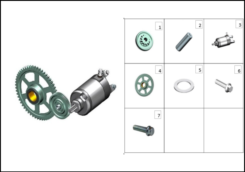
FIGURA N° 24: MOTOR ARRANQUE
