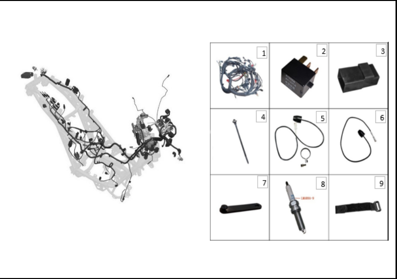
FIGURA N° 94: SISTEMA ELECTRICO
