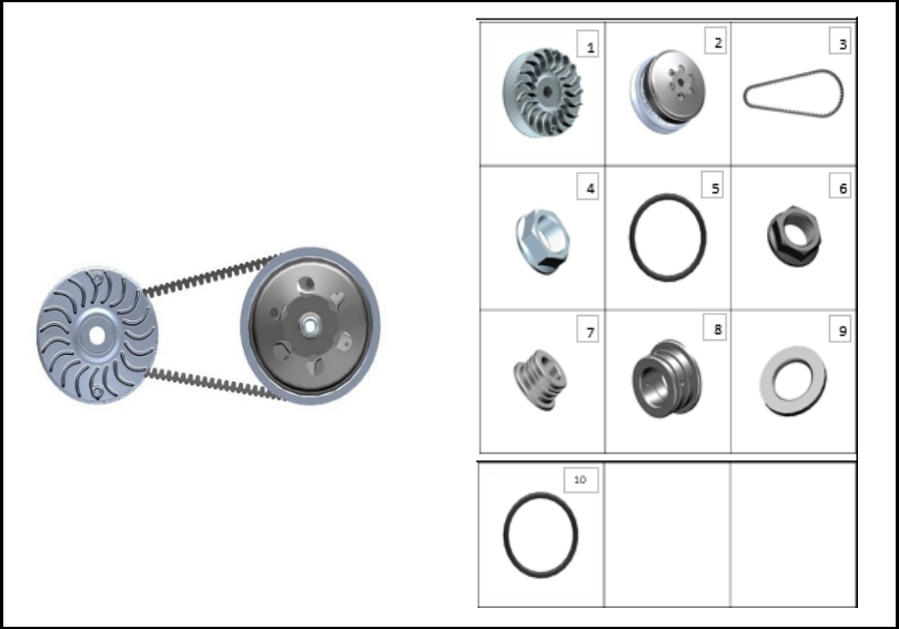
FIGURA N° 6: POLEA CVT
