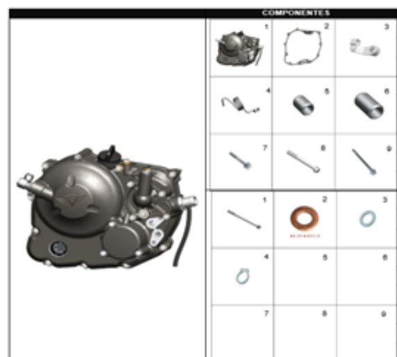
FIGURA N° 124: TAPA CARTER DERECHA
