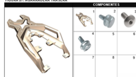
FIGURA 27: AGARRADERA TRASERA
