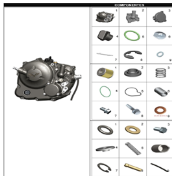
FIGURA N° 125: TAPA CARTER DERECHA
