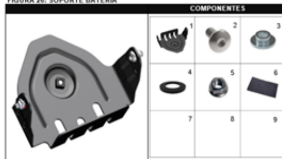
FIGURA 26: SOPORTE BATERÍA
