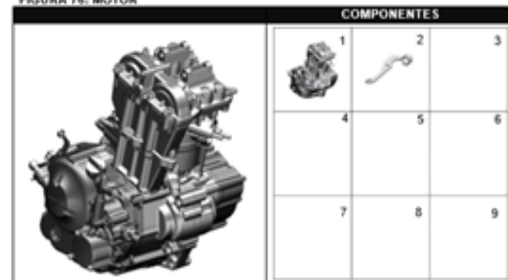
FIGURA 76: MOTOR
