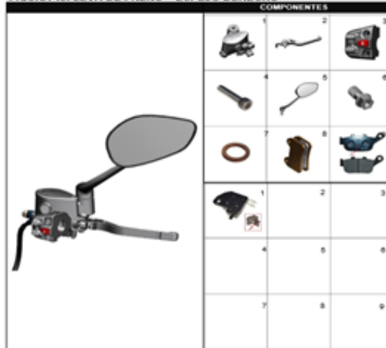
FIGURA 41: LEVA DE FRENO – ESPEJO DERECHO
