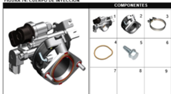
FIGURA 74: CUERPO DE INYECCION
