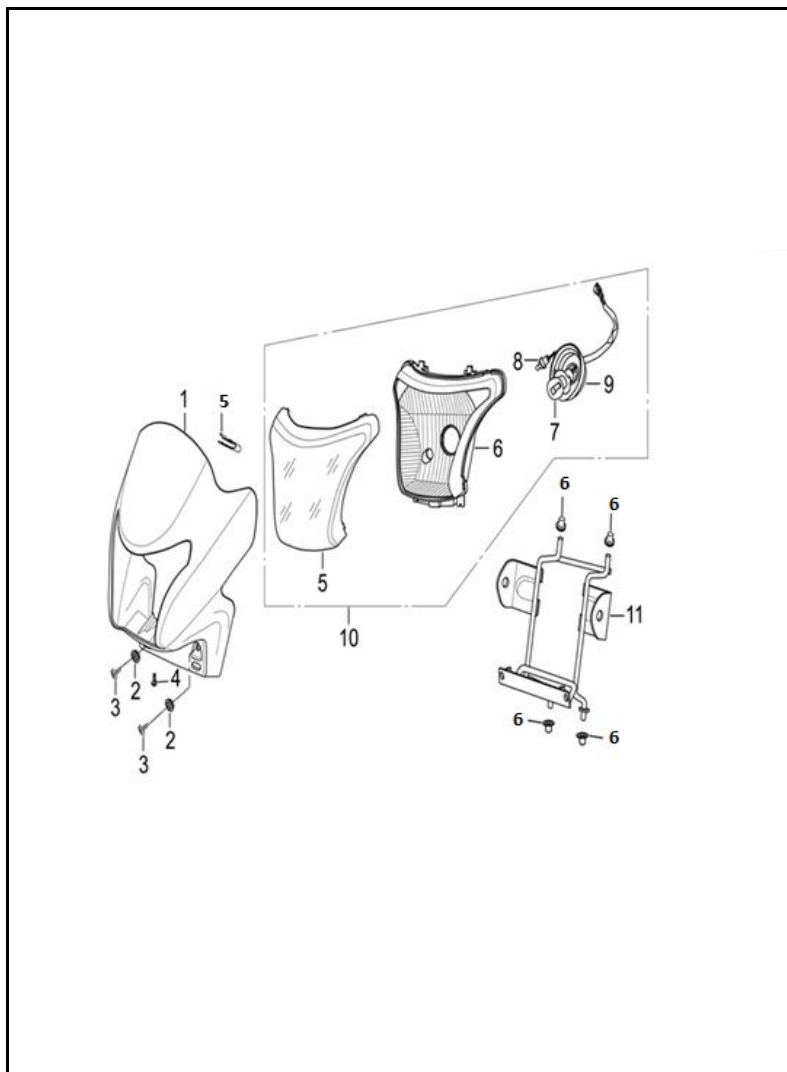
FIGURA N° 22: FAROLA - CARENAGE FAROLA
