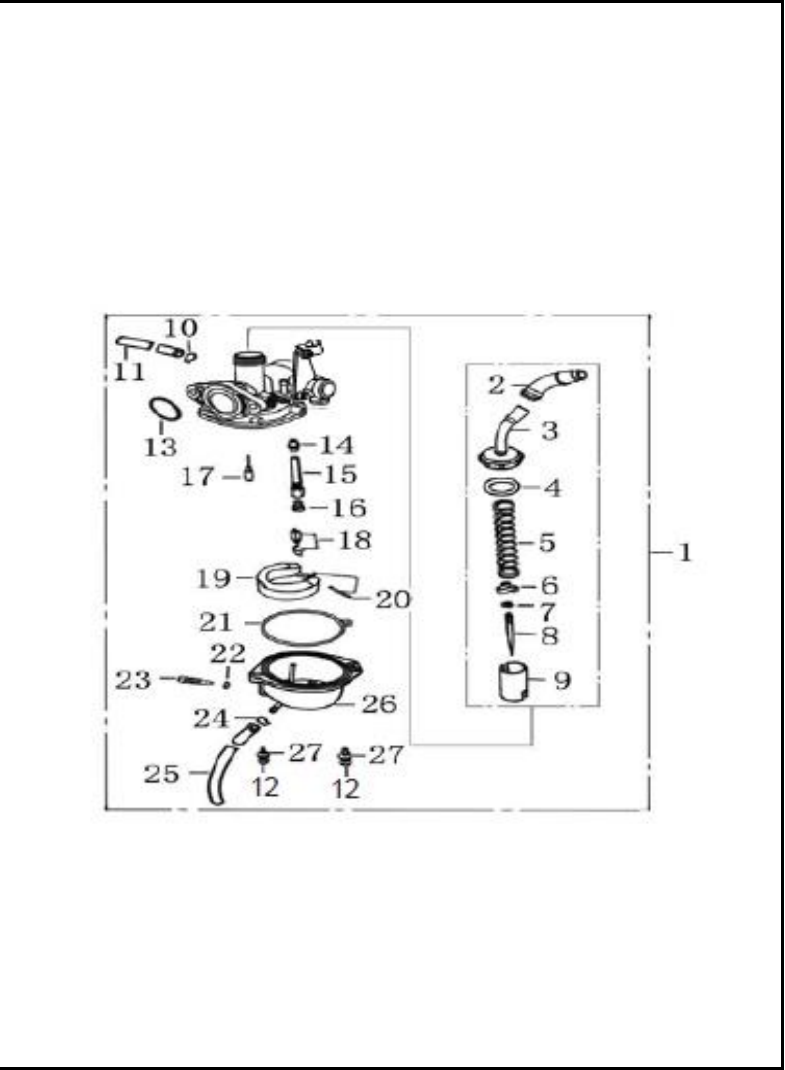
FIGURA N° 14: CARBURADOR (1/2)
