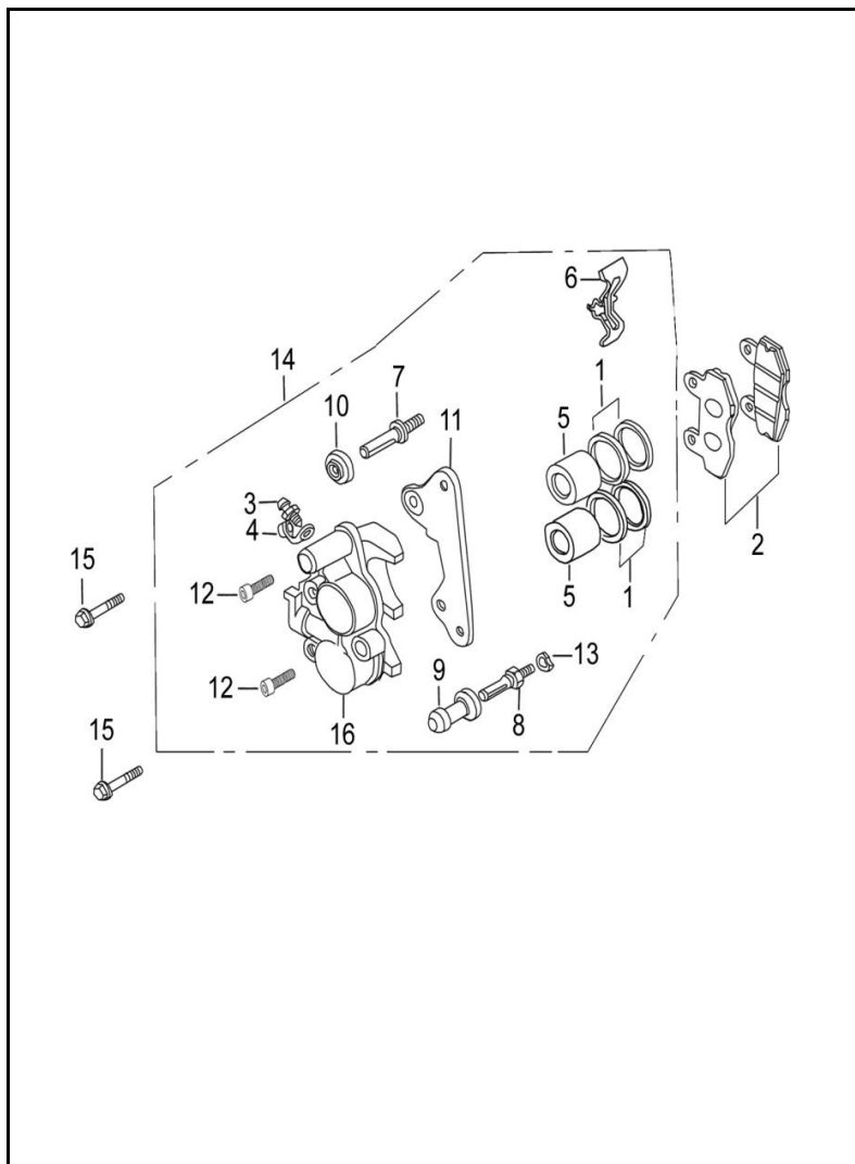
FIGURA N° 27: CALIPER DELANTERO
