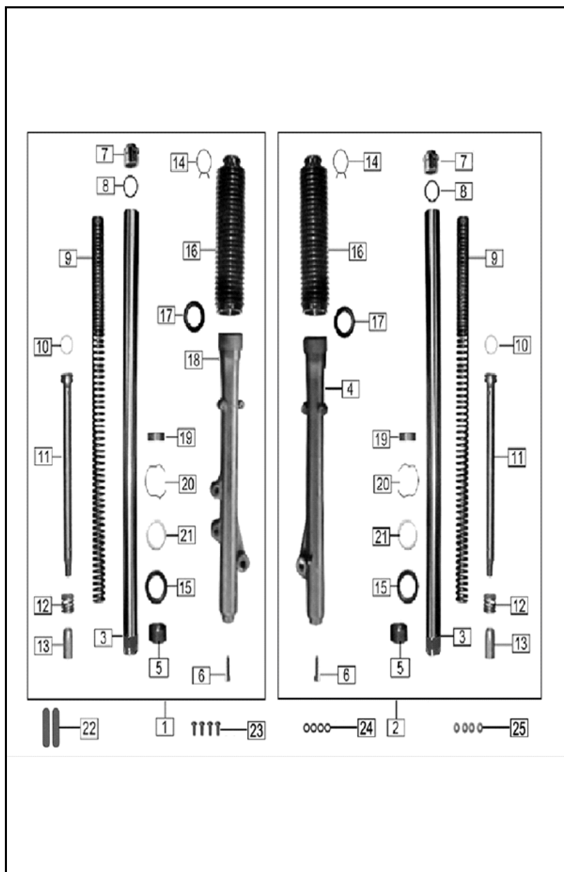
FIGURA N° 23 SUSPENSIÓN DELANTERA
