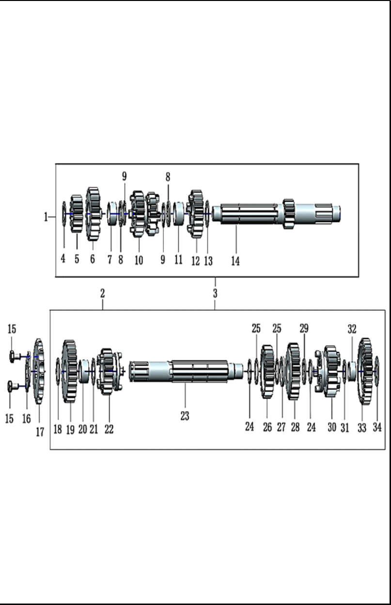
FIGURA N° 8 TRANSMISIÓN (1/2)
