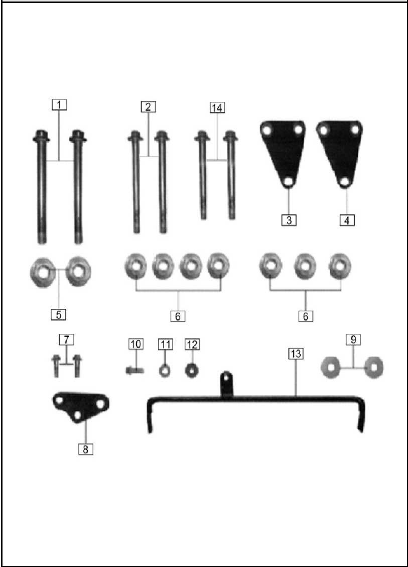
FIGURA N° 45: SOPORTE MOTOR
