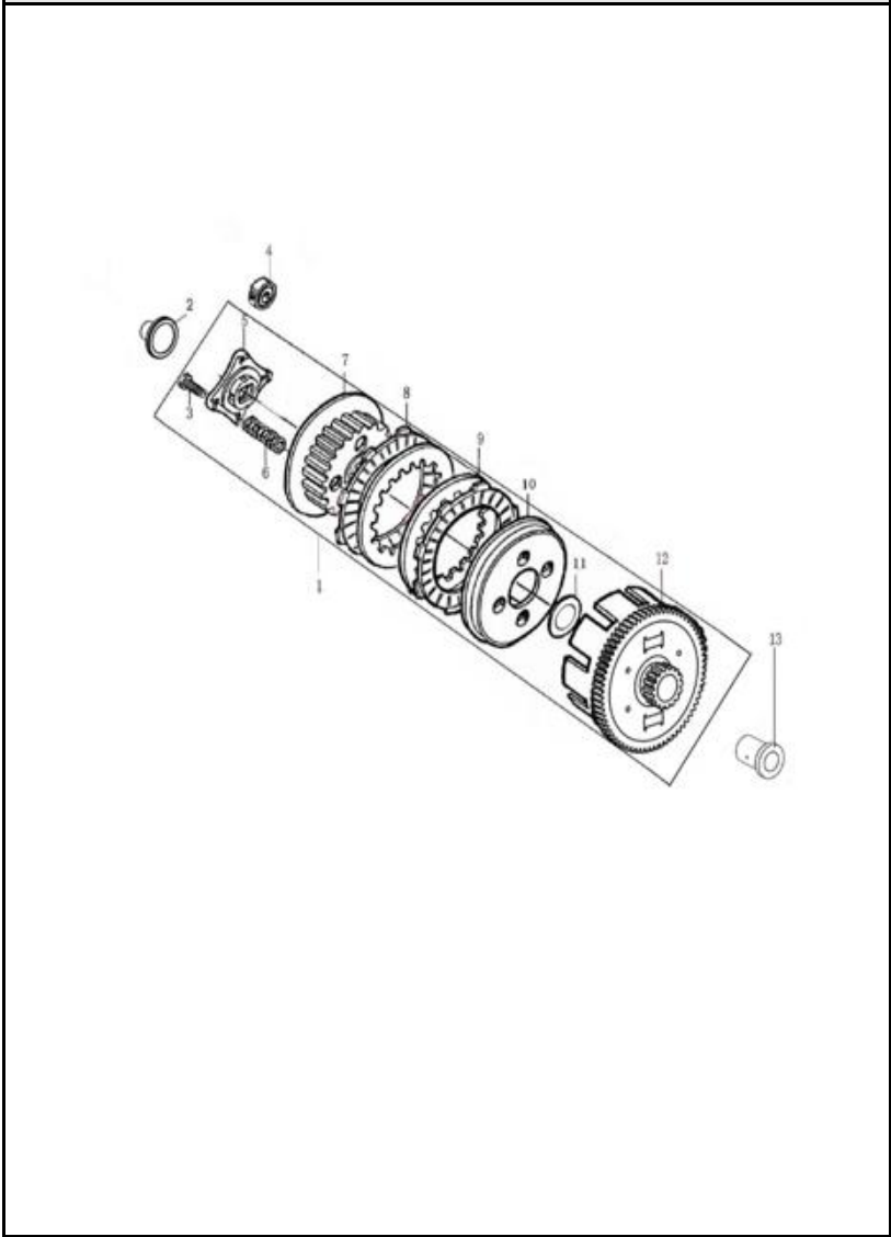
FIGURA N° 4: CLUTCH
