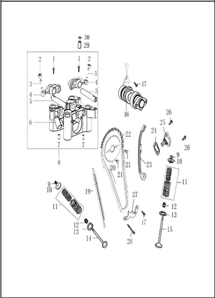
FIGURA N° 2: EJE LEVAS - VALVULAS (1/2)
