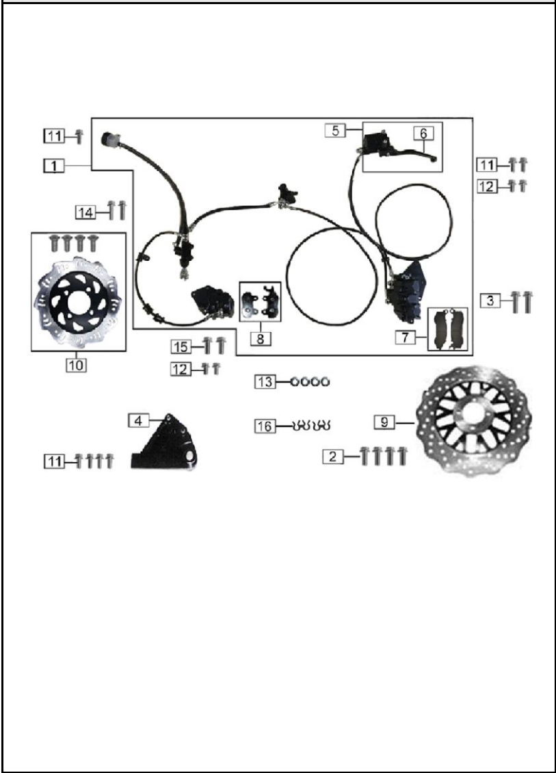
FIGURA N° 35B: BOMBA FRENO CBS
