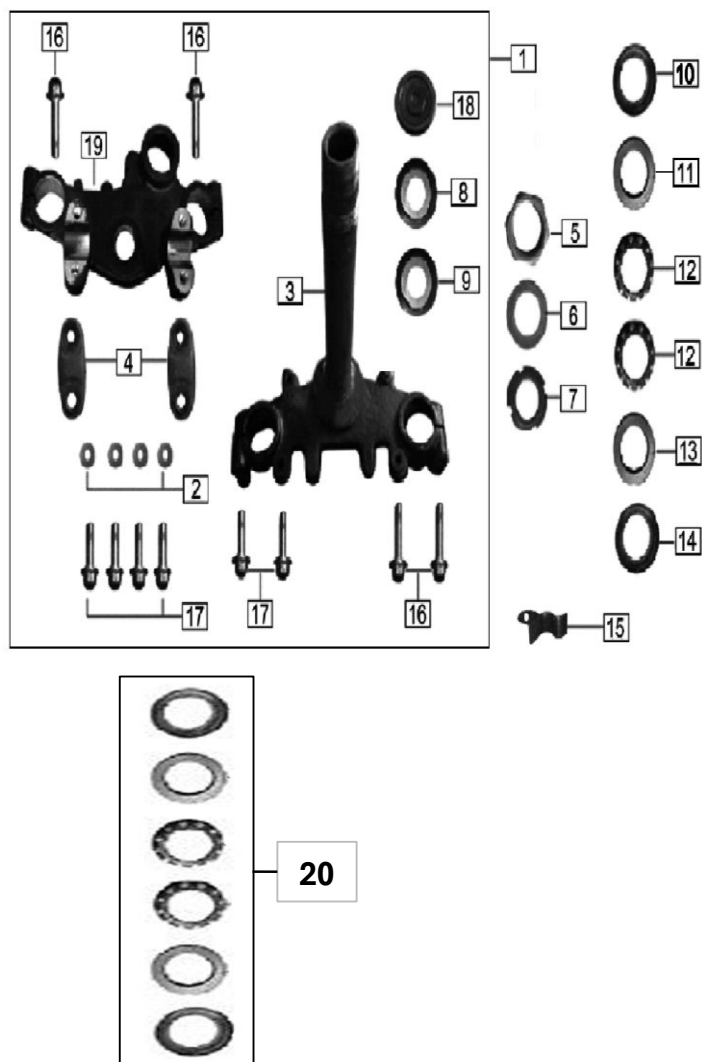
FIGURA N° 31: ESPIGA CENTRAL - CABEZA ESPIGA
