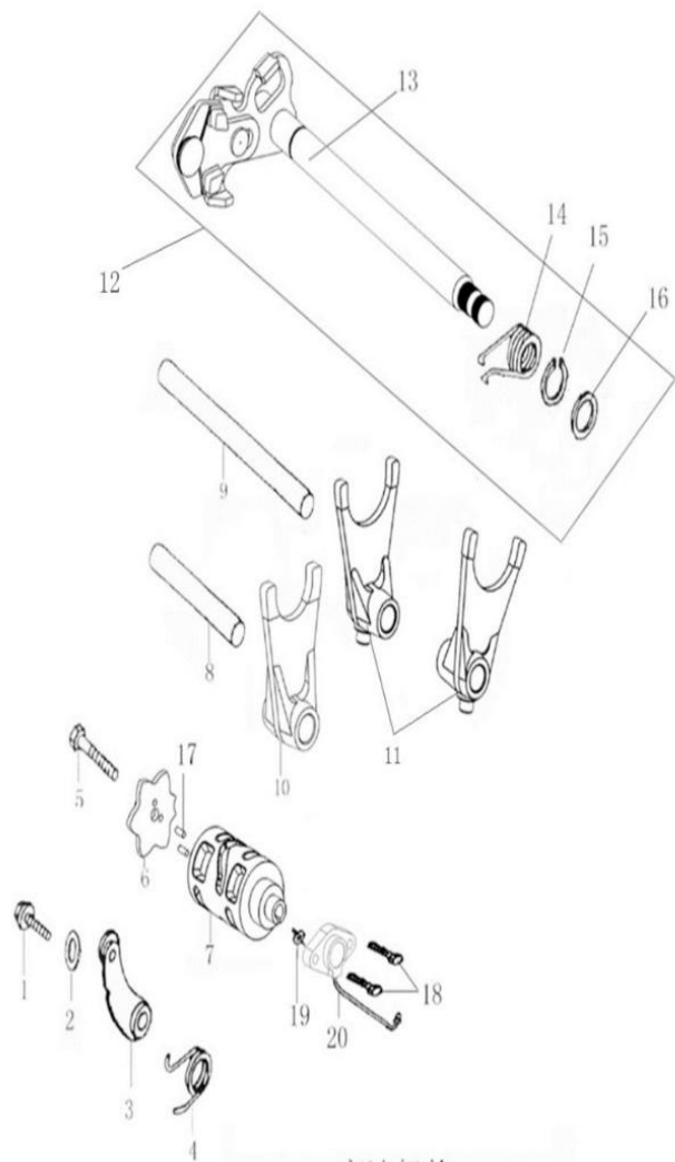
FIGURA N° 9: EJE CAMBIOS - EJE SELECTOR CAMBIOS
