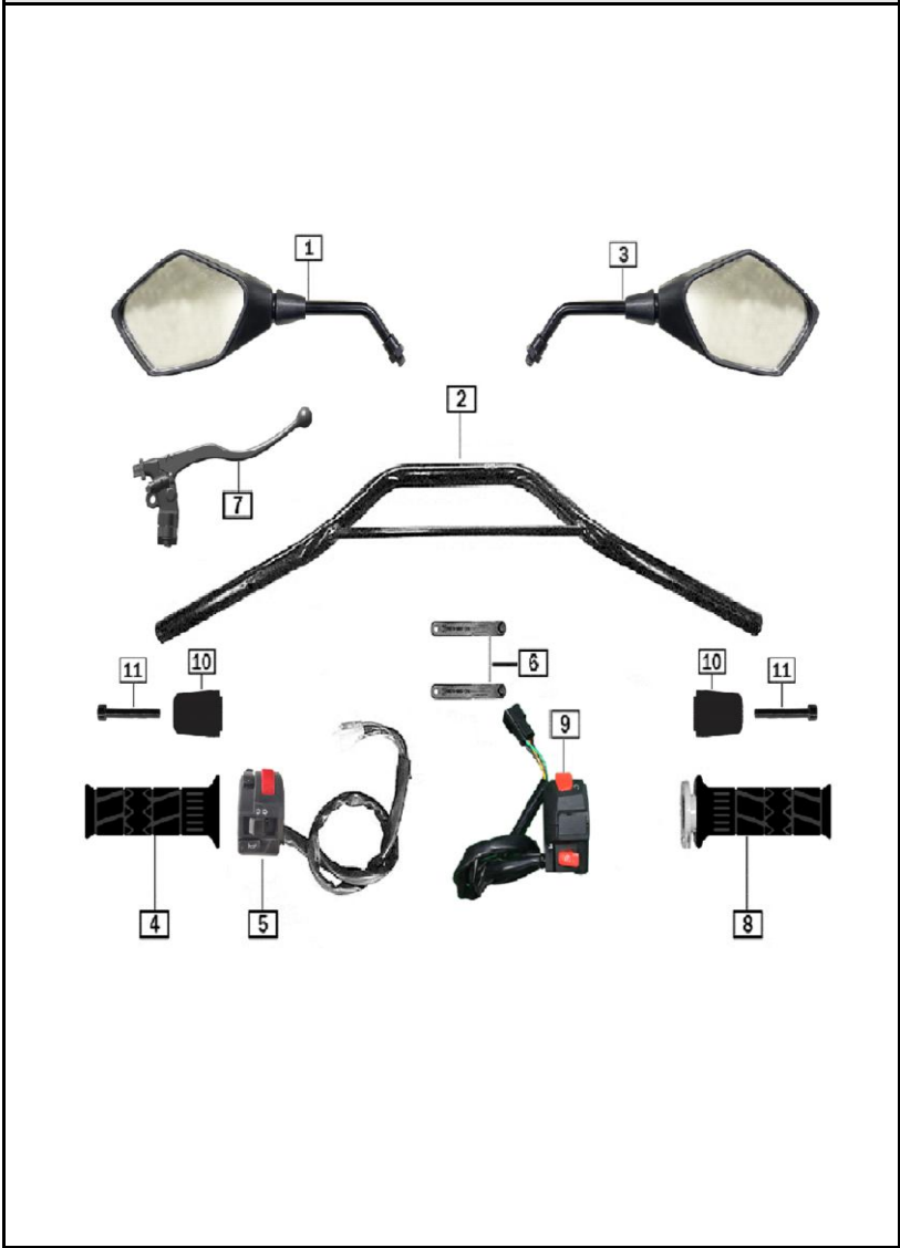
FIGURA N° 18: MANUBRIO - ESPEJOS
