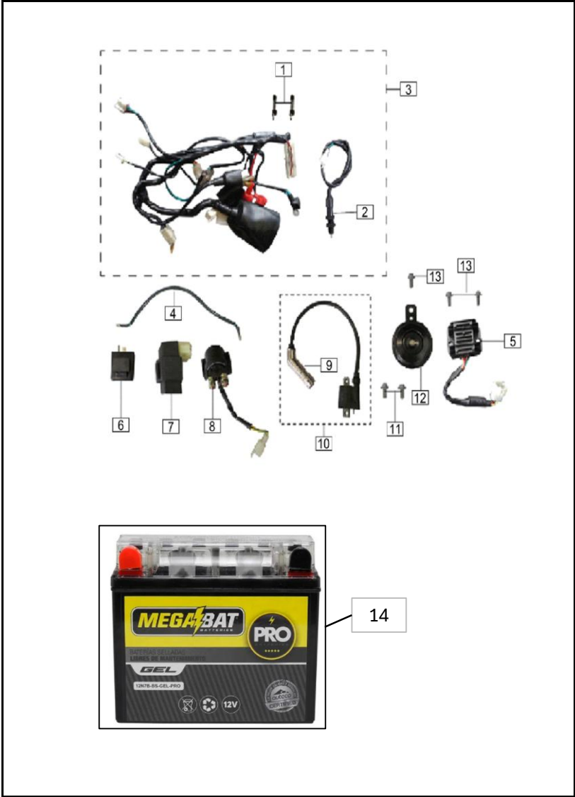
FIGURA N° 22: SISTEMA ELECTRICO
