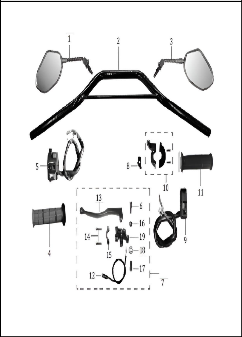
FIGURA N° 19: MANUBRIO - ESPEJOS CAMO PRO
