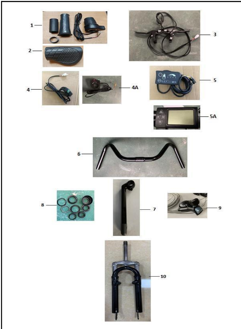
FIGURA N° 1: MANUBRIO - SUSPENSIÓN FRONTAL
