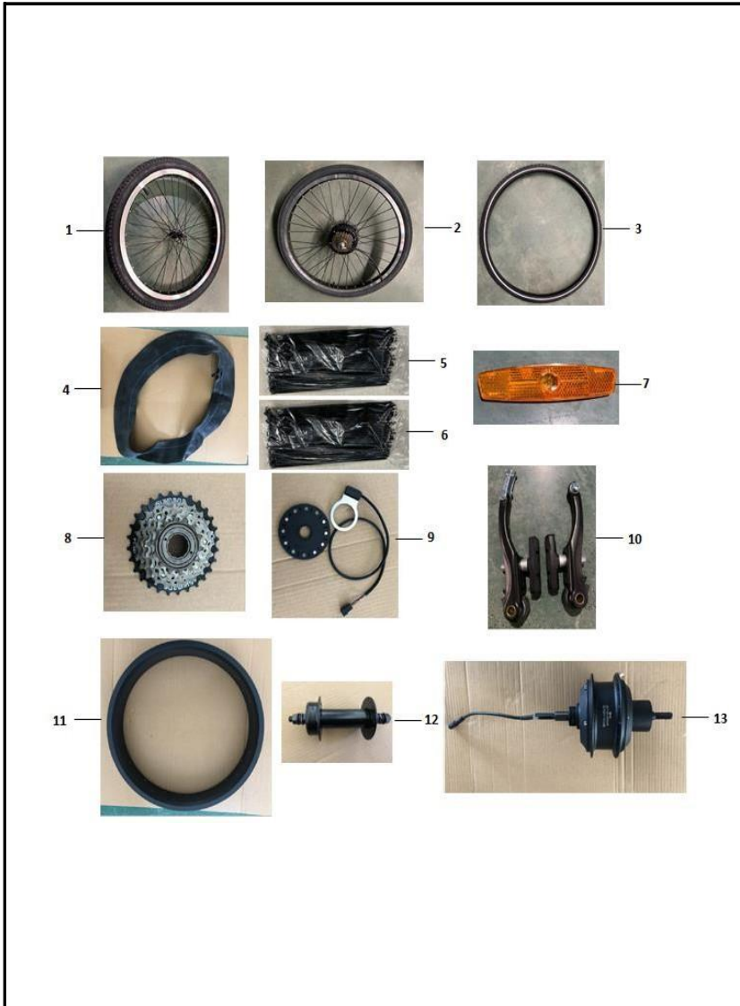
FIGURA N° 2: RUEDA DELANTERA - RUEDA TRASERA
