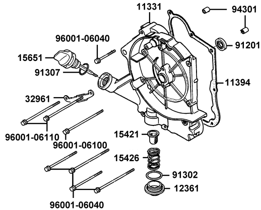
E04: CUBIERTA MOTOR DERECHA
