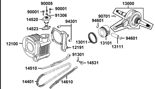
E03: CILINDRO - PISTÓN - CIGUEÑAL
