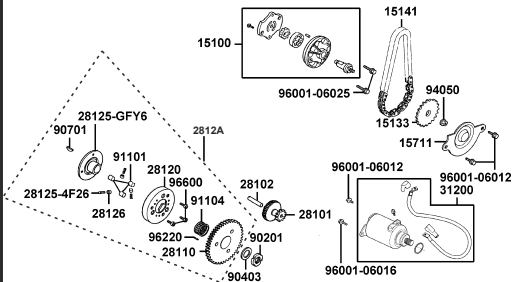
E06: MOTOR DE ARRANQUE - BOMBA DE ACEITE
