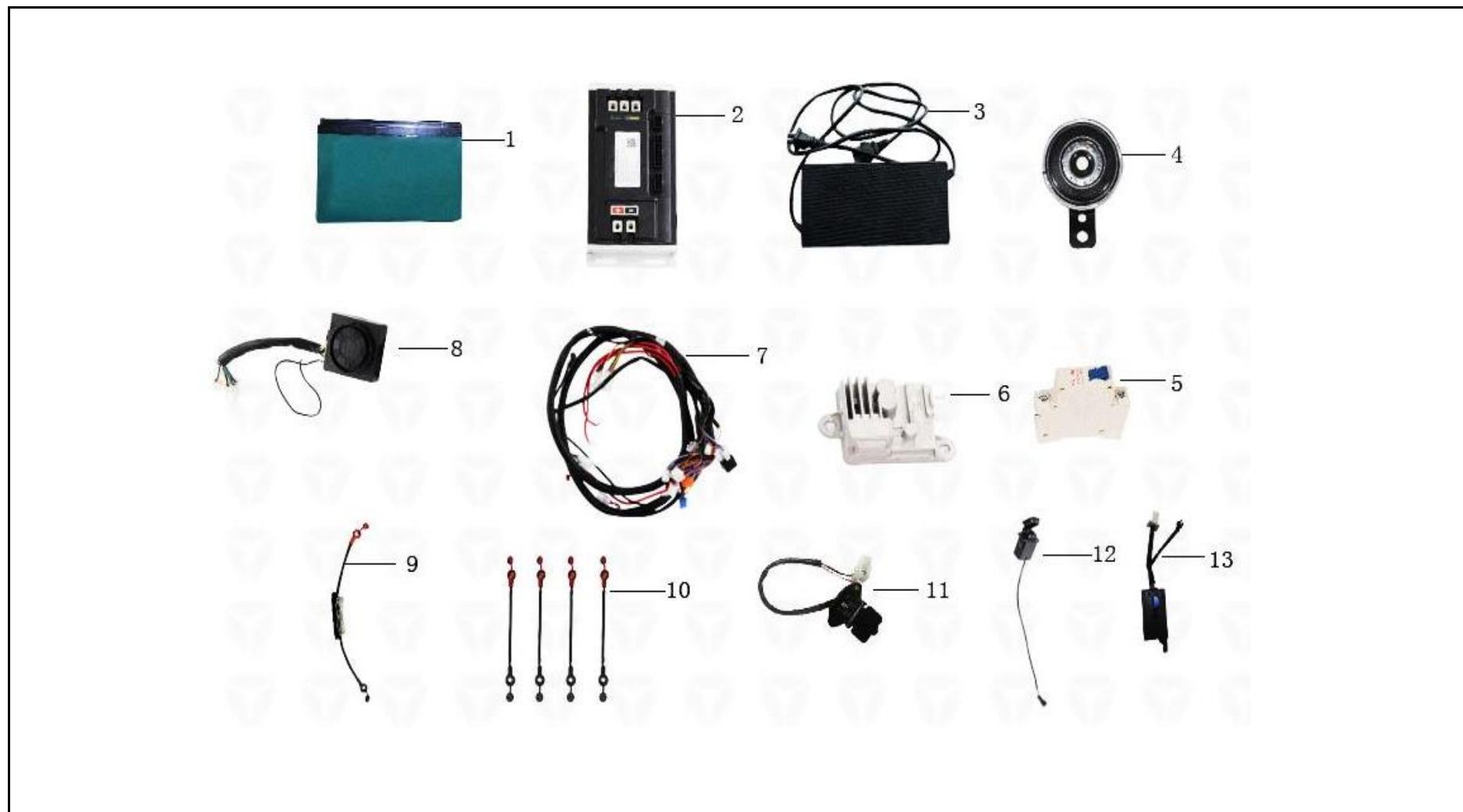
FIGURA N° 7: SISTEMA ELÉCTRICO
