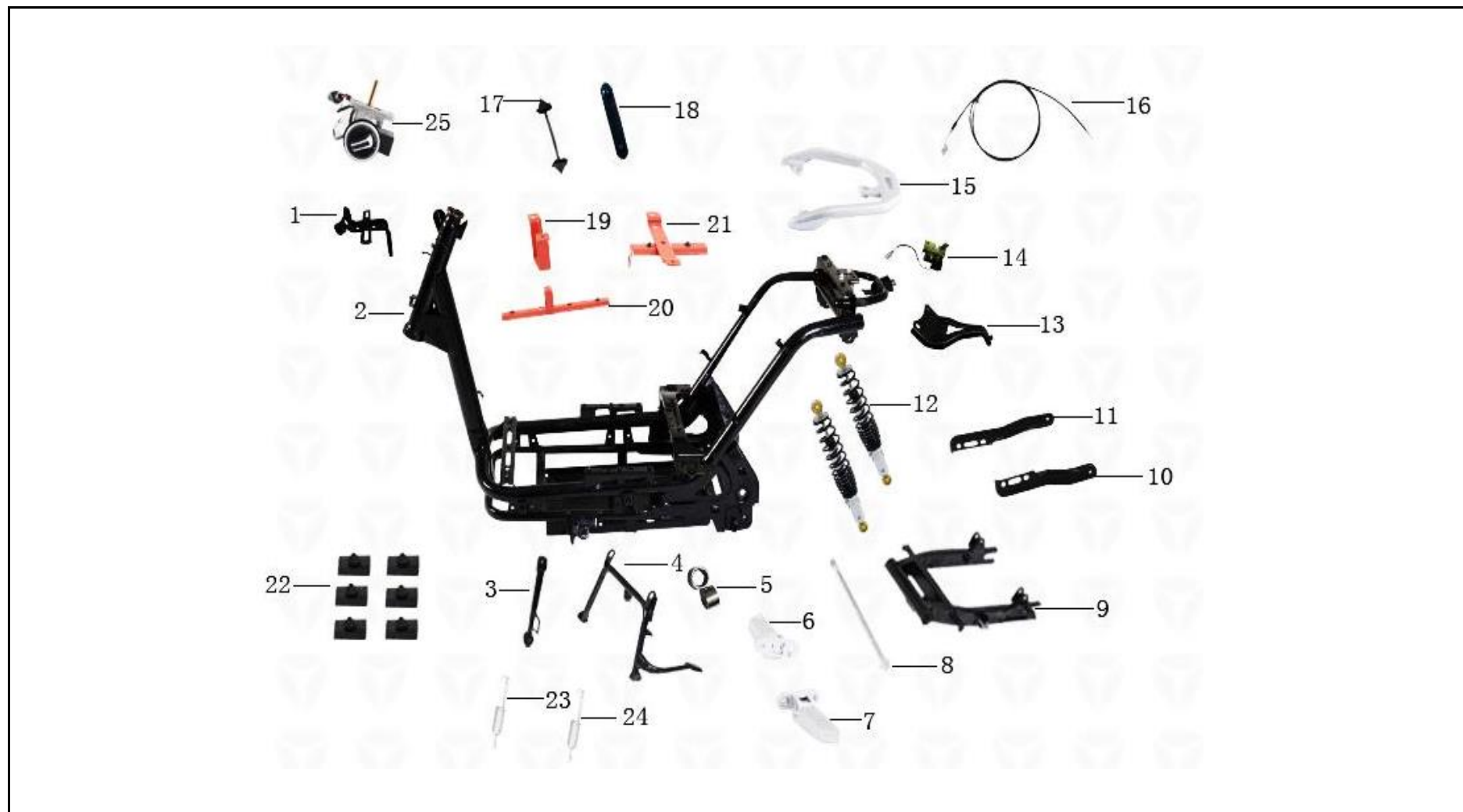
FIGURA N° 4: PARTES DEL CHASIS
