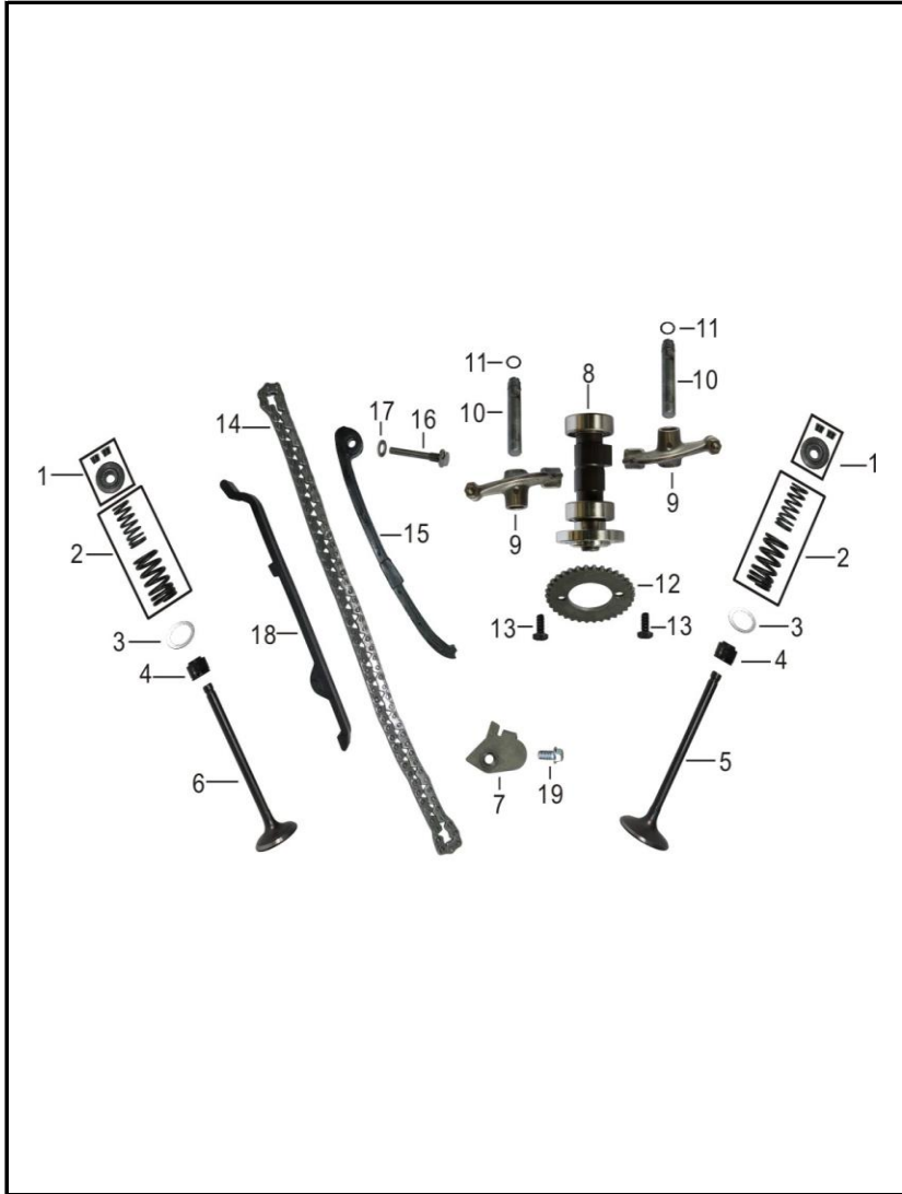
FIGURA N° 3: COMPONENTES CULATA
