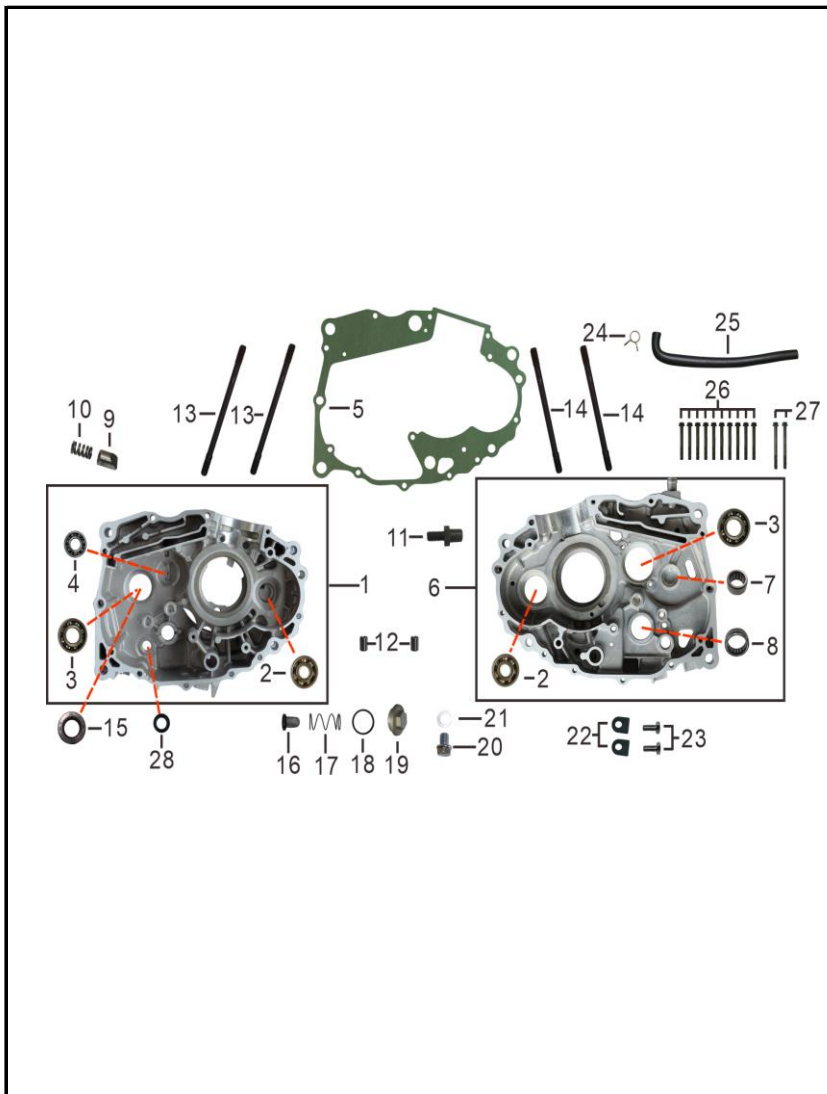
FIGURA N° 4: CARCASAS MOTOR (1/2)
