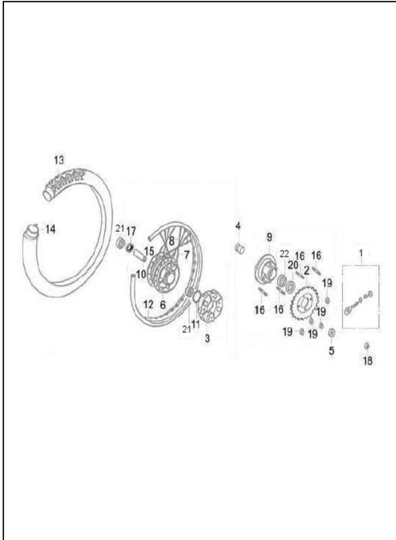
FIGURA N° 28: RUEDA TRASERA (RIN DE RADIOS)
