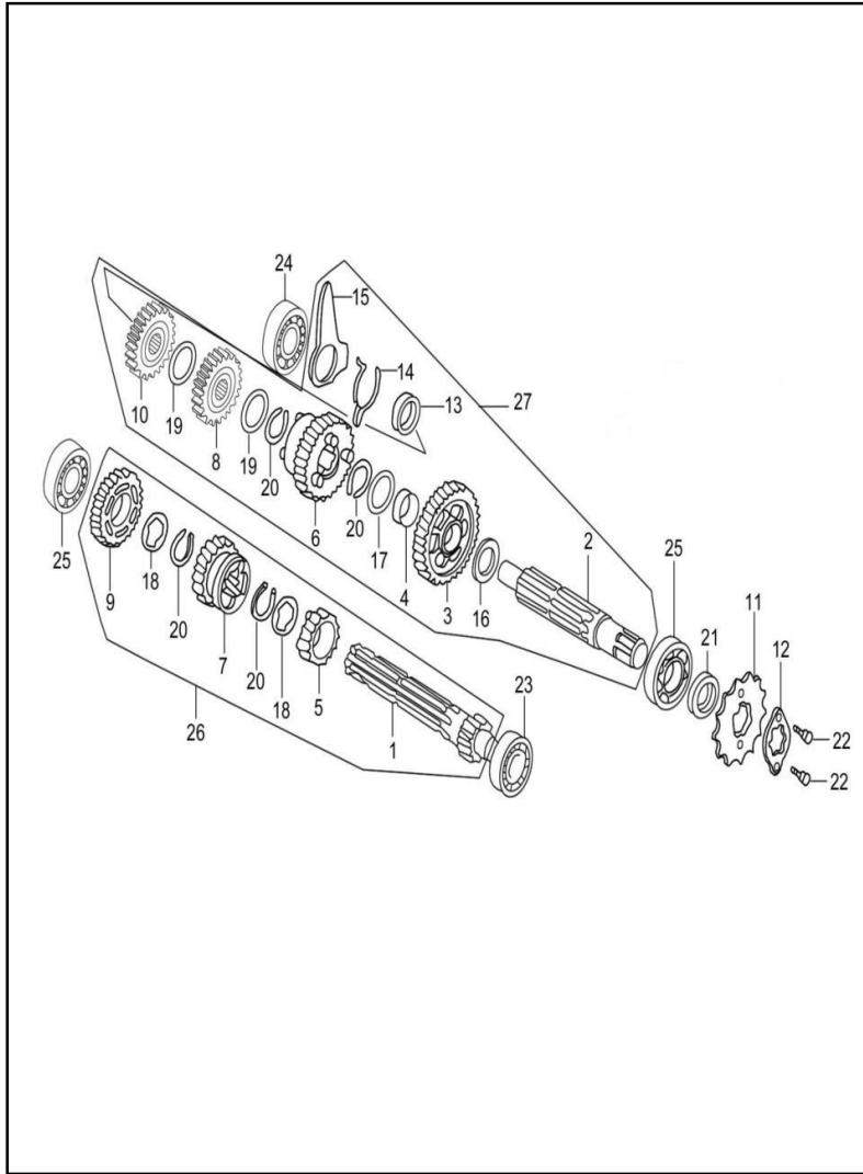
FIGURA N° 14: TRANSMISION
