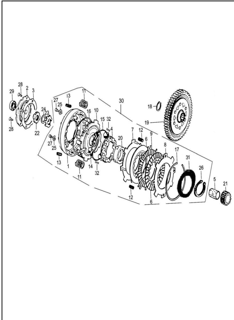
FIGURA N° 7: CLUTCH (7/2)
