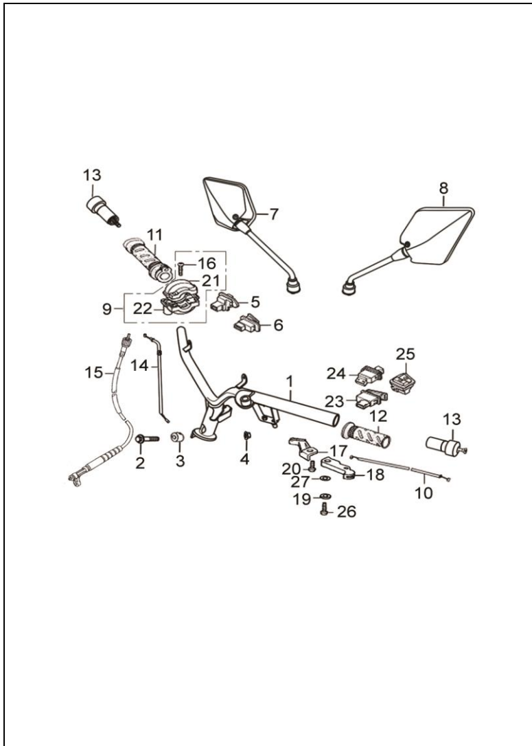
FIGURA N° 20: MANUBRIO - ESPEJOS ONE MP SILVER
