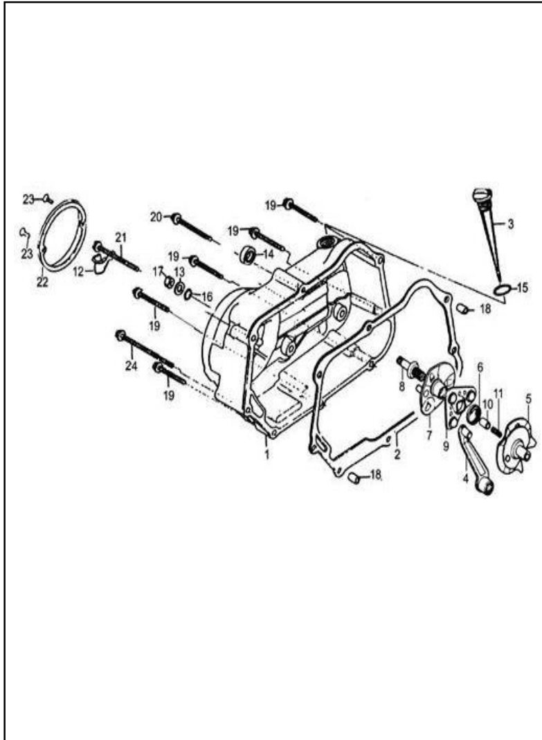
FIGURA N° 6: CUBIERTA CLUTCH
