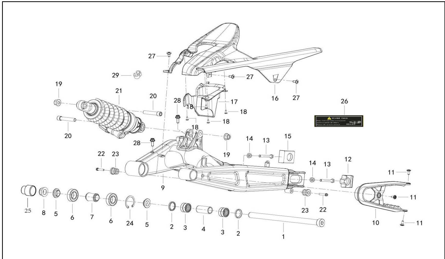
FIGURA N° 22: SUSPENSIÓN TRASERA
