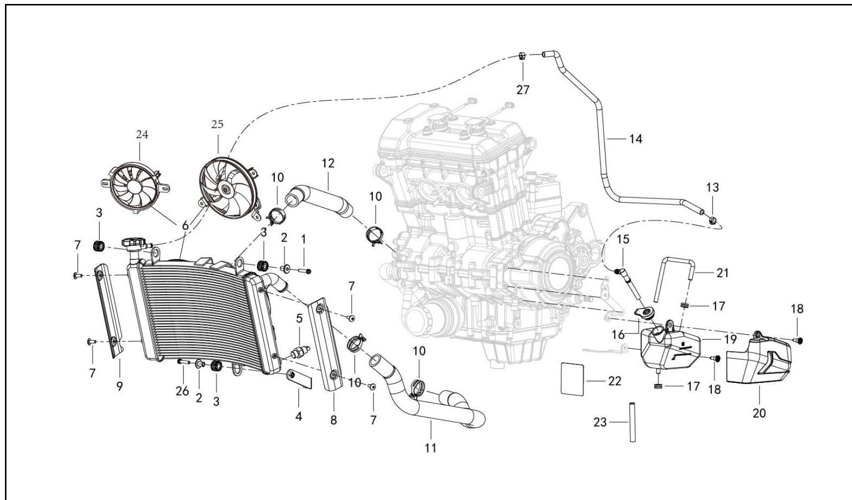
FIGURA N° 35: RADIADOR
