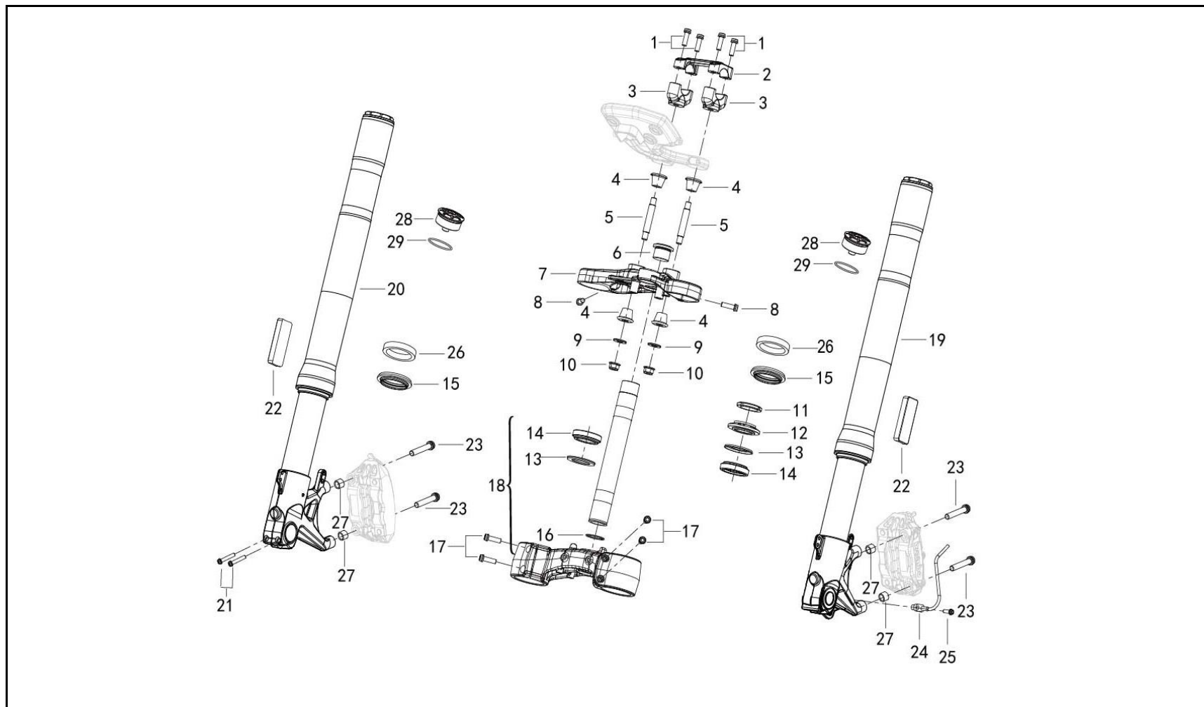
FIGURA N° 17: SUSPENSIÓN DELANTERA
