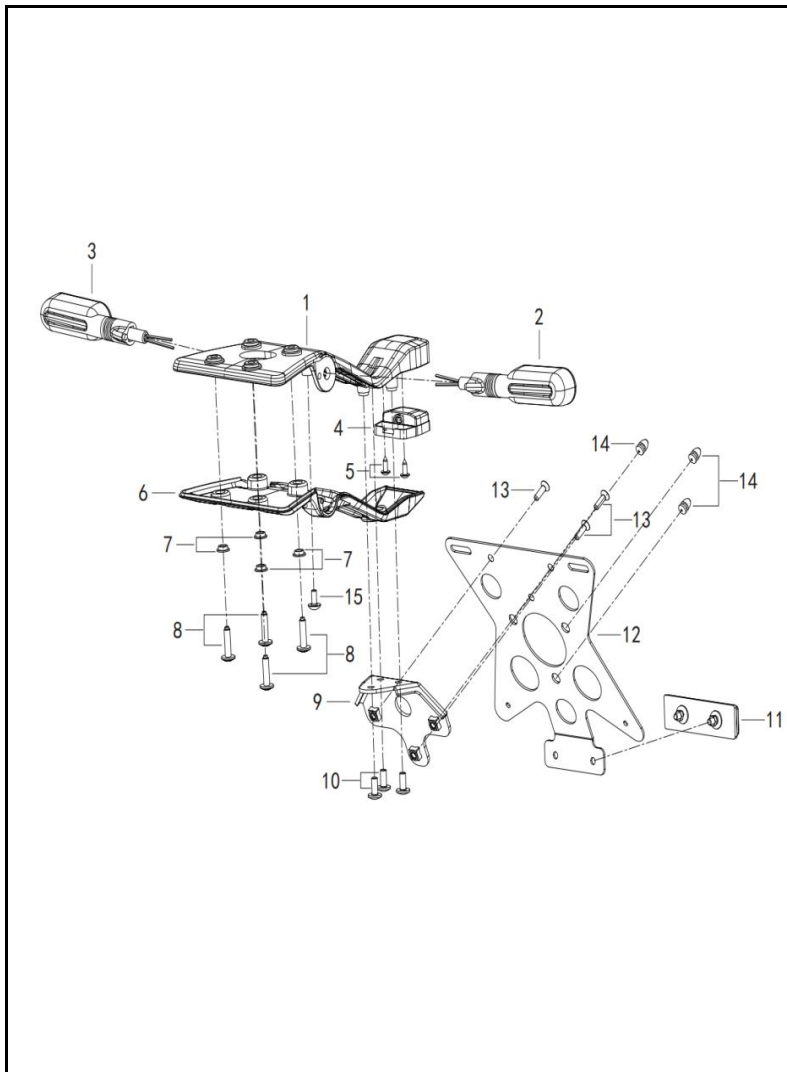
FIGURA N° 34: DIRECCIONALES TRASERAS
