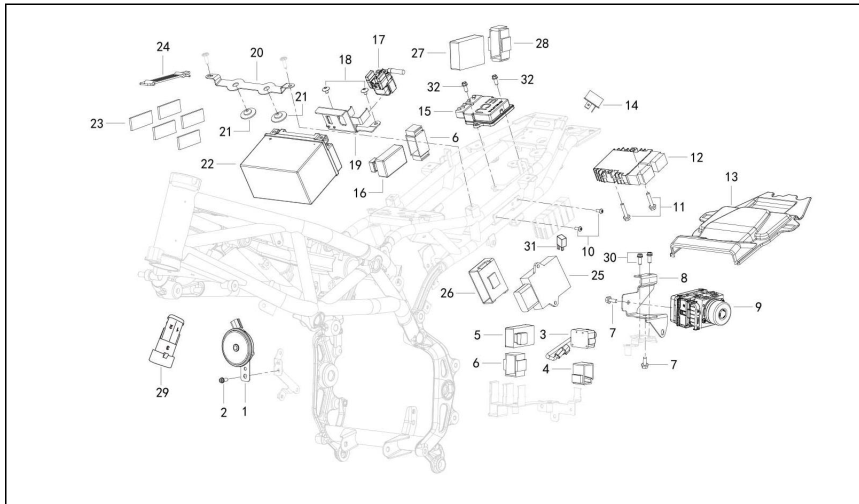
FIGURA N° 36: PARTES ELÉCTRICAS
