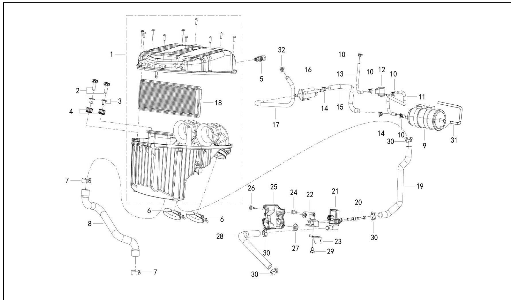
FIGURA N° 21: CAJA FILTRO DE AIRE
