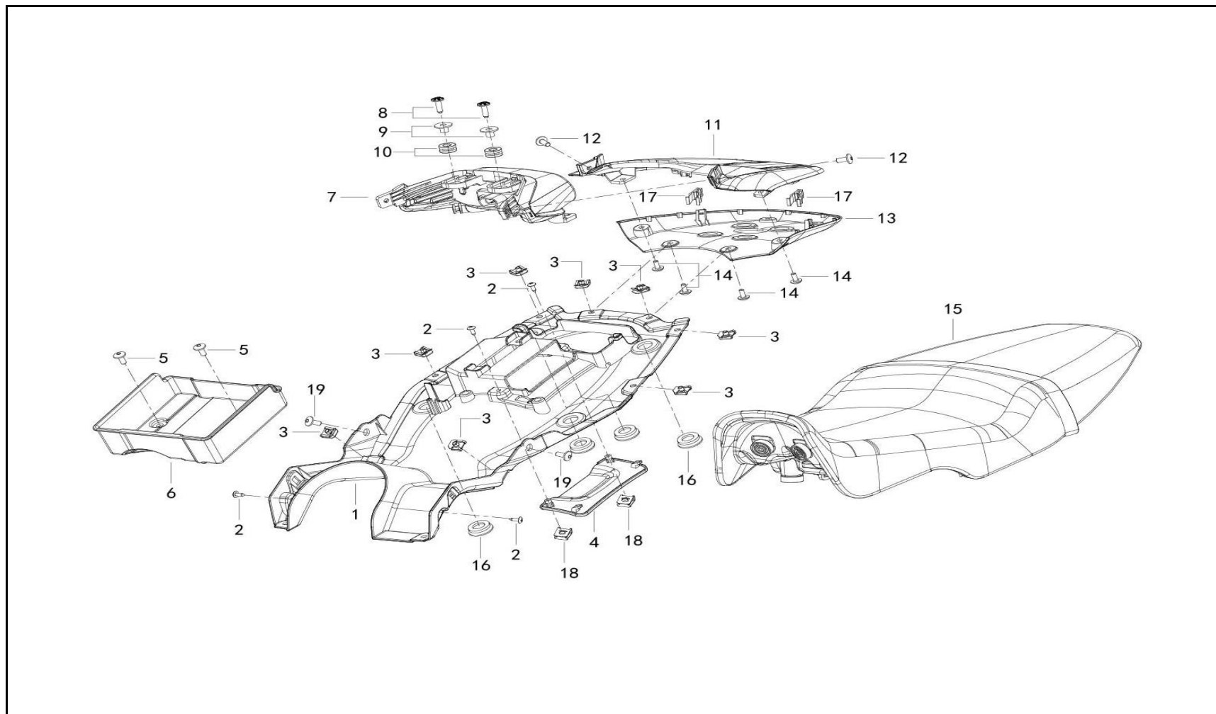
FIGURA N° 33: GUARDABARRO TRASERO - SILLÍN
