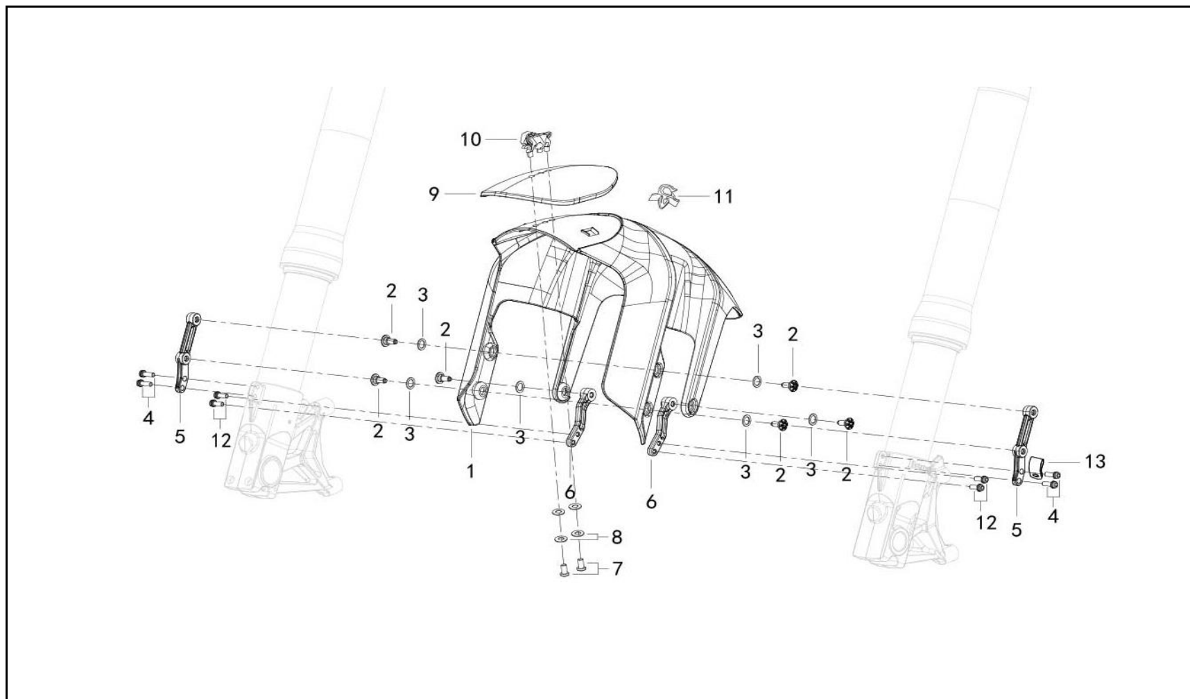
FIGURA N° 32: GUARDABARRO DELANTERO
