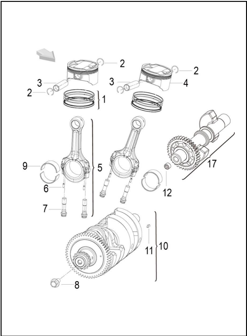
FIGURA N° 5: CIGÜEÑAL - PISTON
