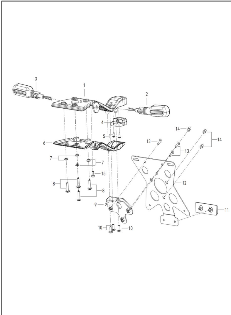
FIGURA N° 35: DIRECCIONALES TRASERAS
