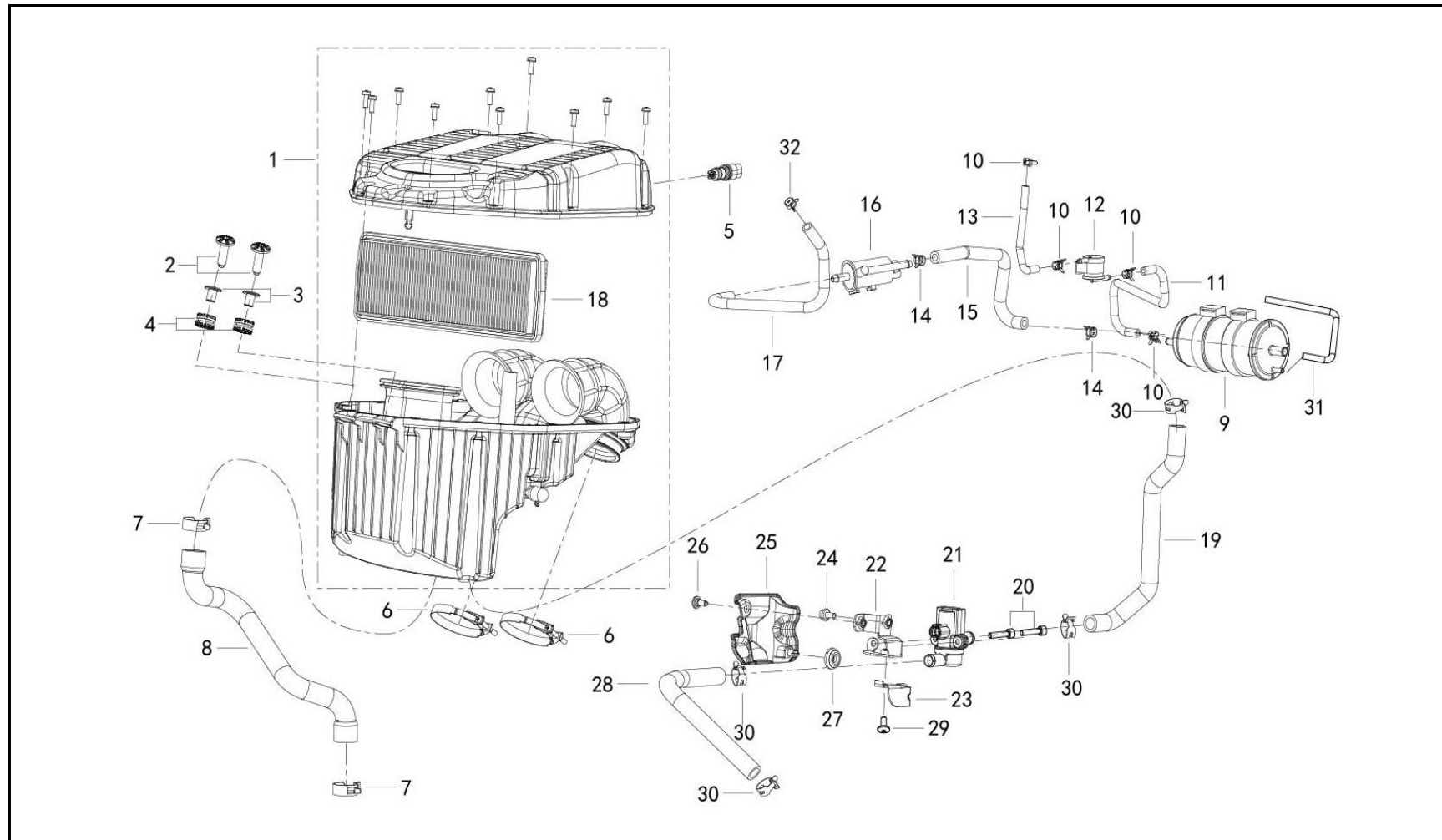
FIGURA N° 21: CAJA FILTRO DE AIRE
