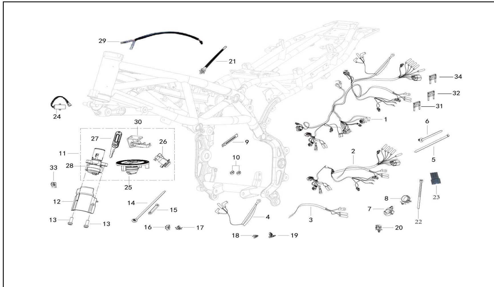
FIGURA N° 39: CUERPO INYECCIÓN
