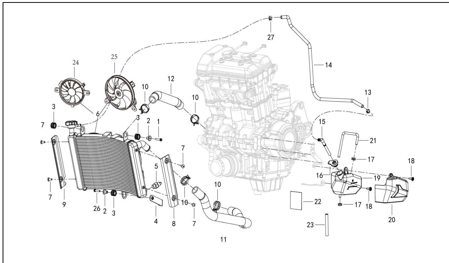
FIGURA N° 36: RADIADOR
