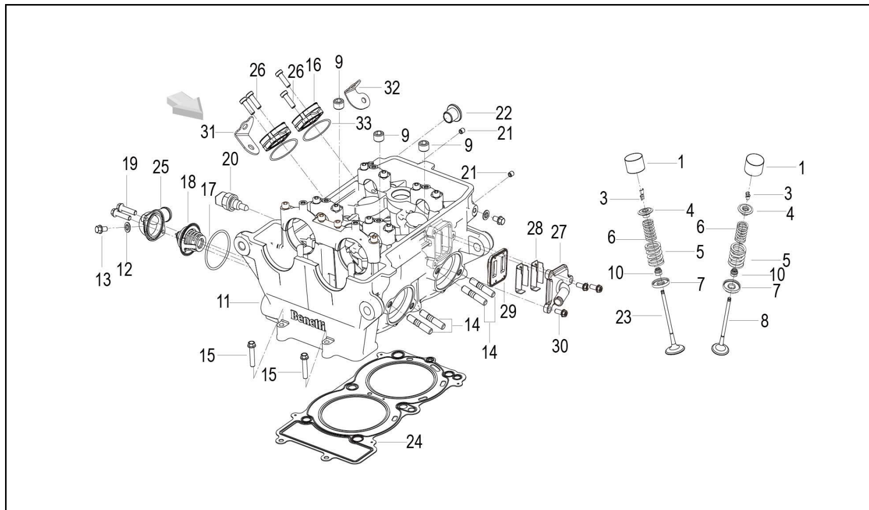
FIGURA N° 2: CULATA
