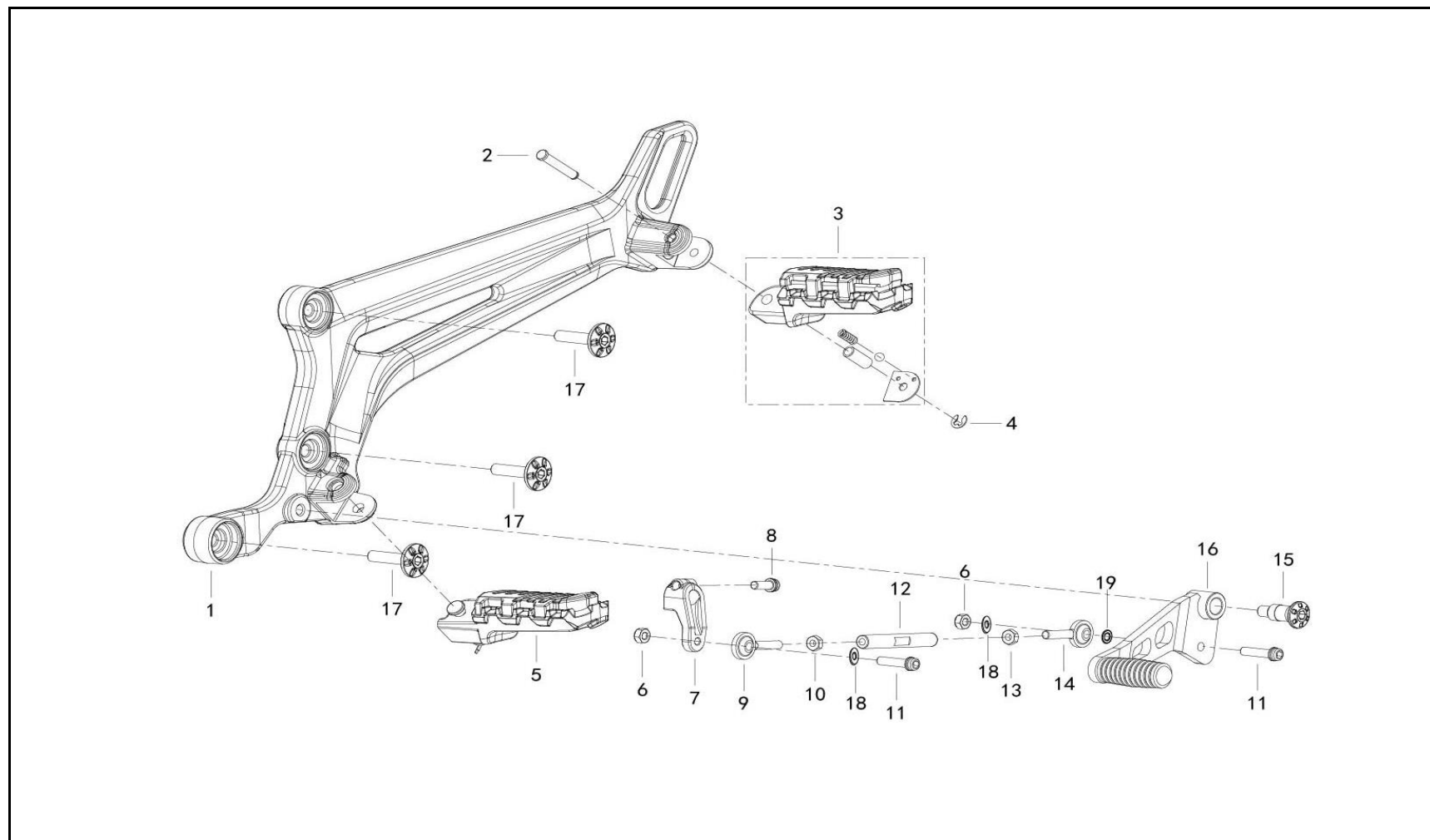
FIGURA N° 28: SOPORTE REPOSAPIE TRASERO-DELANTERO IZQUIERDO
