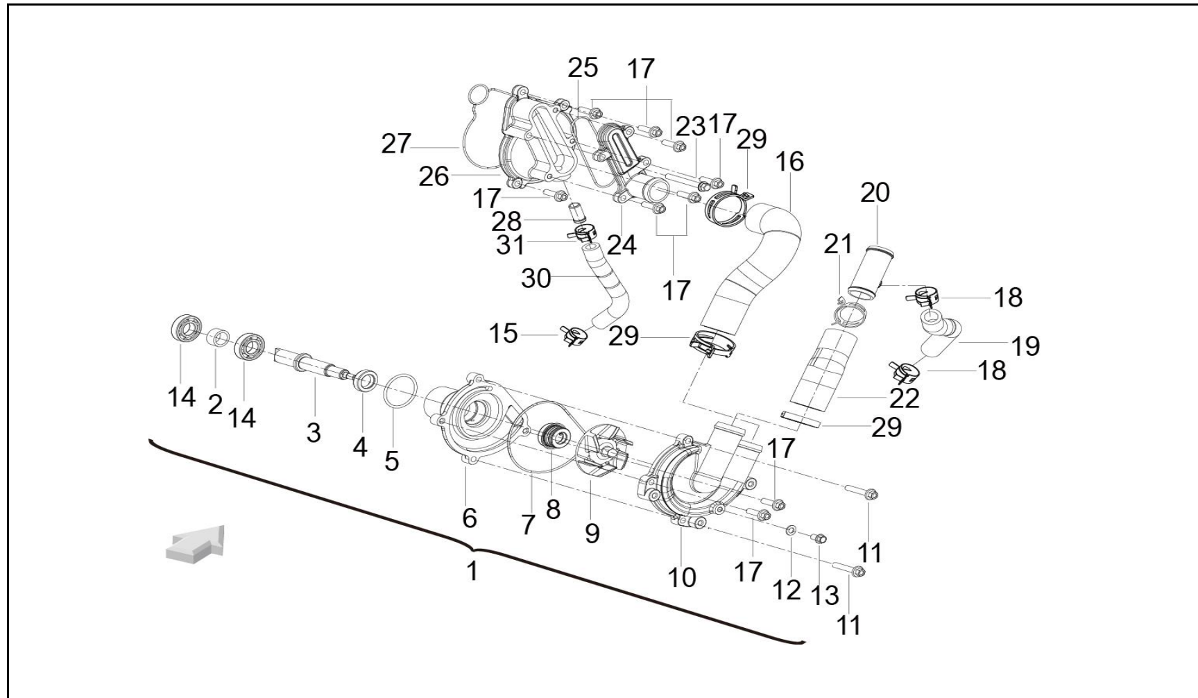
FIGURA N° 14: SISTEMA DE REFRIGERACIÓN
