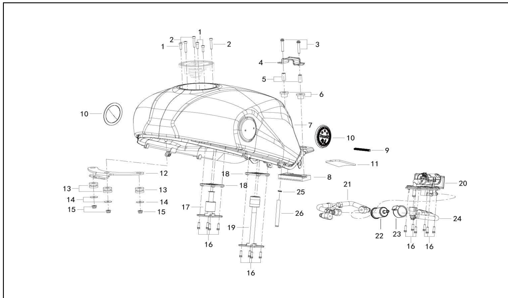
FIGURA N° 22: TANQUE DE COMBUSTIBLE
