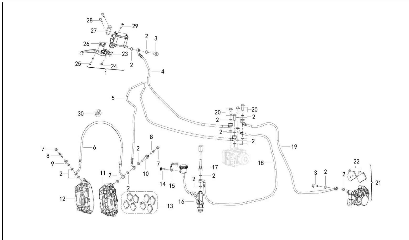
FIGURA N° 19: SISTEMA DE FRENOS
