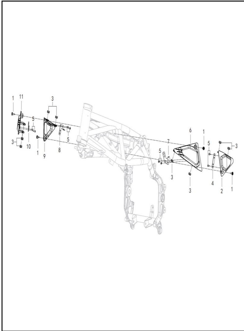
FIGURA N° 25: CUBIERTAS CHASIS
