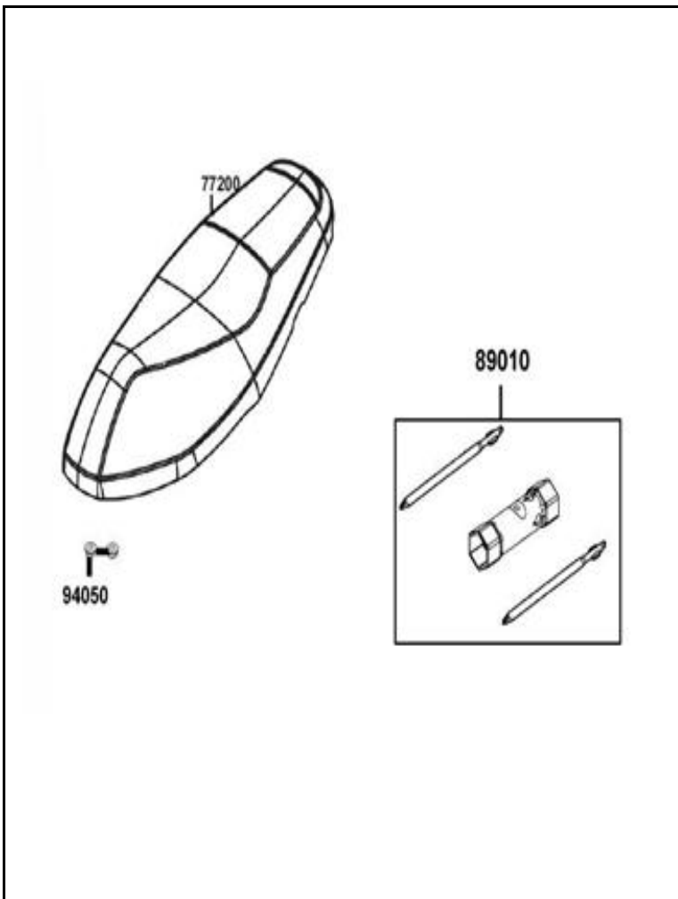
FIGURA N° 18: SILLIN
