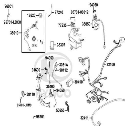
FIG. N° 28 SISTEMA ELECTRICO
