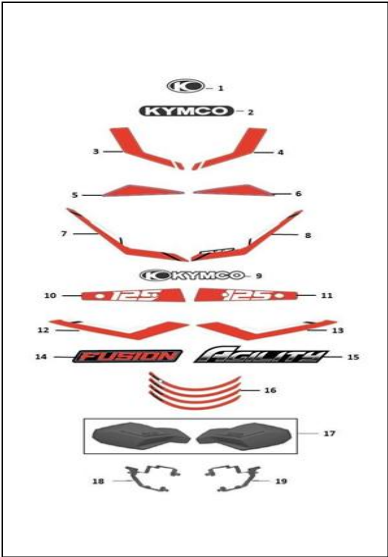
FIGURA N° 30: CALCOMANÍAS Y ACCESORIOS 2/2
