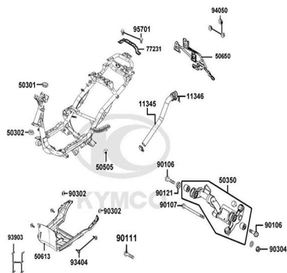
FIG. N° 29 CHASIS
