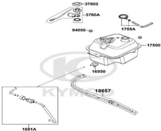
FIG. N° 19 TANQUE DE COMBUSTIBLE
