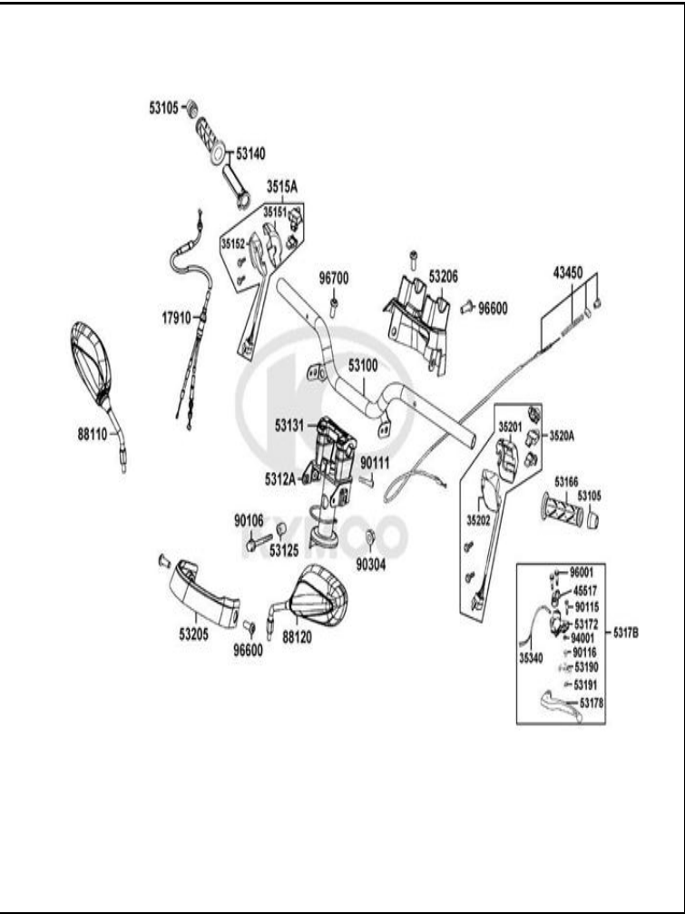
FIGURA N° 12: MANUBRIO - CUBIERTAS MANUBRIO 1/2
