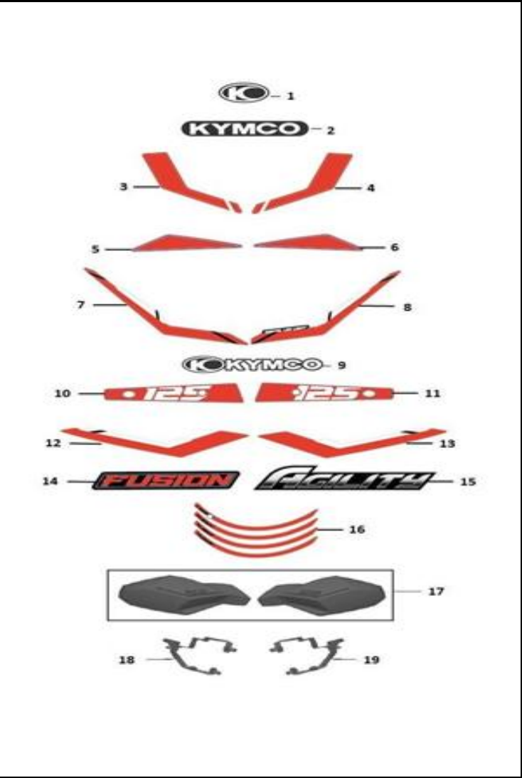
FIGURA N° 30: CALCOMANÍAS Y ACCESORIOS 1/2
