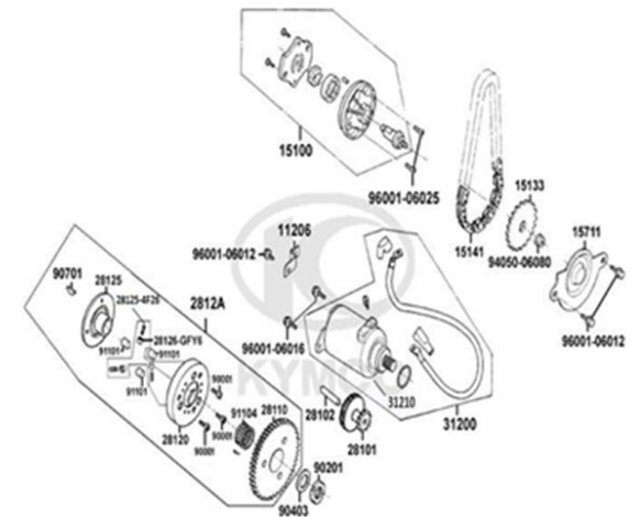
FIG. N° 6 MOTOR DE ARRANQUE - BOMBA DE ACEITE
