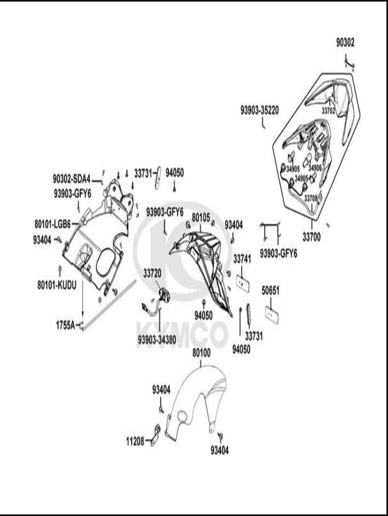
FIGURA N° 27: GUARDABARRO TARSERO
