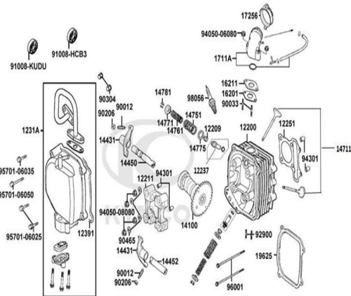
FIG. N° 2 CULATA
