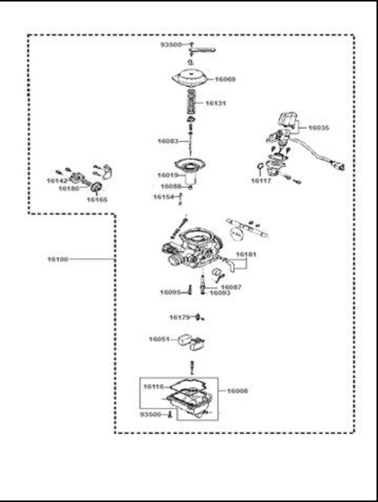
FIGURA N° 9: CARBURADOR
