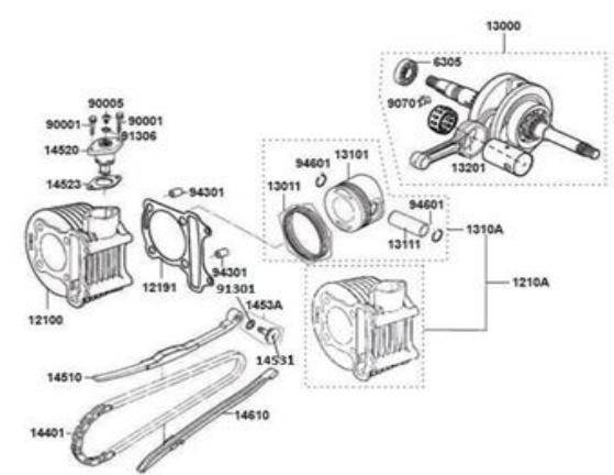
FIG. N° 3 CILINDRO - PISTÓN - CIGÜENAL
