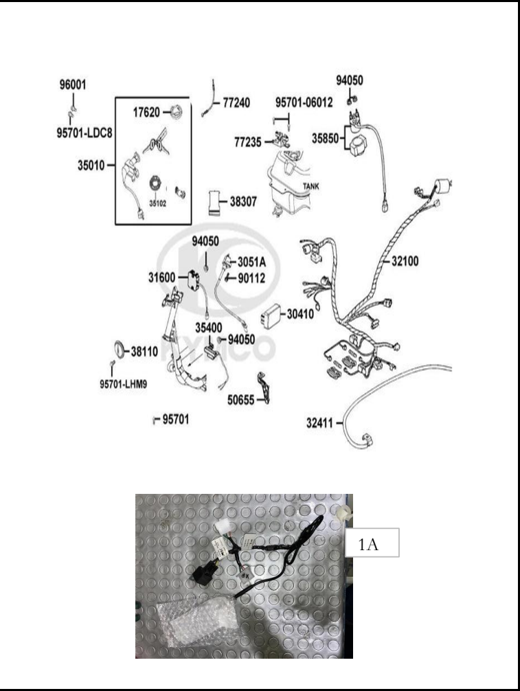
FIGURA N° 28: SISTEMA ELECTRICO
