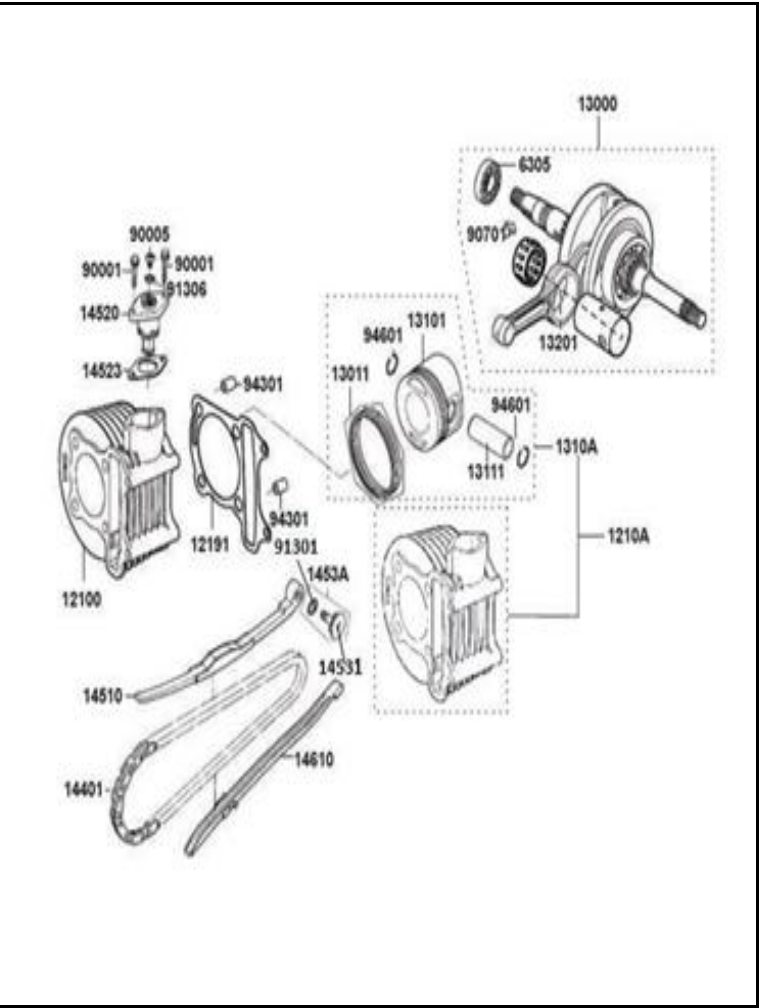
FIGURA N° 3: CILINDRO - PISTÓN - CIGÜEÑAL
