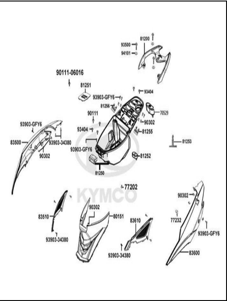
FIGURA N° 21 CUBIERTAS LATERALES - GUANTERA
