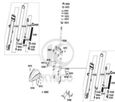
FIG. N° 15 SUSPENSION DELANTERA
