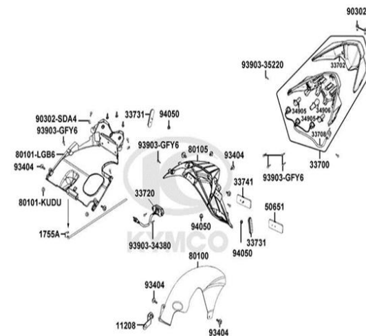
FIG. N° 27 GUARDABARRO TARSERO
