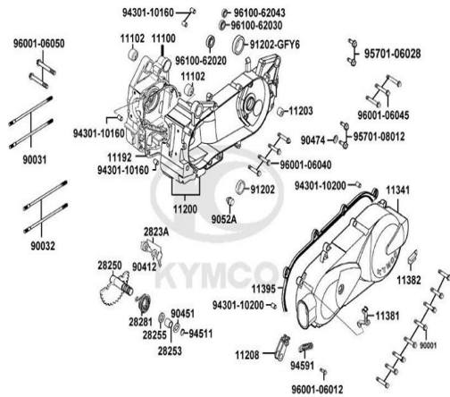
FIG. N° 1 CARCASAS
