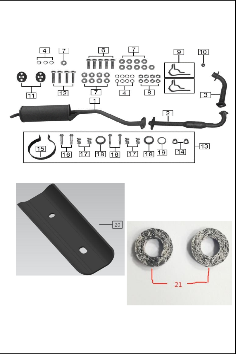
FIGURA N°16 SILENCIADOR
